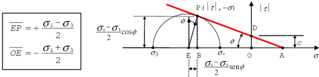
Figura 2.3 - Critério de Mohr-Coulomb.
