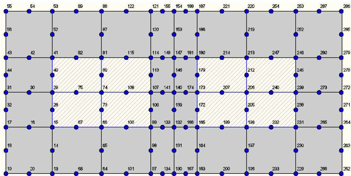
Figura 6.3 - Camada 01 de nós
