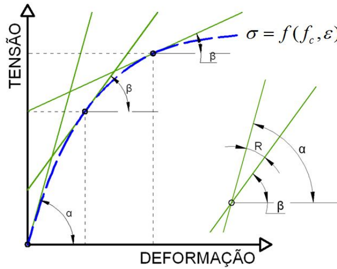
Figura 5.39 - Relação tensão-deformação genérica.
