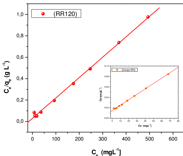
Figura 41 - Linearização da equação de Langmuir das isothermas de adsorção dos corantes RO16 e RR120: pH 4 ( \mu = 0,1 \text{ mol}^{-1} ), 50°C. Fonte: Dados da Pesquisa
