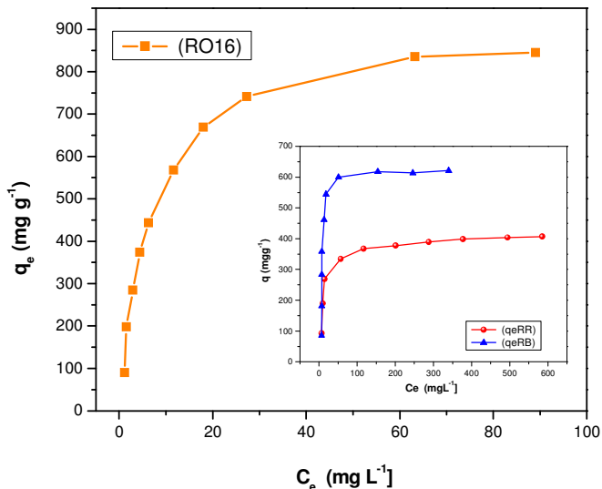
Figura 38 - Isotermas de adsorção dos corantes RO16, RR120 e RB4: pH 4 ( \mu=0,1 mol L -1 ), 25°C. Fonte: Dados da Pesquisa
