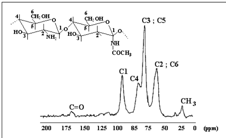
Figura 8 - Espectro de ^{13}\text{C} RMN no estado sólido da quitosana. Fonte: Taboada et al. (2004).
