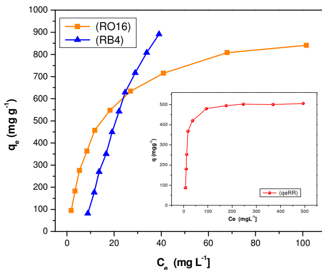
Figura 39 - Isotermas de adsorção dos corantes RO16, RR120 e RB4: pH 4,0 ( \mu=0,1\text{mol L}^{-1} ), 50°C. Fonte: Dados da Pesquisa
