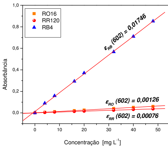
Figura 25 - Curva de calibração dos corantes RO16, RR120 e RB4 lido no \lambda_{max} 602.
