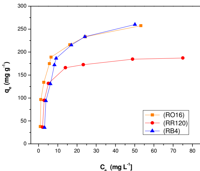
Figura 43 - Isoterma de adsorção dos corantes RO16, RR120 e RB4 em misturas: pH 4 ( \mu=0,1 \text{ mol}^{-1} ), 25°C.
