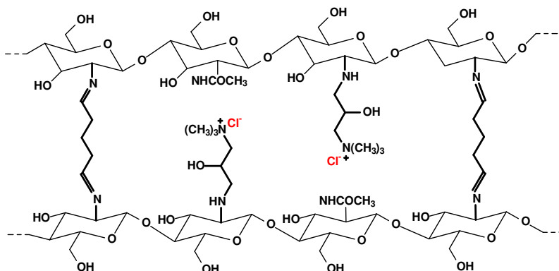
Figura 13 - Estrutura do sal de amônio quaternário de quitosana reticulado.
