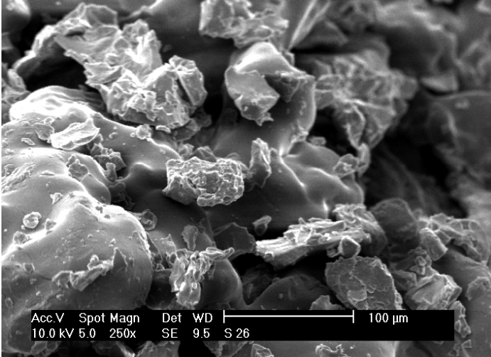
Figura 20 - Microscopia eletrônica de varredura (MEV) do SQQ. Fonte: Dados da Pesquisa
