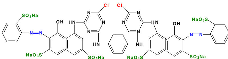
Figura 11 - Estrutura do corante reativo Vermelho 120, diazo, monoclorotriazina.
