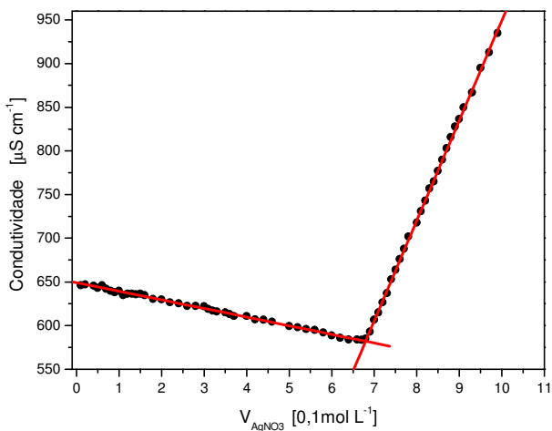
Figura 17 - Titulação condutimétrica do SQQ pelo \text{AgNO}_3 0,1 mol L -1 . Fonte: Dados da Pesquisa
