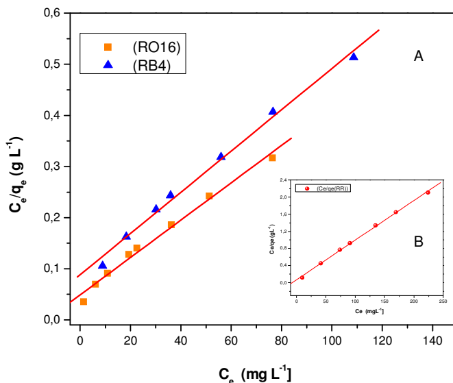
Figura 46 - Linearização da equação de Langmuir das isothermas de adsorção dos corantes RO16, RR120 e RB4 em misturas : pH 12,4 ( \mu = 0,1 \text{ mol L}^{-1} ), 25°C.
