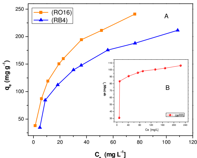
Figura 45 - Isoterma de adsorção dos corantes RO16, RR120 e RB4 em uma solução simulando um efluente têxtil, pH 12,4; 25 °C.
