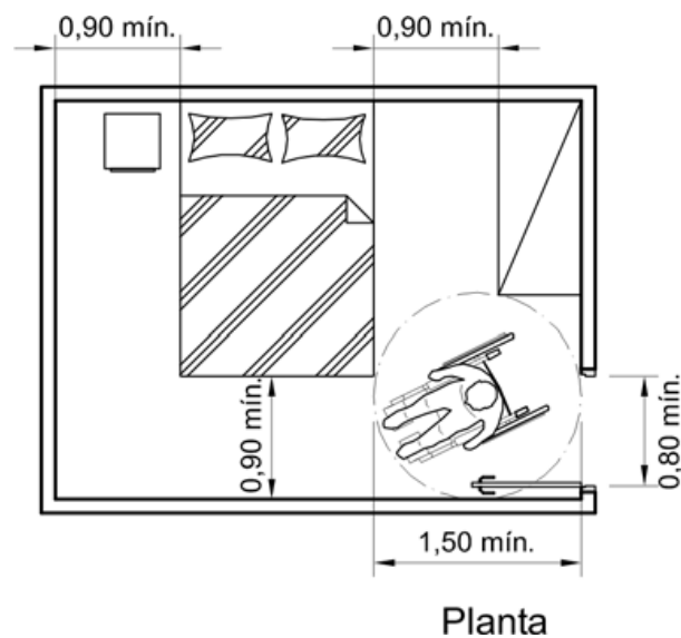
Figura 6: Circulação Mínima em Dormitórios - Exemplo – Fonte 9050:2004
