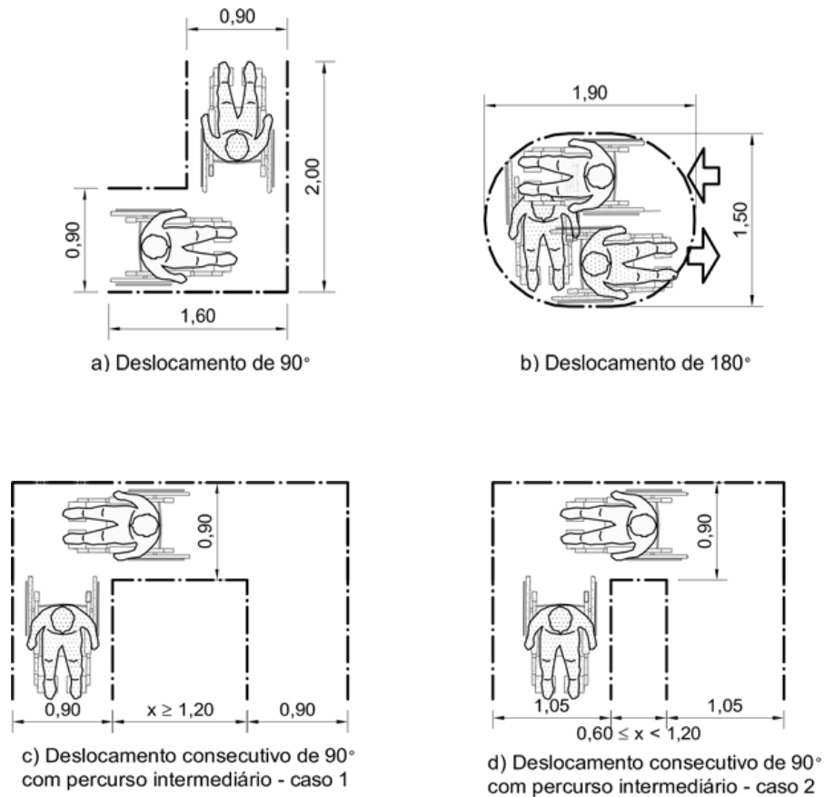
Figura 4: Área para manobra de cadeira de rodas com deslocamento – Fonte: NBR 9050:2004
