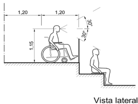
Figura 5: Anteparos em arquibancadas – Vista lateral – Fonte: NBR 9050:2004
