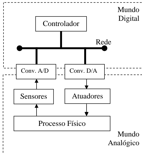
Figura 1.4 – Configuração de blocos digitais e analógicos de uma estrutura de sistemas de controle por rede.
