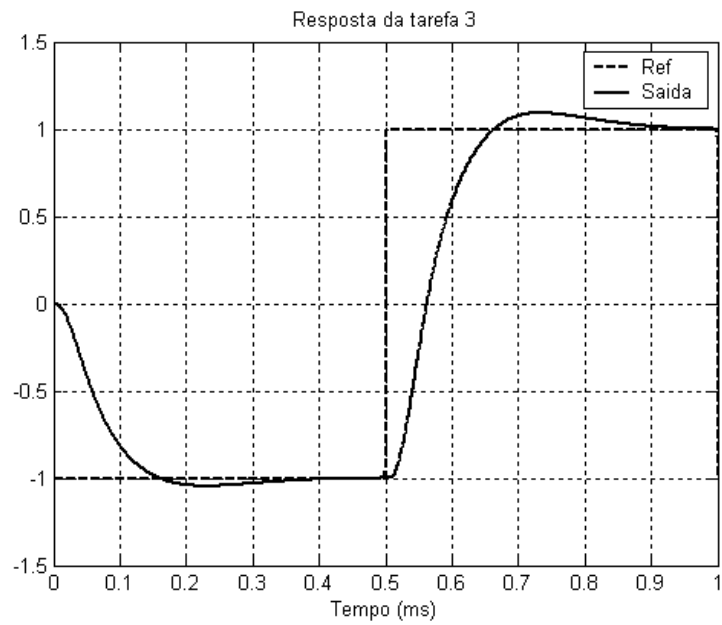
Figura B.5 – Saída da tarefa #3 com taxa monotônica.
