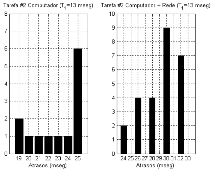
Figura 5.19 – Histograma caso T_1 = 13 ms e T_2 = 50 ms.
