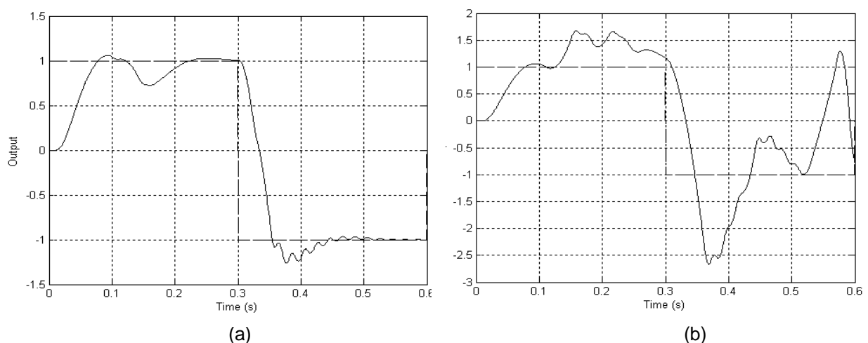
Figura 3.1 – Influência da perda de pacotes sobre a performance do controle.
