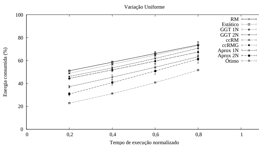
Figura 4.11: Processador teórico de 4 níveis mais espaçados.
