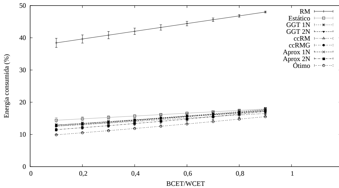
Figura 4.19: CNC.
