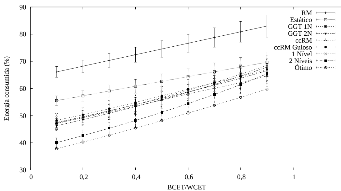
Figura 4.21: Aviônica.
