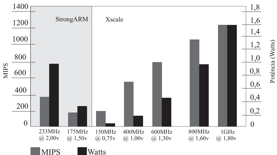
Figura 2.1: Comparação do consumo de energia e do desempenho para as arquiteturas StrongARM e XScale.
