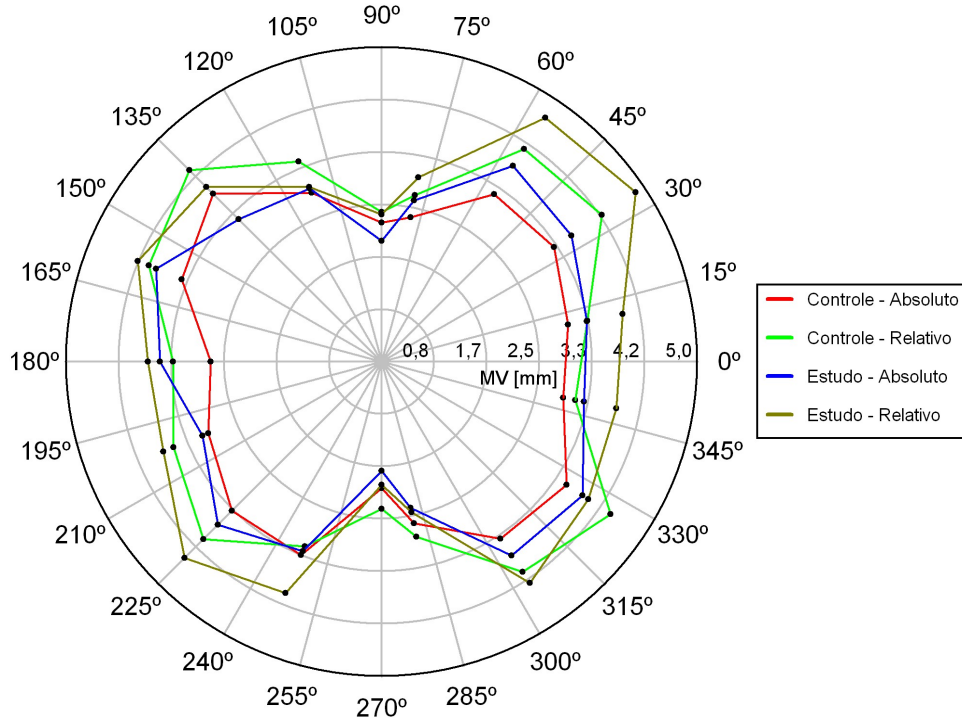
Gráfico 15- Médias entre a 1ª e 12ª tentativa do parâmetro variabilidade no movimento (MV) em função das direções estudadas para o grau de dificuldade 5 bits, segundo os grupos e seus respectivos modos de controle.
