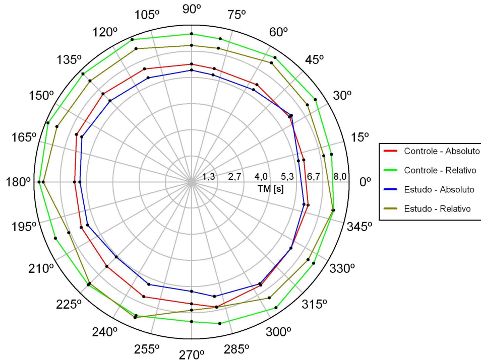
Gráfico 13- Médias entre a 1ª e 12ª tentativa do parâmetro tempo de movimento (TM) em função das direções estudadas para o grau de dificuldade 5 bits, segundo os grupos e seus respectivos modos de controle.
