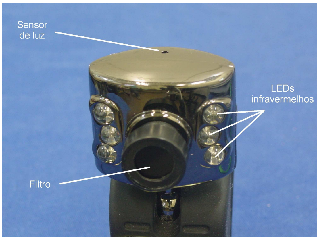
Figura 2- Detalhe da câmera tipo "webcam" com seis LEDs infravermelhos, sensor de luz e filtro.
