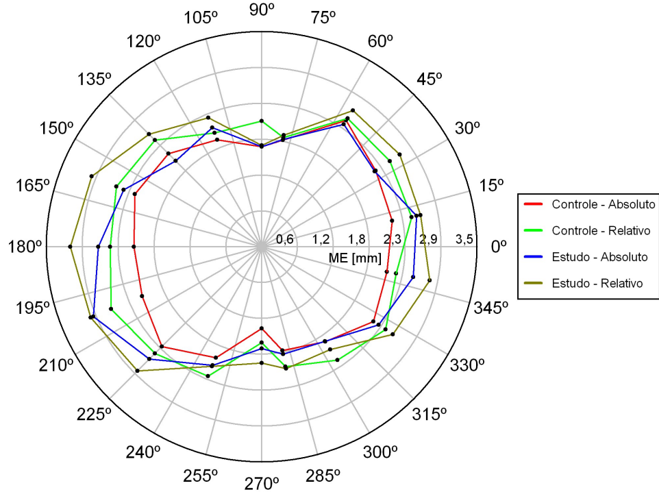
Gráfico 16- Médias entre a 1ª e 12ª tentativa do parâmetro erro no movimento (ME) em função das direções estudadas para o grau de dificuldade 2 bits, segundo os grupos e seus respectivos modos de controle.
