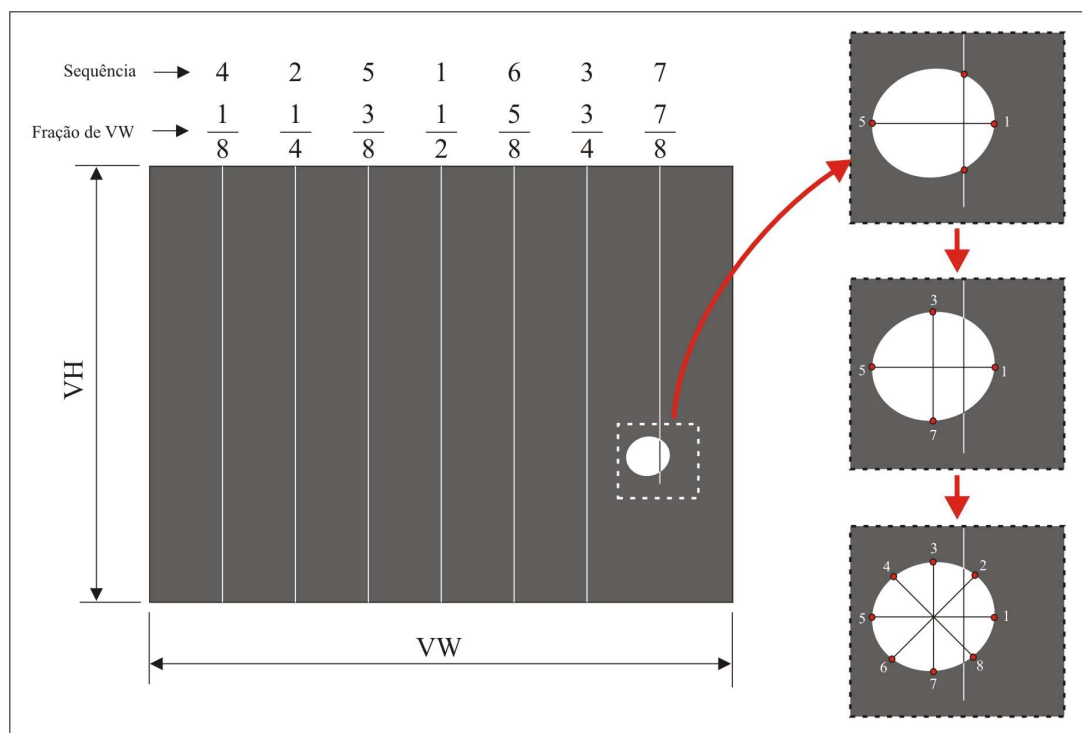
Figura 4- Esquema hipotético da descrição da seqüência e posição da coluna de rastreo para a determinação do centro do alvo na imagem da câmera. Onde “VH” e “VW” representam a altura e a largura da imagem. Detalhe (à direita) do método de identificação dos oito pontos do possível objeto.
