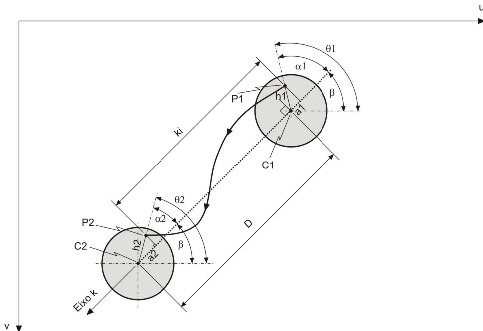
Figura 21- Representação do método para determinação da projeção ( k_i ) dos pontos de parada dentro dos objetos alinhados ao eixo k . As coordenadas de todos os pontos foram medidas em relação ao eixo u-v da tela do monitor.
