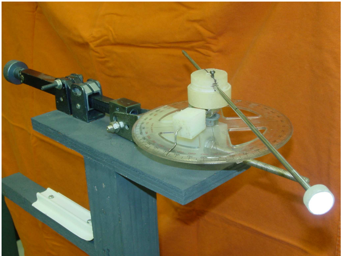
Figura 10- Dispositivo utilizado para simular o movimento de rotação da cabeça.
