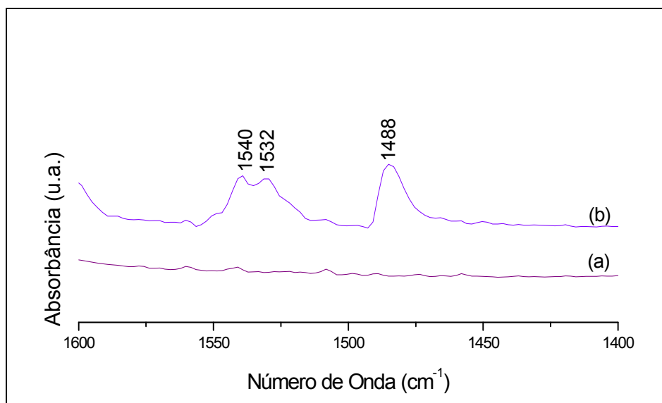
Figura 3.3 - FTIR de 20HPW/ \text{ZrO}_2 antes (a) e depois de adsorção com Py (b).
