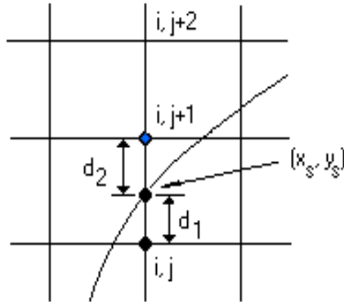
Figura 3.8: Transferência de informações de cada ponto do contorno imerso com dois nós adjacentes da malha.
