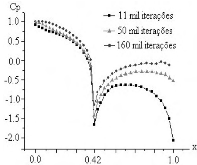
Figura 4.5: Comparação dos coeficientes de pressão para a Eq. de Navier Stokes segundo o número de iterações.
