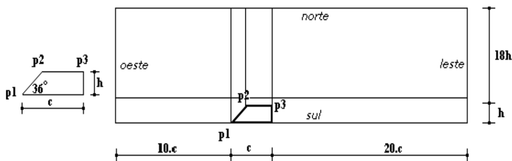
Figura 4.1: Dimensões da geometria simplificada e indicação das regiões no domínio.
