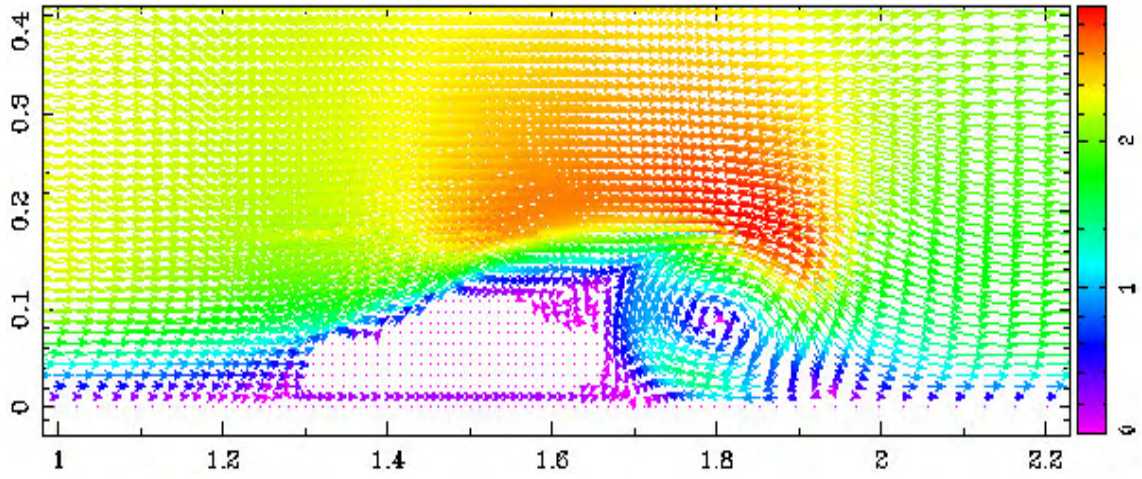
Figura 4.16: Campo de velocidades sobre o automóvel.
