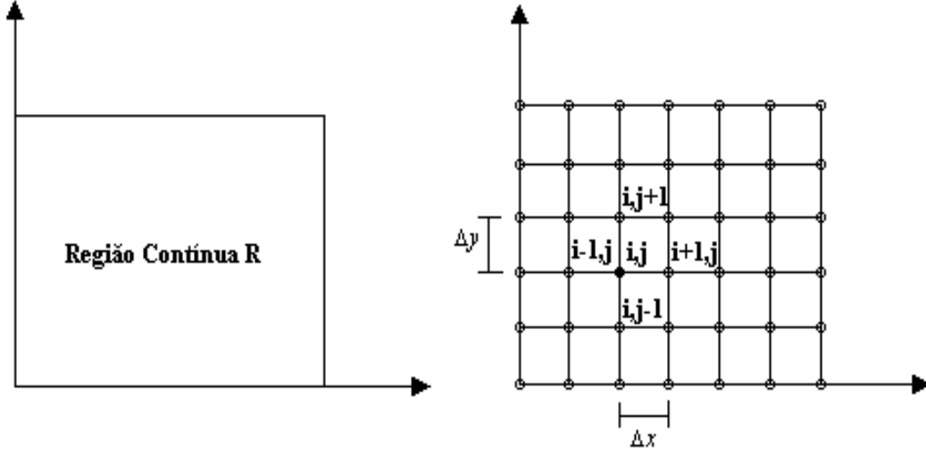
Figura 3.3: Regiões contínua e discretizada
