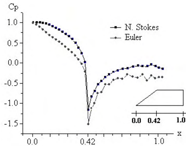
Figura 4.8: Comparação entre os coeficientes de pressão para geometria simplificada.
