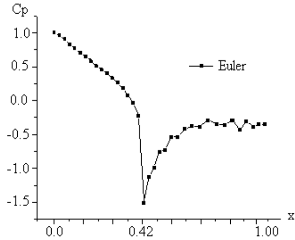
Figura 4.7: Coeficiente de pressão utilizando as equações de Euler.
