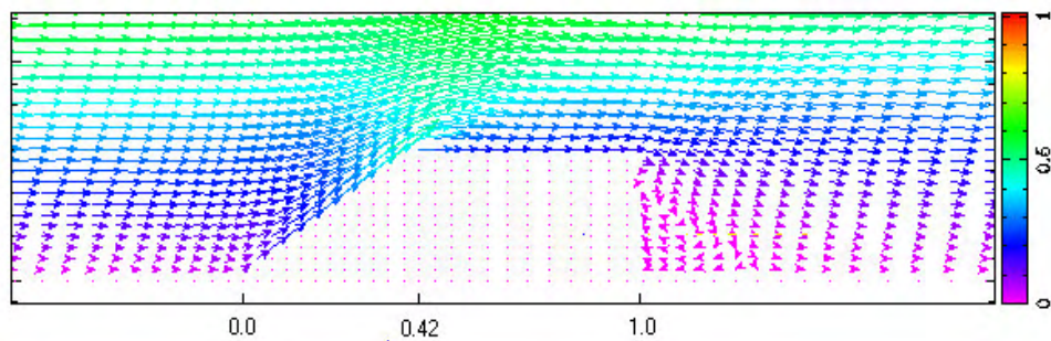
Figura 4.6: Campo de velocidades sobre a geometria simplificada através da equação de Navier-Stokes.
