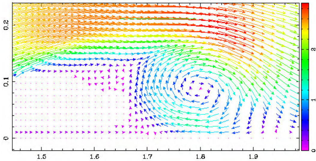
Figura 4.17: Ampliação do campo de velocidades da figura 4.16.
