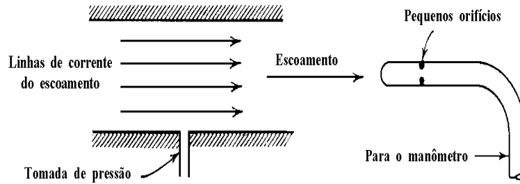
Figura 4.18: Medição da pressão estática.
