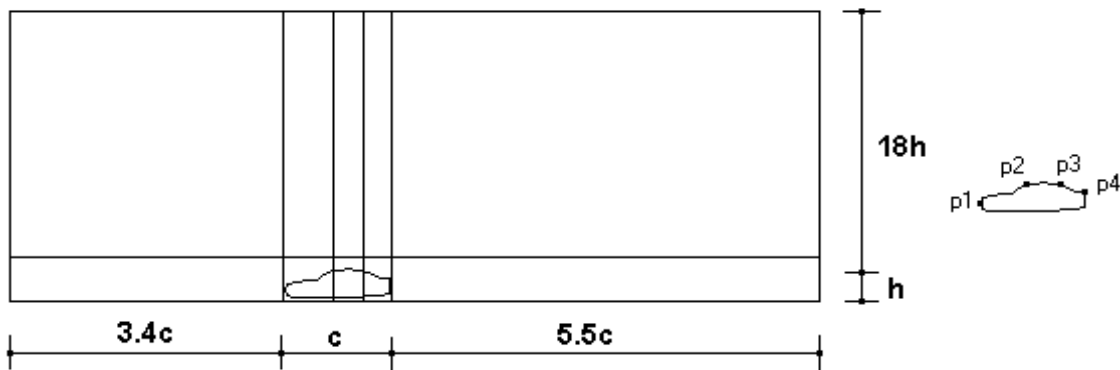
Figura 4.9: Dimensões do automóvel em relação à malha computacional.
