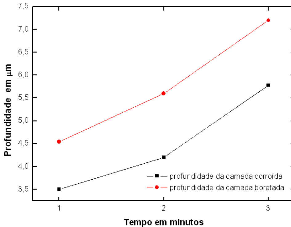
Figura 4.21 - Variação da profundidade da camada corroída com a profundidade da camada boreta versus o tempo de corrosão.
