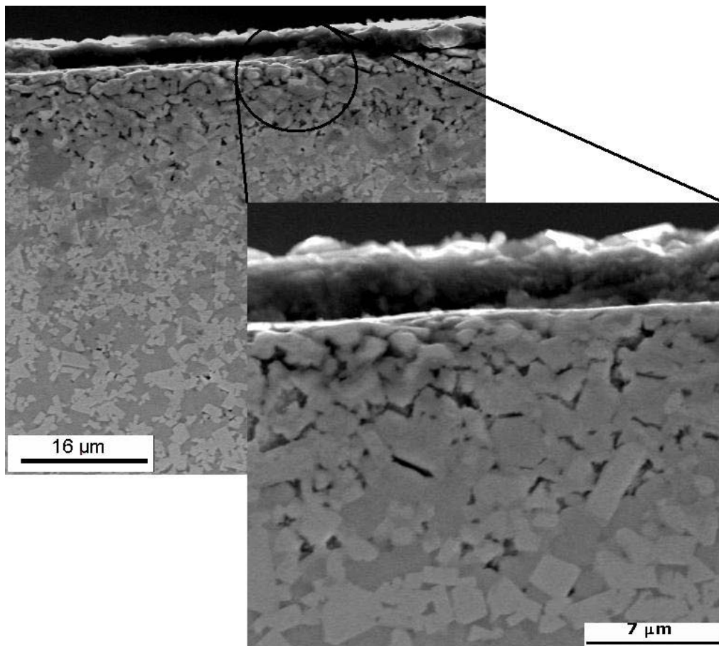
Figura 4.28 - Interface da amostra de WC-Co com TiC que foi boretada com 15\%B_4C + 10\%KBF_4 + 5\%C + 70\%SiC na temperatura de 1000^{\circ}C por 5h ; corroída com H_2SO_4 + H_2O_2 (2:8) por 1 minuto e em seguida crescimento de diamante por 5h.
