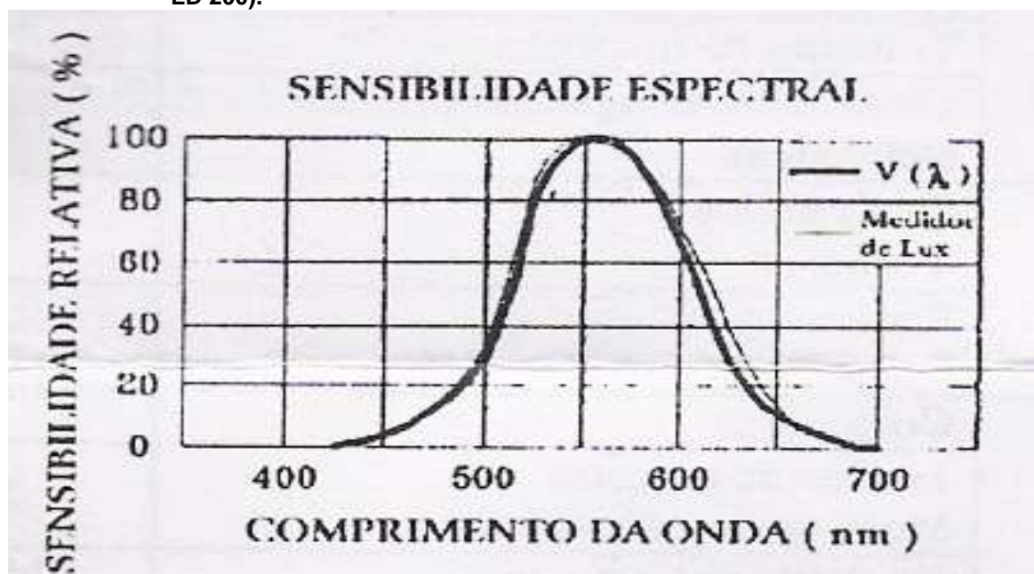
Apêndice G - Sensibilidade espectral, nos diferentes comprimentos de onda (Luxímetro LD 200).
