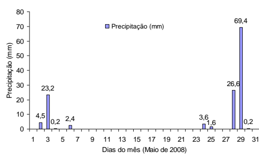
Figura 6 – Temperaturas mínimas, médias e máximas (° C) (a) e total de precipitação diária (mm) durante o mês de Maio de 2008. Santa Maria/RS (b).
