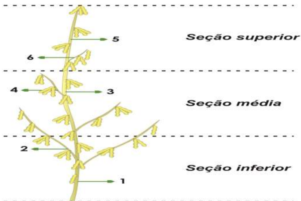
Figura 1 - Esquema de divisão das plantas de soja em seis estratos (1: haste principal inferior, 2: ramos inferiores, 3: haste principal média, 4: ramos médios, 5: haste principal superior e 6: ramos superiores) por dois planos paralelos ao solo, em relação à estatura da planta.
