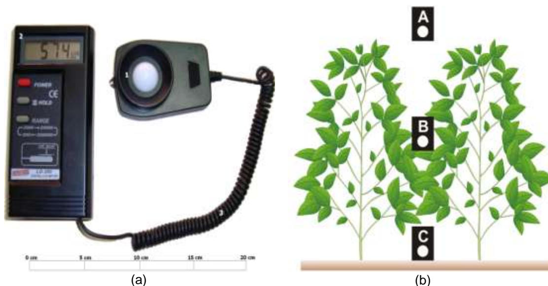
Figura 1 - Luxímetro digital utilizado para as avaliações da quantidade de luz incidente no dossel (1: fotocélula, 2: display digital de registro e 3: interface flexível) (a). Níveis do dossel em que as leituras foram efetuadas, onde “A” significa nível superior, “B” nível médio e “C” em nível do solo (b).
