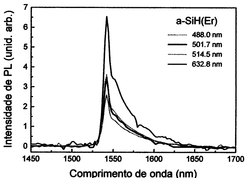
Figura 4 — Espectros de PL de um filme de a-Si:H dopado com Er (Si# 151), obtidos a 12 K segundo fótons com diferentes comprimentos de onda. O sinal refere-se à transição entre os níveis ^4I_{13/2} e ^4I_{15/2} do íon terra-rara Er^{3+} . Exceto por pequenas variações na intensidade total do sinal (todos obtidos com \sim 10 mW), o formato de linha da transição permanece inalterado.
