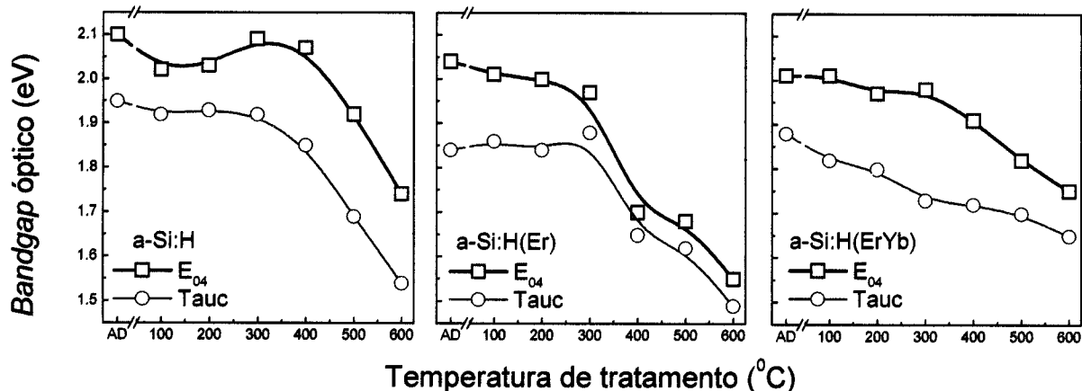
Figura 2 – E_{04} e E_{T_{auc}} ( bandgap óptico) de filmes de a-Si:H não dopado e dopado com Er e Er+Yb , para diferentes temperaturas de tratamento térmico. Independentemente do método adotado para definir o bandgap óptico, verifica-se o mesmo tipo de comportamento para todas as amostras. Note a redução nos valores de E_{04} e E_{T_{auc}} à medida que os tratamentos são feitos a maiores temperaturas.
