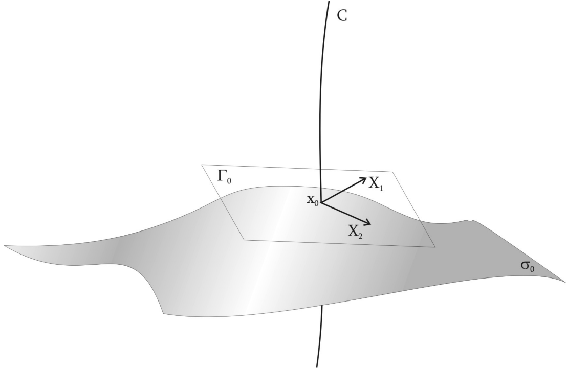
Figura 2.2: A trajetória C , uma superfície \sigma_0 e o respectivo plano tangente \Gamma_0 . O vetor tangente a C é ortogonal aos vetores de base que geram a distribuição. A condição de integrabilidade é satisfeita se a figura for estendida a toda família \sigma e a toda congruência de curvas K , do qual C é membro.
