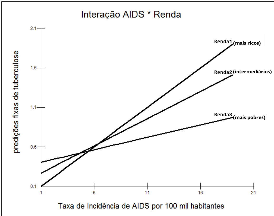
Figura 4 - Interação entre taxa de AIDS e proporção de domicílios com renda de até 2 salários mínimos, e associação com as predições fixas de tuberculose, Brasil 2001 – 2003.
