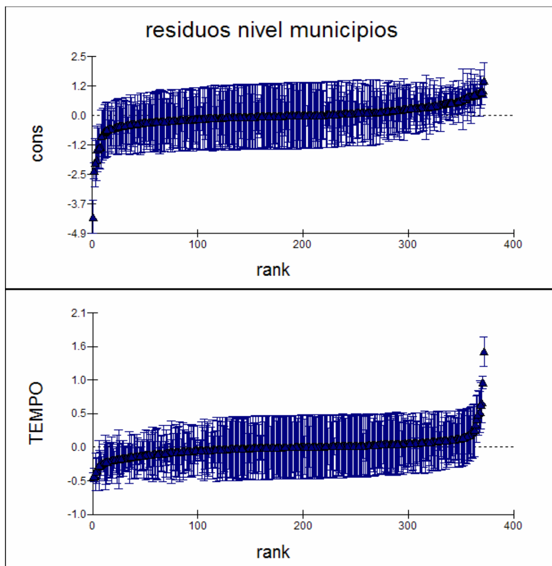
Figura 14 – Erro padrão dos resíduos versus ranque (nível municípios)
