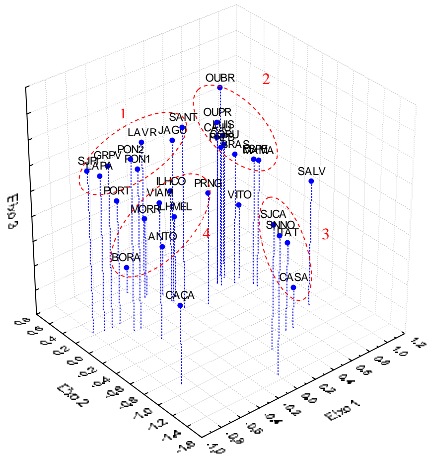
Figura 10. Gráfico de ordenação dos 32 estudos comparados por CA, considerando os eixos um, dois e três com autovalores 0,25; 0,17; 0,06 respectivamente. Elipses adicionadas arbitrariamente.
