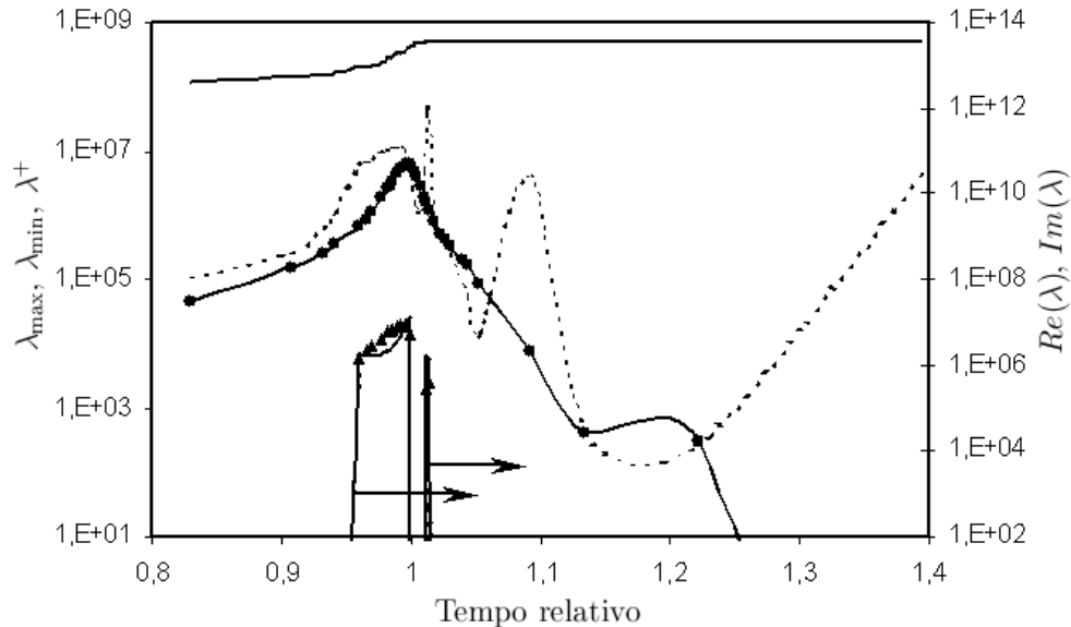
Figura 6.17: Evolução dos autovalores principais \lambda_{\max}(-) ; \lambda_{\min}(\cdots) ; \lambda^+(\bullet-) ; |Re(\lambda_c)|(-) ; |Im(\lambda_c)|(\blacktriangle \cdots) para o regime P = 10atm , k_m = 16 , meio “ H_2 + O_2 ”.
