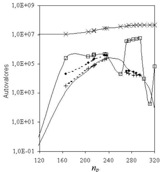
Figura 6.13: Evolução dos autovalores: \lambda_{\max} ( \times ); \lambda_{\min} ( \square ); \lambda^+ ( - ); Re(\lambda_c) ( -+ ); Im(\lambda_c) ( - \bullet ) em função de n_p , para as etapas S1 , S2
