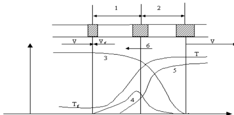
Figura 2.3: Frente de chama premista
