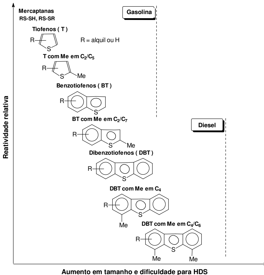
Figura 2. Reatividade de compostos orgânicos de enxofre em processos de HDS relacionada com seus tamanhos de anel e a posição dos substituintes (adaptado de Song 90 ).
