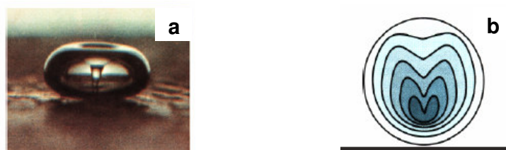
Figura 7. Micrografia da (a) implosão de uma bolha de cavitação próxima a uma superfície sólida e (b) evolução da cavidade formando o jato (adaptado de Suslick 98 ).
