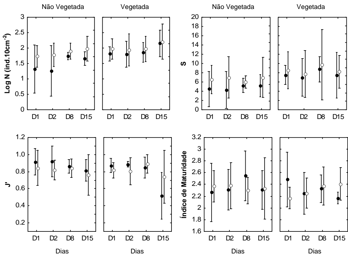
Figura 13. Densidade (N) de indivíduos de Nematoda, número de gêneros (S), Equitatividade de Pielou (J) e índice de maturidade (média \pm erro padrão) no tratamento de arrasto (●) e no controle (○) realizados em áreas vegetadas e não vegetadas, ao longo de 15 dias.
