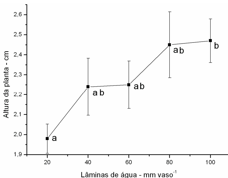
Gráfico 4.16. Valores médios da altura de planta (AP) do Algarrobeira, quando submetido ao fator lâminas de água (W) aos 180 DAT. Barras representam o valor médio e as linhas verticais, o erro-padrão de estimativa da média de cada tratamento.
