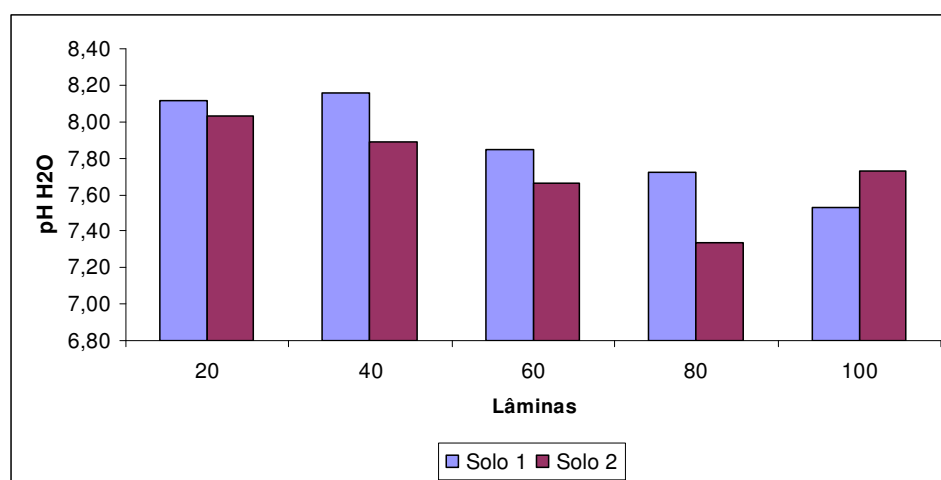
Gráfico 4.27. Valores de pH no final do experimento para os dois tipos de solo.
