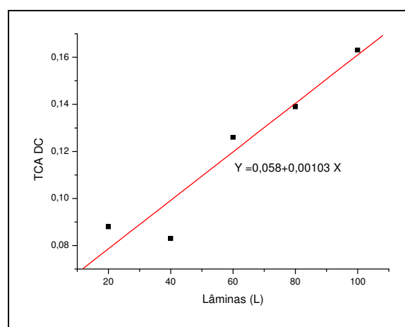
Gráfico 4.25. Taxa de crescimento absoluto de diâmetro caulinar aos 90 dias após transplântio. (coeficiente de determinação R^2=0,9139 )
