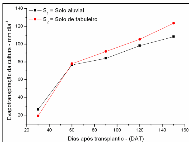
Gráfico 4.13. Variação da evapotranspiração da algarobeira, 30, 60, 90, 120 e 150 dias após transplante (DAT), quando aos tipos de solo, no período de janeiro a Junho de 2008, em Campina Grande/PB.
