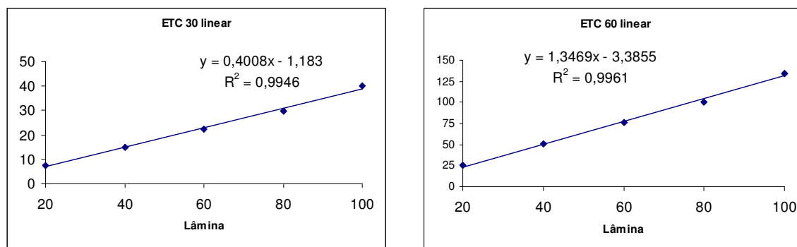
Gráfico 4.14a. Evapotranspiração da cultura (ETc) da algaroba, aos 30 e 60, dias após transplante (DAT), em função do nível de reposição de água.
