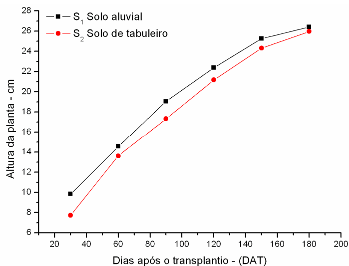
Gráfico 4.19. Valores médios da altura da planta durante o total 180 DAT durante o total 180 DAT da planta Algarobeira, submetido ao fator tipo de solo.
