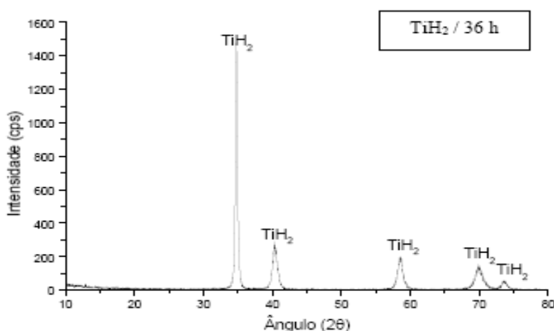
Figura 15 – Difratograma de raios X dos pós de TiH_2 , moídos por 36h (SANTOS, 2006).
