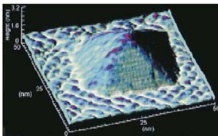
Figura 9 - Em crescimento por epitaxia por feixes moleculares, átomos de germânio auto-organizaram espontaneamente sobre uma base de silício para formar uma nanopirâmide (CHAVES, 2002).
