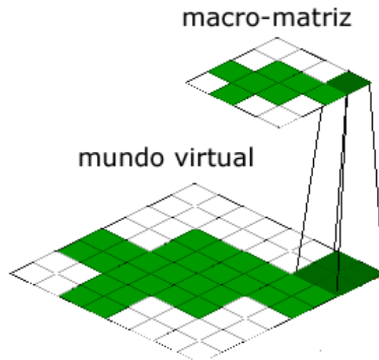
Figura 3.2: Mapeamento da MM para o mundo virtual: cada vértice da MM é mapeado para diversos vértices no mundo virtual.
