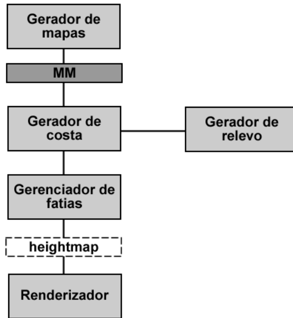
Figura 3.1: Estrutura básica para geração de conteúdo
