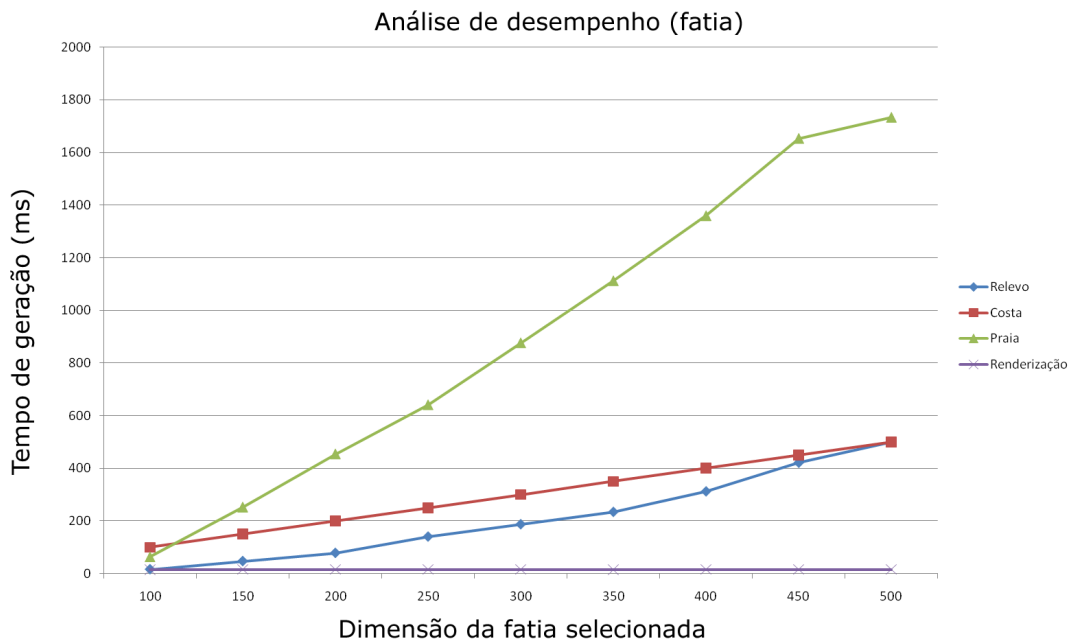
Figura 5.14: Tempo de processamento dos algoritmos envolvidos na geração de uma fatia do mundo virtual (em função do tamanho da fatia).
