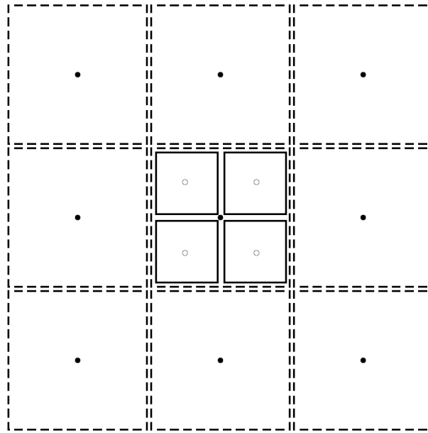
Figura 2.19: Quadtree utilizada para a geração do terreno (DOLLINS, 2002)
