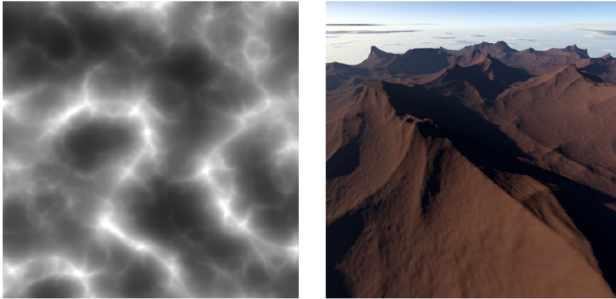
Figura 2.9: À esquerda, heightmap gerado a partir da técnica de ruído de Perlin ridged ; à direita, o mesmo heightmap renderizado em 3D (HäGGSTRÖM, 2006)
