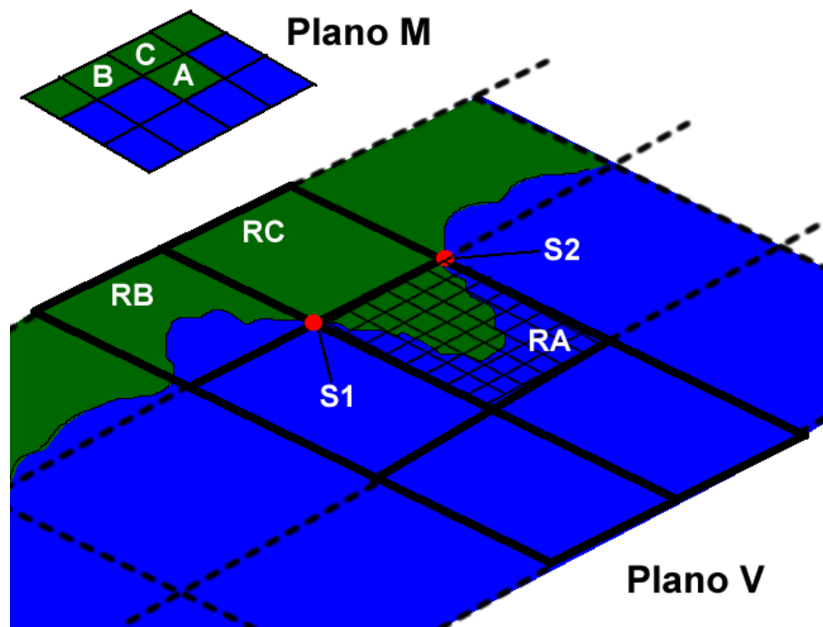
Figura 4.11: Funcionamento do algoritmo de quebra de linearidade da costa
