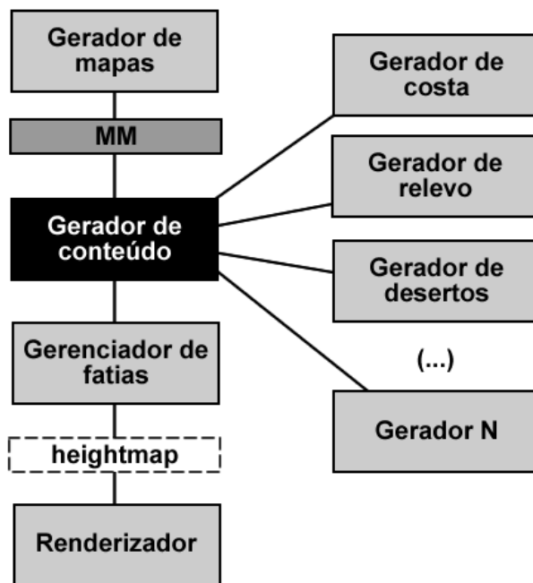
Figura 6.1: Alteração na estrutura atual para permitir uma maior flexibilidade na geração de conteúdos para diferentes tipos de terreno.
