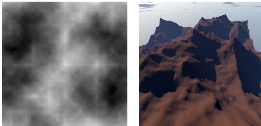
Figura 2.4: À esquerda, heightmap gerado a partir de divisões estocásticas; à direita, o mesmo heightmap renderizado em 3D (DOLLINS, 2002)
