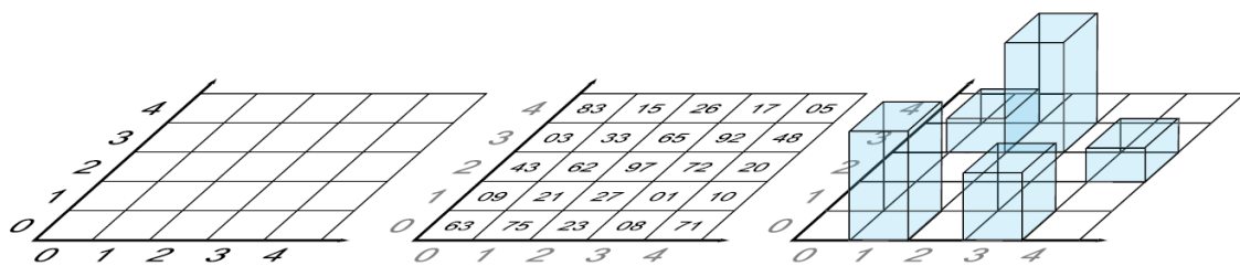
Figura 2.10: Mundo virtual dividido em células. Cada uma delas possui uma semente calculada com base em sua posição e com base uma semente global referente à cidade (GREUTER et al., 2005)
