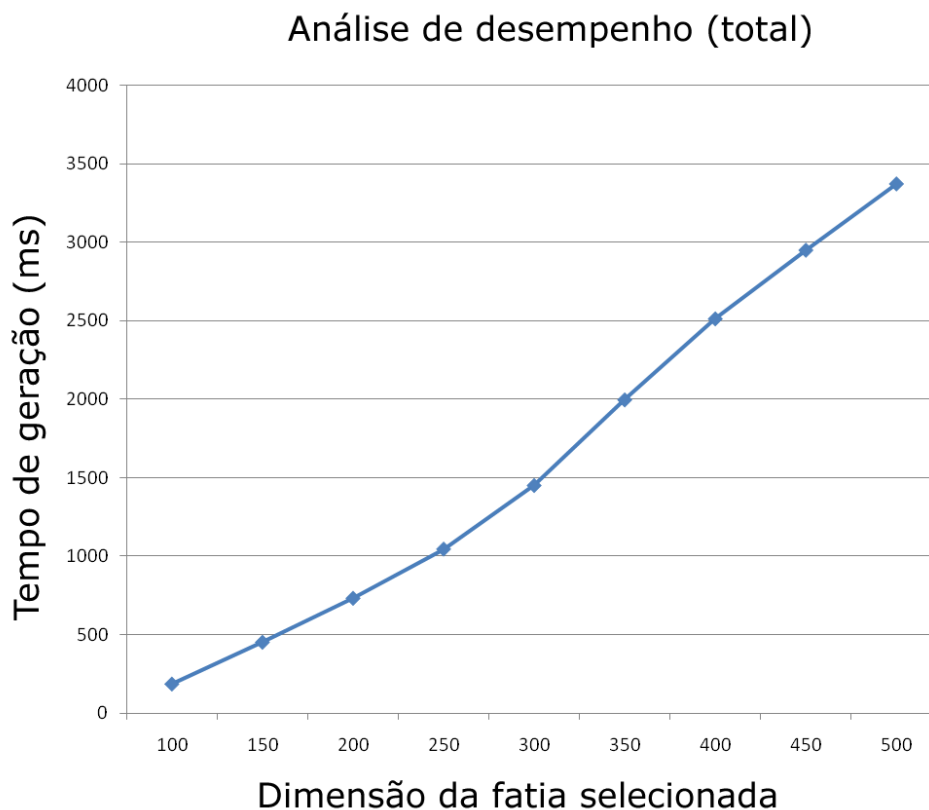
Figura 5.15: Tempo total de processamento dos algoritmos para geração de uma fatia do mundo virtual (em função do tamanho da fatia).
