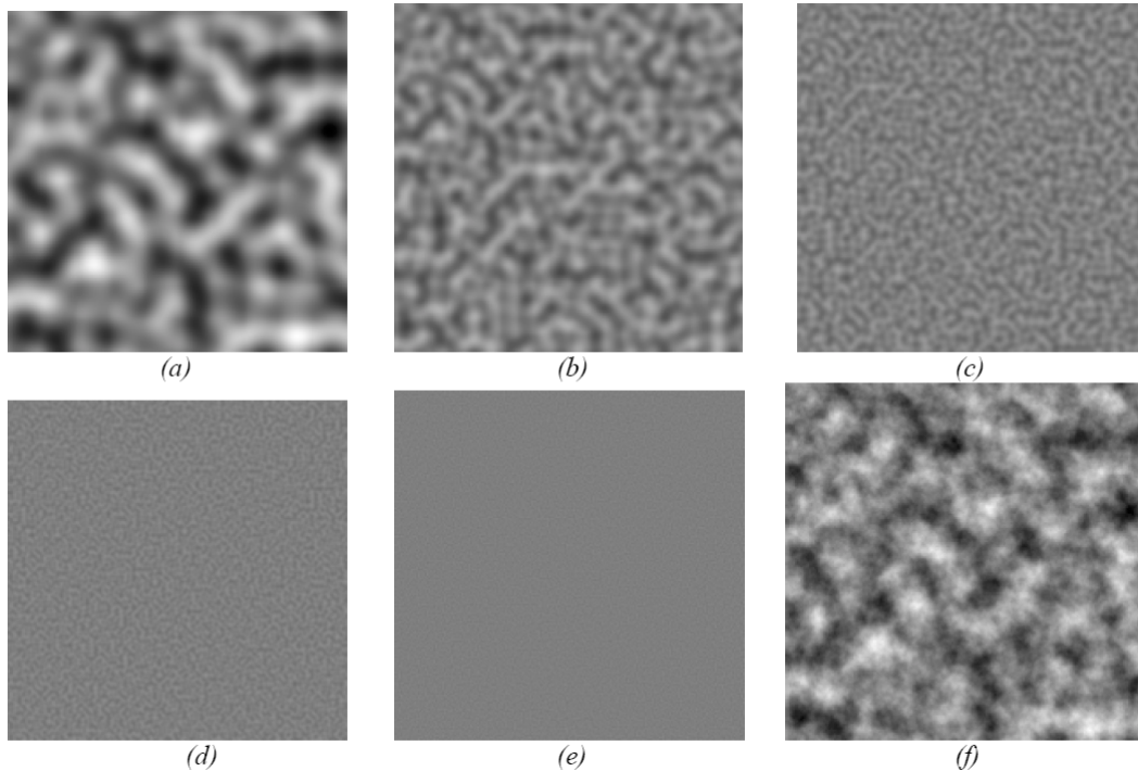
Figura 2.3: Desenho em 2D dos pontos gerados por uma função de ruído de Perlin (ELIAS, 2009)
