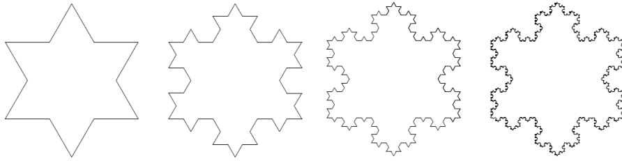
Figura 2.1: Quatro primeiras iterações do fractal de floco-de-neve de Koch (DOLLINS, 2002)
