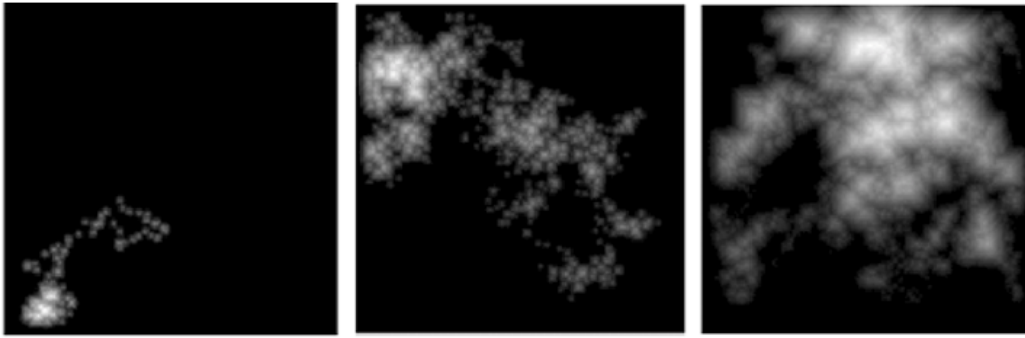
Figura 2.6: Heightmaps obtidos com o algoritmo de deposição de sedimentos. (RIBBLE, 2001)
