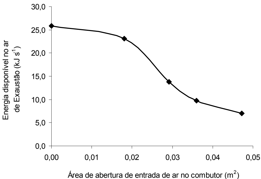
Figura 28: Valores máximos de energia disponível no ar de exaustão, em função das aberturas de entrada de ar no combustor.
