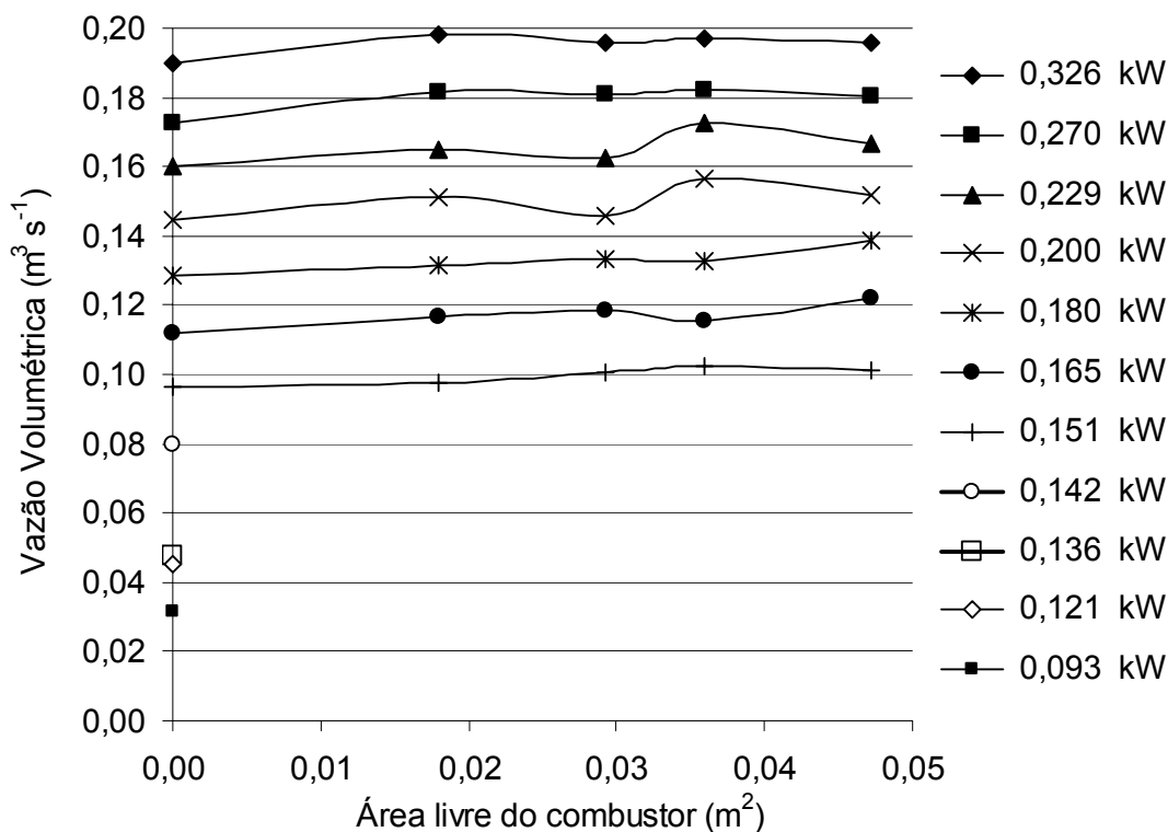
Figura 29: Vazão volumétrica de ar de exaustão em função das áreas de aberturas de entrada de ar no combustor, para diferentes valores de potência ativa média do motor.
