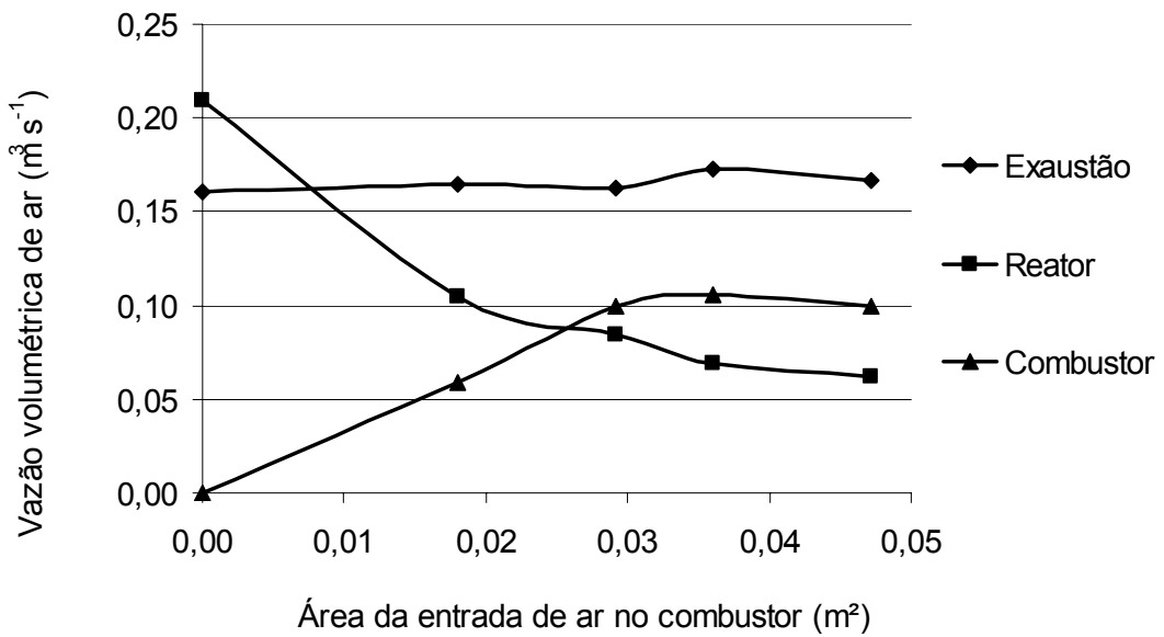
Figura 25: Vazão volumétrica de ar ( \text{m}^3 \text{s}^{-1} ) nas entradas de ar (reator e combustor) e exaustão, para a potência ativa média de 229 W, em função da área de entrada de ar no combustor, durante o processo de gaseificação.
