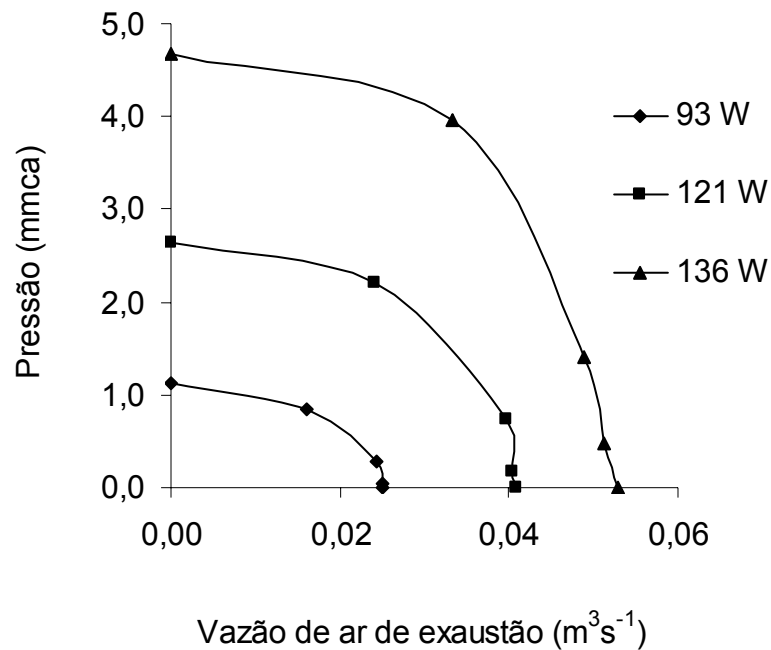
Figura 18: Curva do ventilador (pressão versus vazão volumétrica) para as potências ativa média 93, 121 e 136 W.
