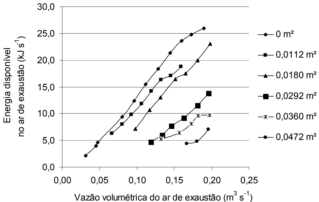
Figura 27: Energia disponível no ar de exaustão por unidade de tempo ( \text{kJ s}^{-1} ) em função da vazão volumétrica, para diferentes valores de área de abertura no combustor.
