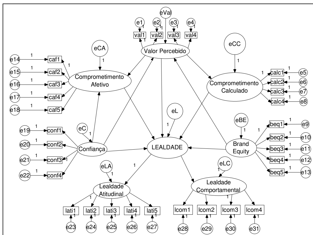
Figura 5 – Modelo Híbrido
