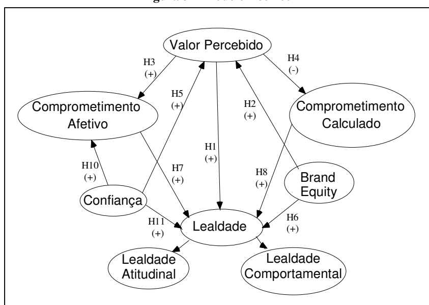
Figura 3 – Modelo Teórico
