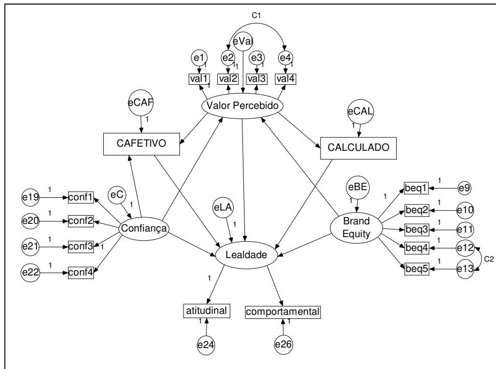
Figura 14 – Modelo Agregado
