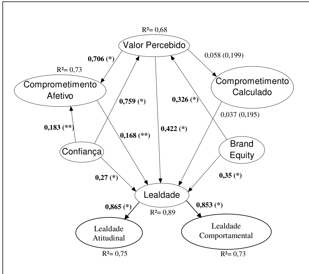
Figura 15 – Modelo estimado
