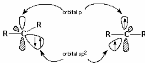
Figura 10 - Ilustração dos estados singleto e tripleto de um carbeno.
