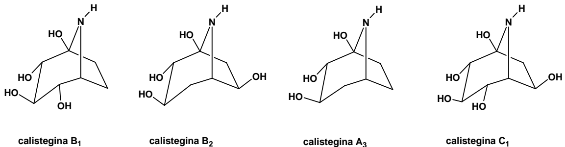
Figura 2 - Tipos de calisteginas (Dräger, 2002).
