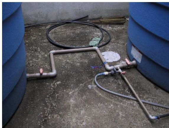
Figura 14 – Tubulação de saída da água armazenada para uso e reabastecimento da cisterna enterrada
