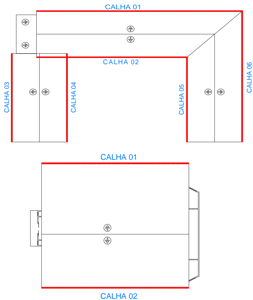
Figura 42 – Localização em planta, das calhas
