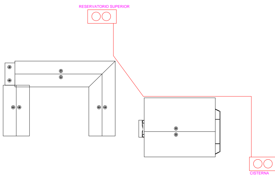
Figura 47 – Localização em planta do reservatório inferior, cisterna e do reservatório superior
