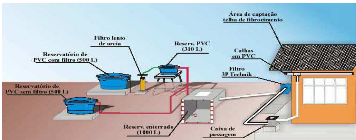
Figura 5 – Esquema do sistema de aproveitamento de água da chuva
