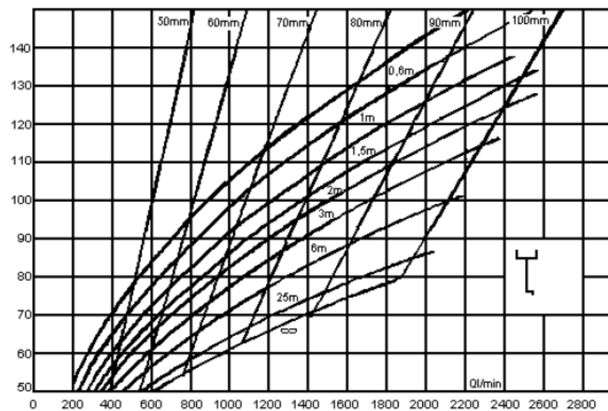
Figura 25 – Calha com saída em aresta viva
