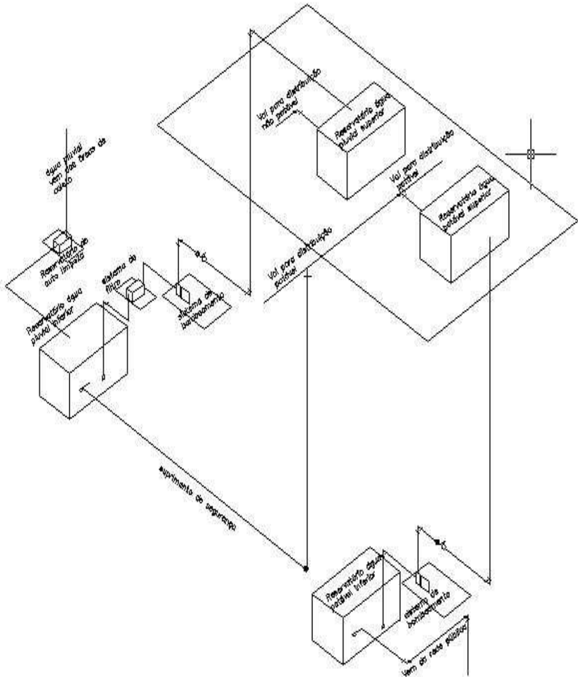
Figura 29 – Sistema de interligação de reservatórios
