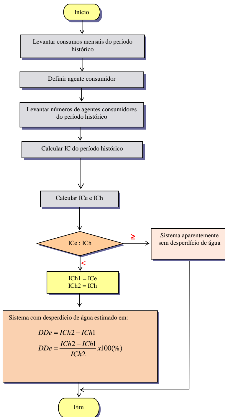
Figura 24 – Fluxograma para a realização do diagnóstico preliminar do consumo de água em um edifício escolar
