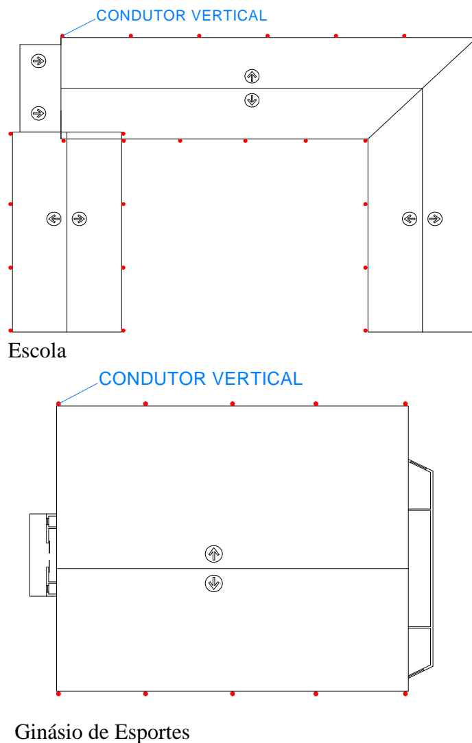
Figura 43 – Localização dos condutores nas calhas da Escola e do Ginásio de Esportes
