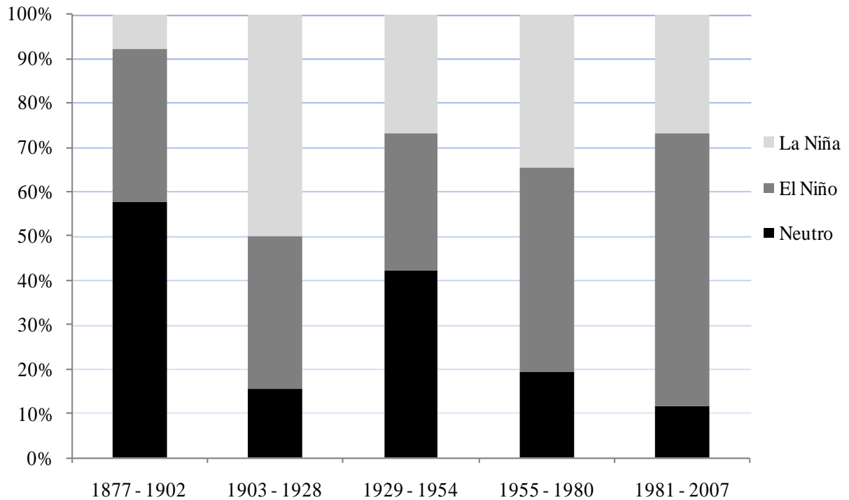
Figura 8 - Ocorrência relativa de anos Neutros, de El Niño e La Niña de 1877 a 2007, divididos em sub-períodos de 26 anos cada.
