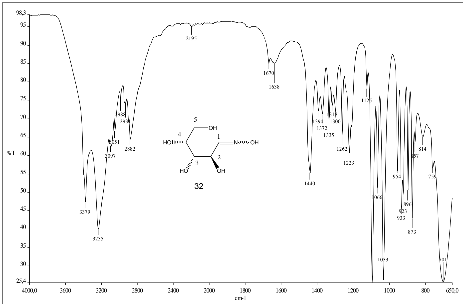
Figura 38 – Espectro no IV de 32 .
