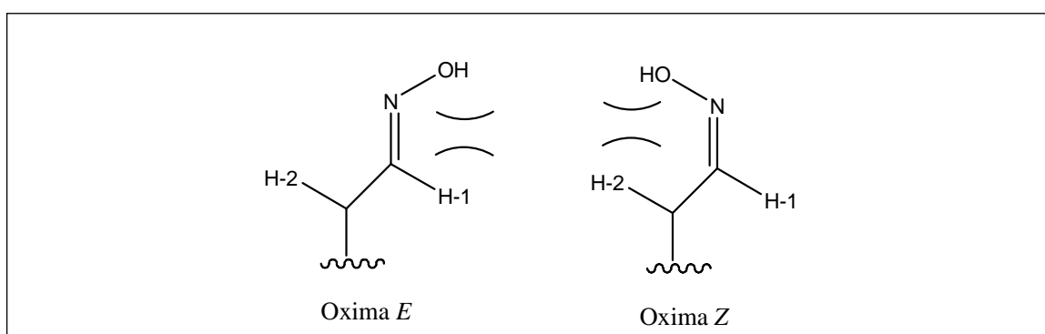
Figura 20 - Efeito de compressão estérica presente em aldoximas.
