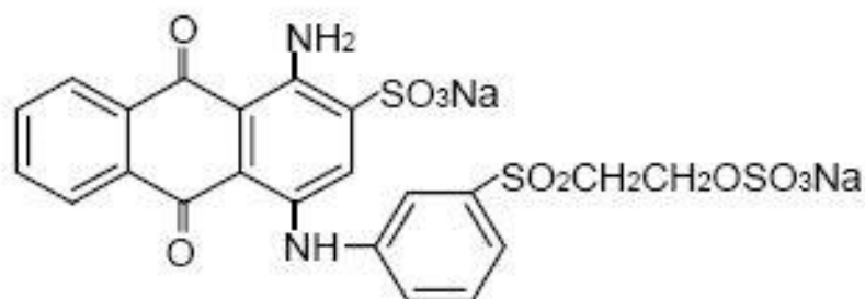
Figura 1. Estrutura química do corante azul reativo 19.
