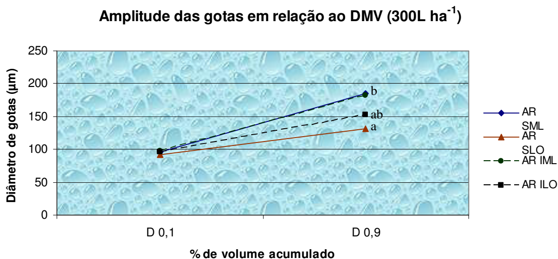
Figura 16. Amplitude relativa das gotas em papel hidrossensível após pulverização de cafeeiro com turbopulverizador hidráulico e volume de calda de 300 L.ha -1 . Campos Gerais, MG. Safra: 2007/2008.
