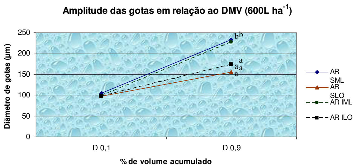
Figura 17. Amplitude relativa das gotas em papel hidrossensível, após pulverização de cafeeiro com turbopulverizador hidráulico e volume de calda de 600 L.ha -1 . Campos Gerais, MG. Safra: 2007/2008.
