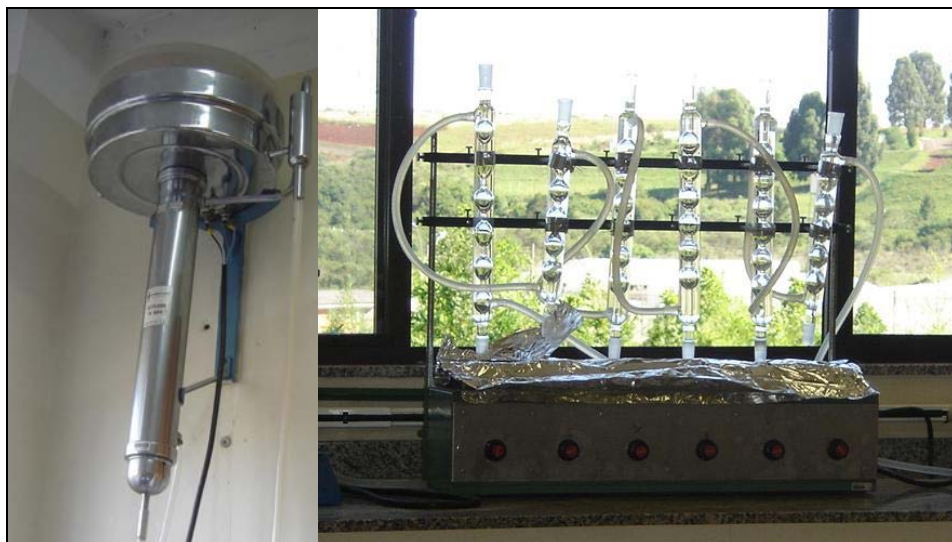
Figura 18 e 19: Destilador e condensador do laboratório de Físico-química – Engenharia de Alimentos – FEAR
