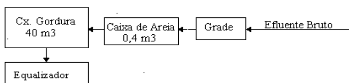
ESQUEMA ETE PARA TRATAMENTO DE EFLUENTE DE UM LATICÍNIO
