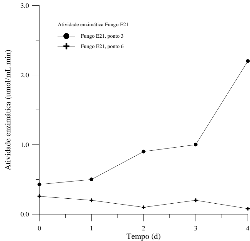
Figura 13i: Atividade lipolítica ( \mu\text{molAG/mL.min} ) versus tempo de fermentação do fungo E21. Ponto 3: saída do equalizador; Ponto 6: saída do tanque de aeração.
