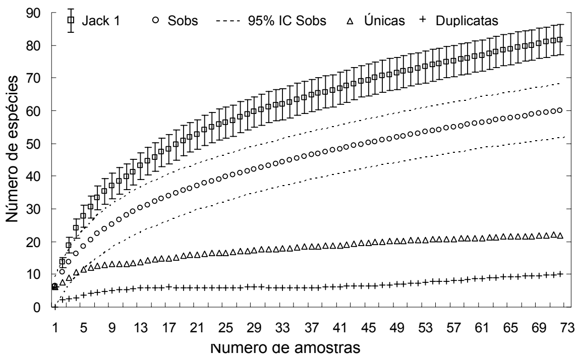
Figura 11 – Curva geral de acumulação da riqueza de espécies de formigas ponerines (estimadas, observadas, únicas e duplicatas) em 72 amostras de serapilheira na ECFPn, Caxiuanã, Melgaço, Pará, Brasil. Jack 1= estimador Jackknife 1 indicando o desvio padrão; Sobs= riqueza observada - Mao Tau; IC= intervalo de confiança; únicas= espécies com um registro; e duplicatas= espécies com dois registros.
