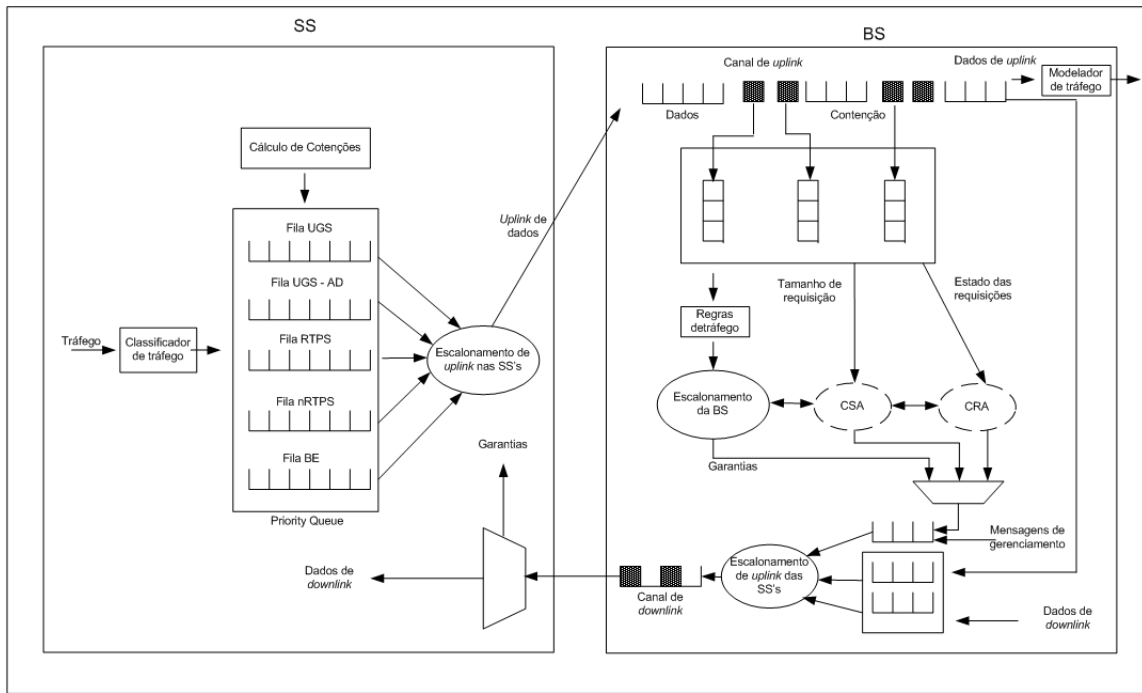
Figura 4.6: Arquitetura de QoS, proposta por Chu et al.
