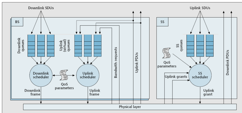
Figura 4.9: Funções dos schedulers para garantia de QoS, propostas por Cicconetti et al.
