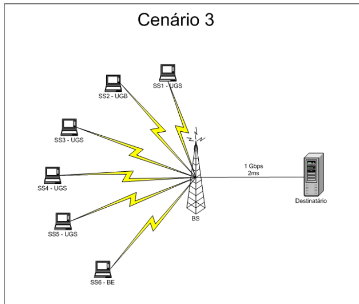
Figura 5.10: Estrutura da rede para o cenário 3
