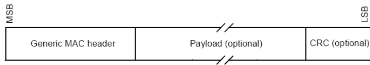
Figura 3.12: Formato do MAC PDU
