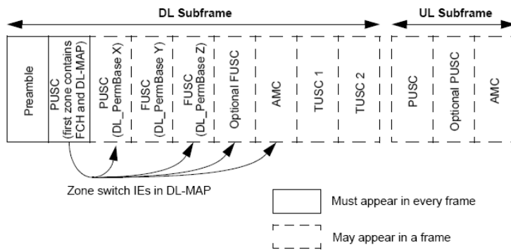
Figura 3.8: Múltiplas zonas permitidas no frame OFDMA
