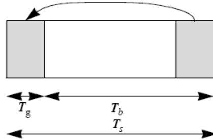
Figura 3.4: Representação do símbolo OFDM
