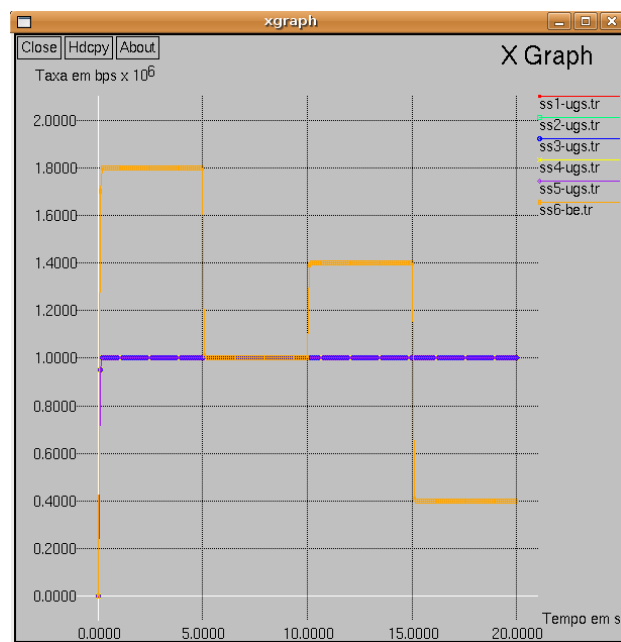
Figura 5.12: Gráfico da Taxa de transmissão X tempo, deste trabalho, para o Cenário 3
