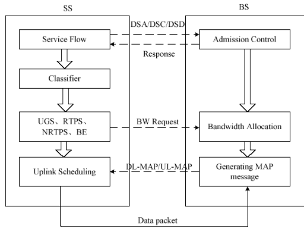
Figura 4.10: Arquitetura de QoS, proposta por Lilei et al.
