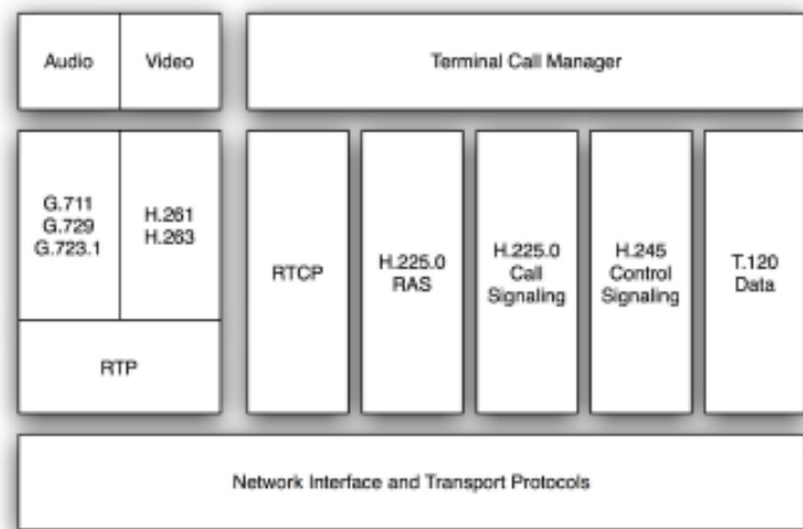
Figura 2.3: Pilha de protocolos para serviços VoIP utilizando H323
