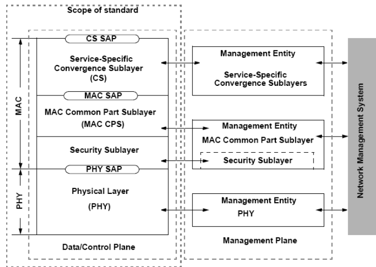
Figura 3.11: Modelo de referência da estrutura em camadas
