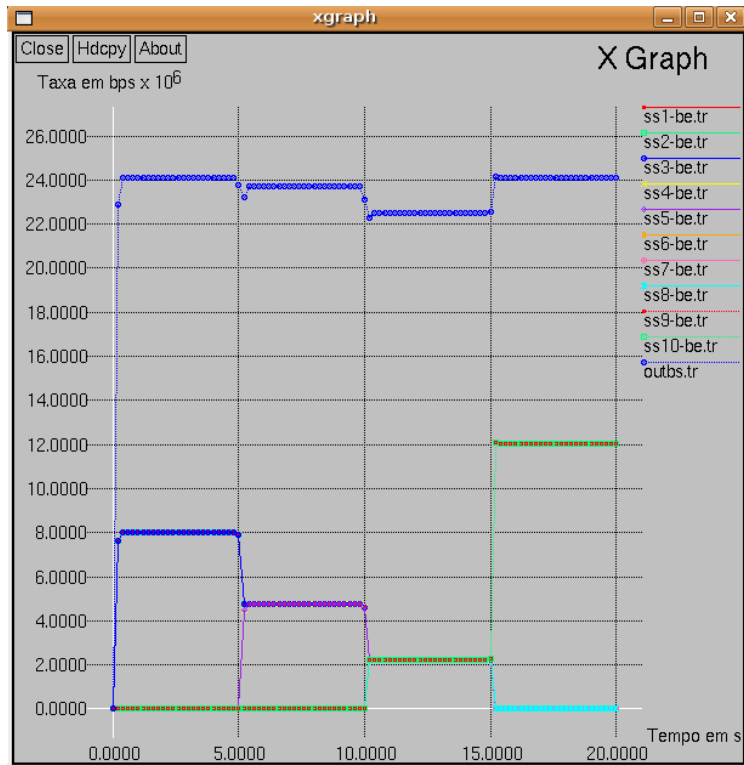
Figura 5.3: Gráfico da Taxa de transmissão X tempo, deste trabalho, para o Cenário 1
