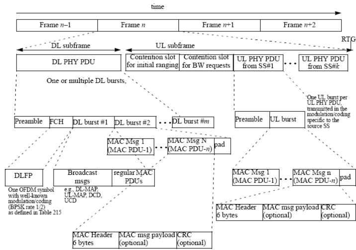
Figura 3.5: Frame para camada física WirelessMAN-OFDM operando em PMP.
