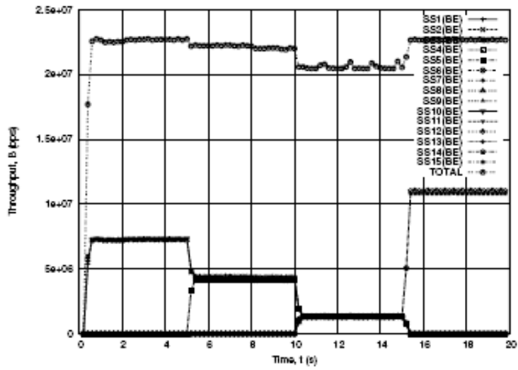
Figura 5.2: Gráfico da Taxa de transmissão X tempo, para o Cenário 1 em Sayenko et al.
