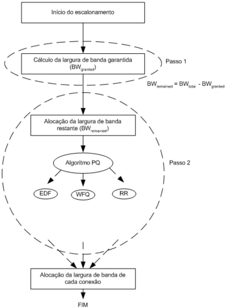
Figura 4.11: Algoritmo QBMS
