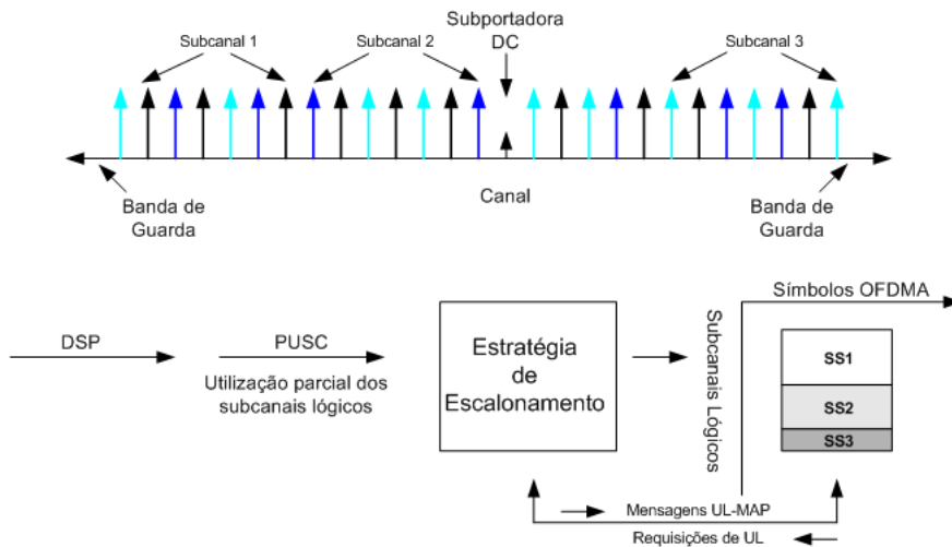
Figura 3.9: Diagrama esquemático da função do scheduler na alocação de subcanais lógicos
