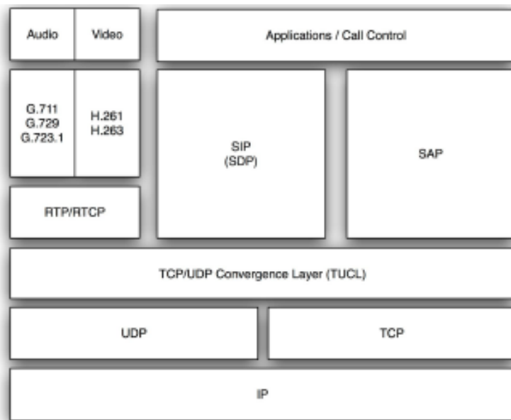
Figura 2.1: Arquitetura Funcional para serviços VoIP
