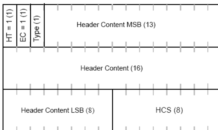
Figura 3.15: Cabeçalho de sinalização sem payload - Tipo II
