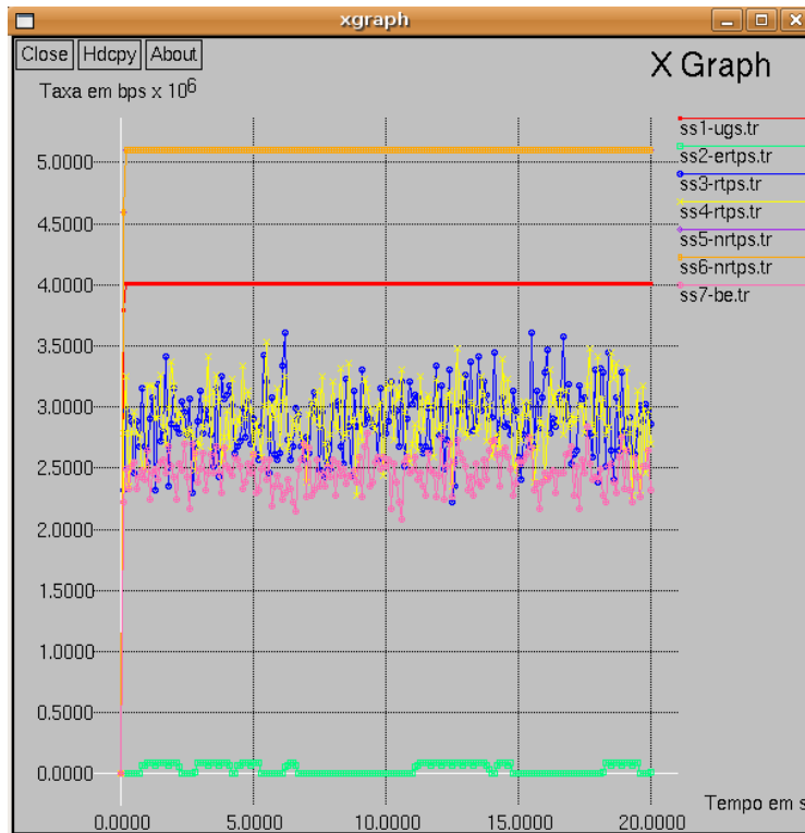
Figura 5.7: Resultado do cenário 2 - DL/UL - 3:1
