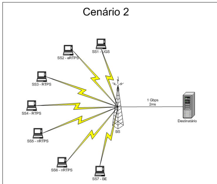
Figura 5.4: Estrutura da rede para o cenário 2
