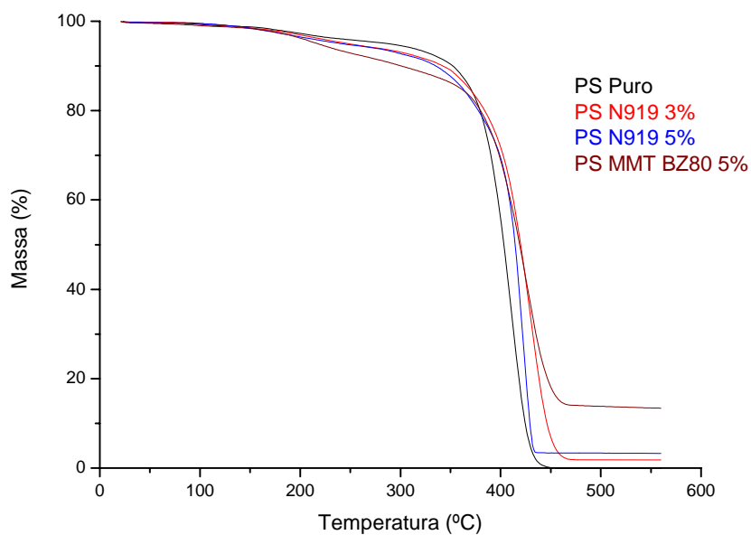
Figura 4.13 – Comparativo ATG PS e diferentes nanocompósitos.
