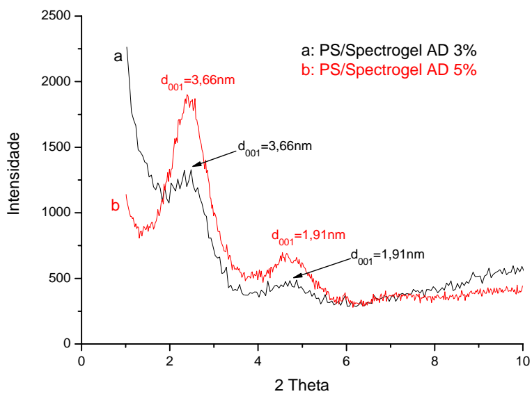
Figura 3.22 – Comparativo DRX PS/Spectrogel AD 3 e 5%.
