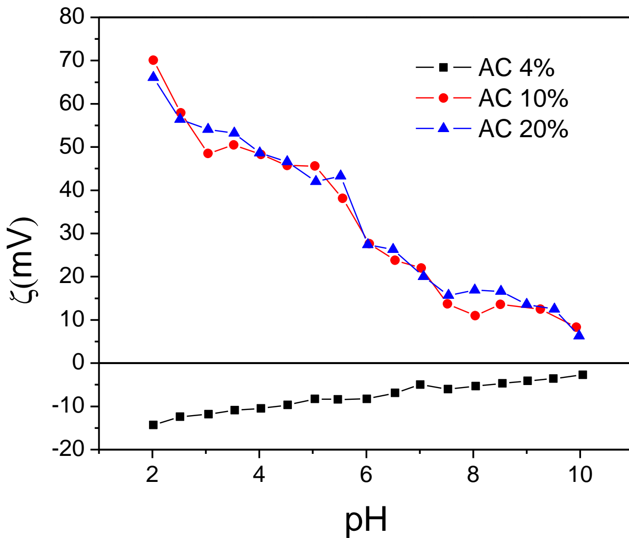
Figura 22: Efeito da adiço de amido catinico (AC) nas disperses de fibras de celulose e PCC, (a) 4% em massa de AC; (b) 10% em massa de AC; (c) 20% em massa de AC e (d) todos juntos para efeito de comparao.
