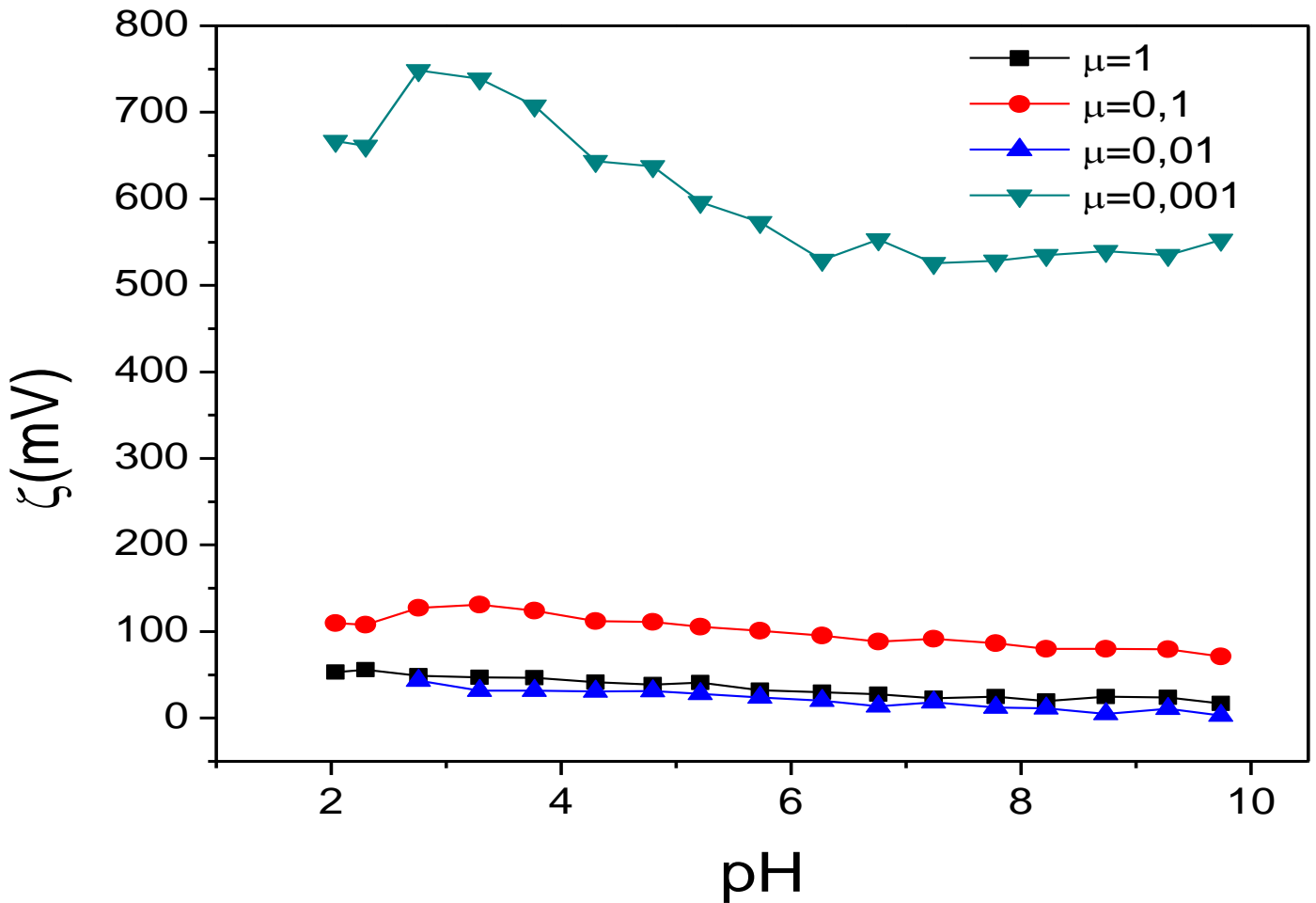
Figura 20: Efeito da força iônica (ajustada com eletrólito simétrico, NaCl) sobre o potencial zeta em suspensão de fibra de celulose e carbonato de cálcio.
