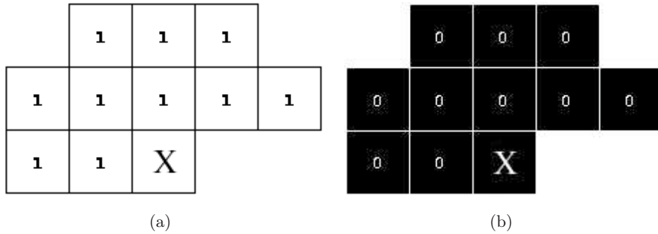
Figura 2.13: As frequências de ocorrência de 0's e 1's estão condicionadas a dois contextos, (a) C_1 e (b) C_2 . Nas figuras, X representa o pixel a ser codificado.
