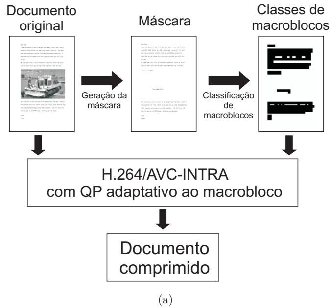
Figura 5.6: H.264/AVC-INTRA - Composto ou AVC-C : esquema do codificador proposto.
