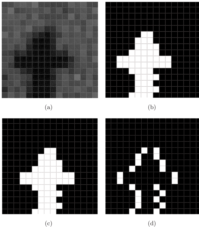
Figura 4.7: (a) Macrobloco original; (b) \bar{m}_n(i, j) : máscara invertida relativa ao limiar t_n = 36 . (c) \bar{m}_{nd}(i, j) máscara deslocada de uma coluna à direita; e (d) valor absoluto da diferença entre \bar{m}_n(i, j) e \bar{m}_{nd}(i, j) , ou seja, \bar{m}_{ndif}(i, j) = |\bar{m}_n(i, j) - \bar{m}_{nd}(i, j)| .
