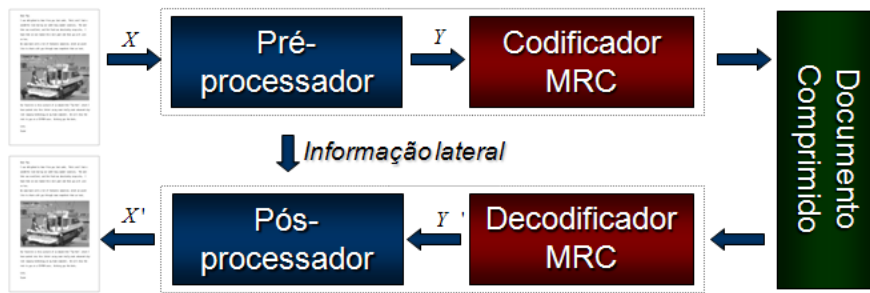
Figura 7.1: Ilustração das etapas de pré-processamento, codificação, decodificação e pós-processamento.
