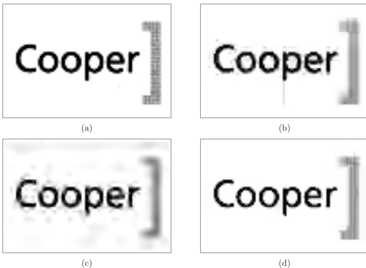
Figura 7.20: Comparação entre codificadores. Parte ampliada 1 do documento “IEEE3”: (a) original; (b) codificado e reconstruído com o AVC-I (PSNR = 26,5116 dB); (c) codificado e reconstruído com o JPEG2000 (PSNR = 23,9971 dB); (d) codificado e reconstruído com o codificador MRC proposto (PSNR = 24,2050 dB). A taxa de bits observada foi aproximadamente 0,19 \text{ bit/pixel} .
