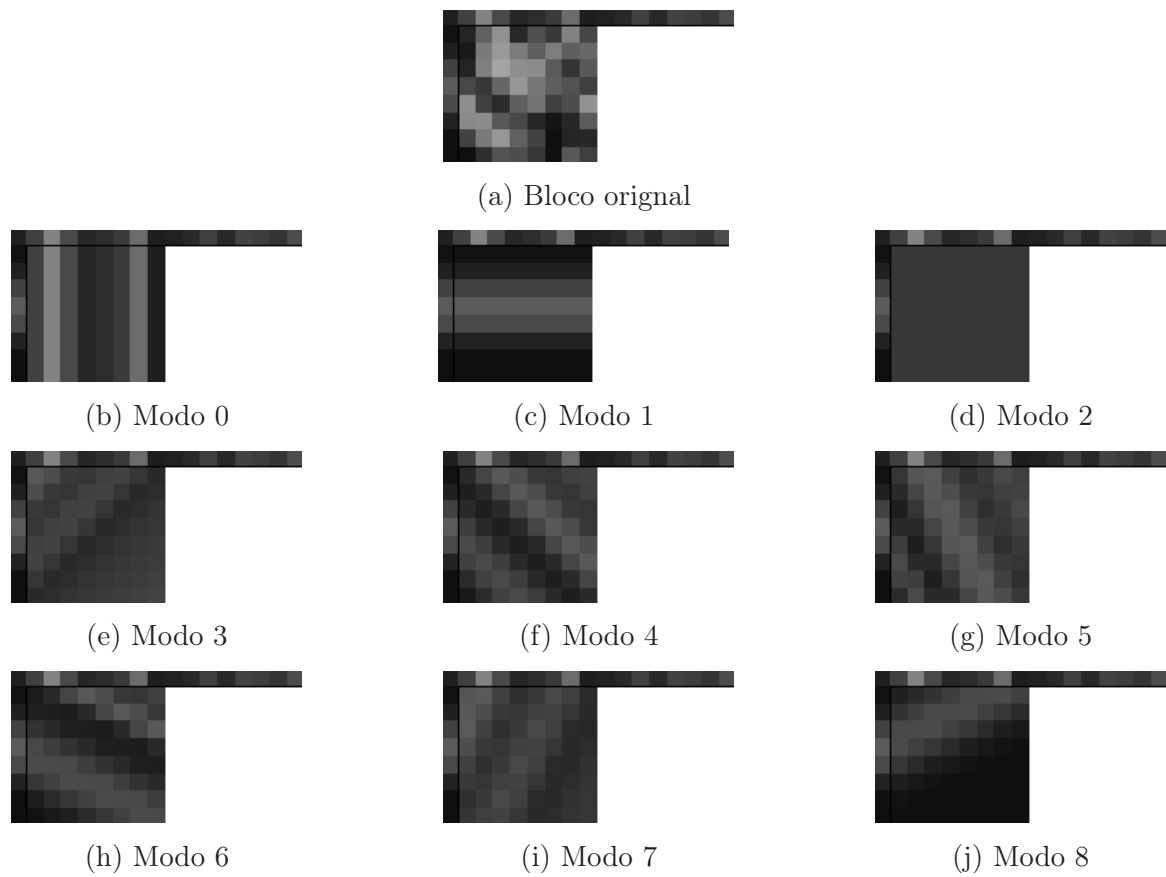
Figura 3.12: Exemplo de previsões I8 : (a) bloco original a ser predito; (b) a (j) previsões geradas a partir dos modos de previsão 0 a 8, respectivamente.
