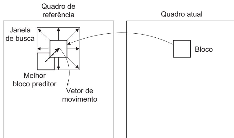
Figura 3.4: Estimação de movimento.
