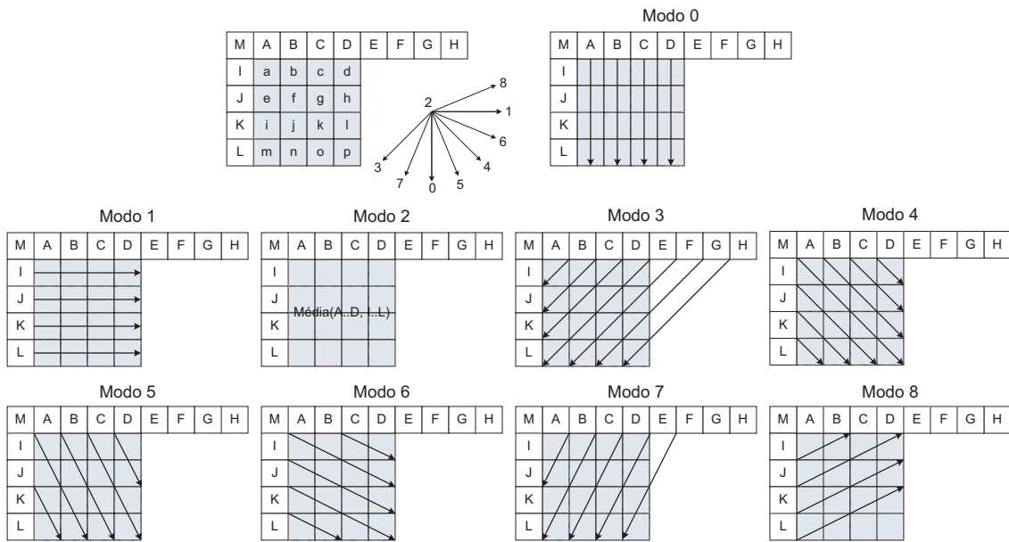
Figura 3.9: Predição intra para blocos de luminância com tamanho 4 \times 4 pixels. Oito “direções de predição” e modo DC.
