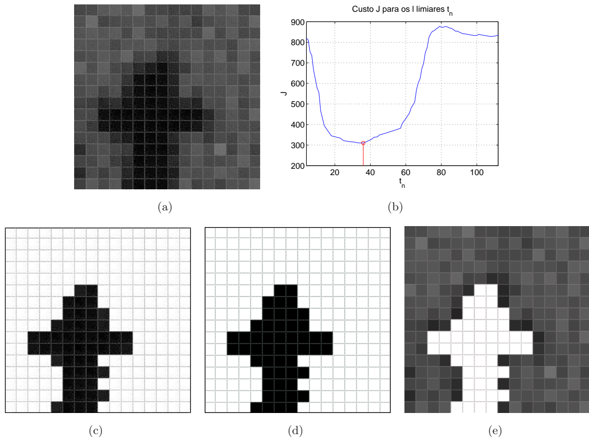
Figura 4.8: Exemplo de segmentação: (a) macrobloco original; (b) custo observado para cada um dos possíveis limiares t_n ; (c), (d) e (e) representam o FG, a máscara e o BG, respectivamente, para t_n = 36 .
