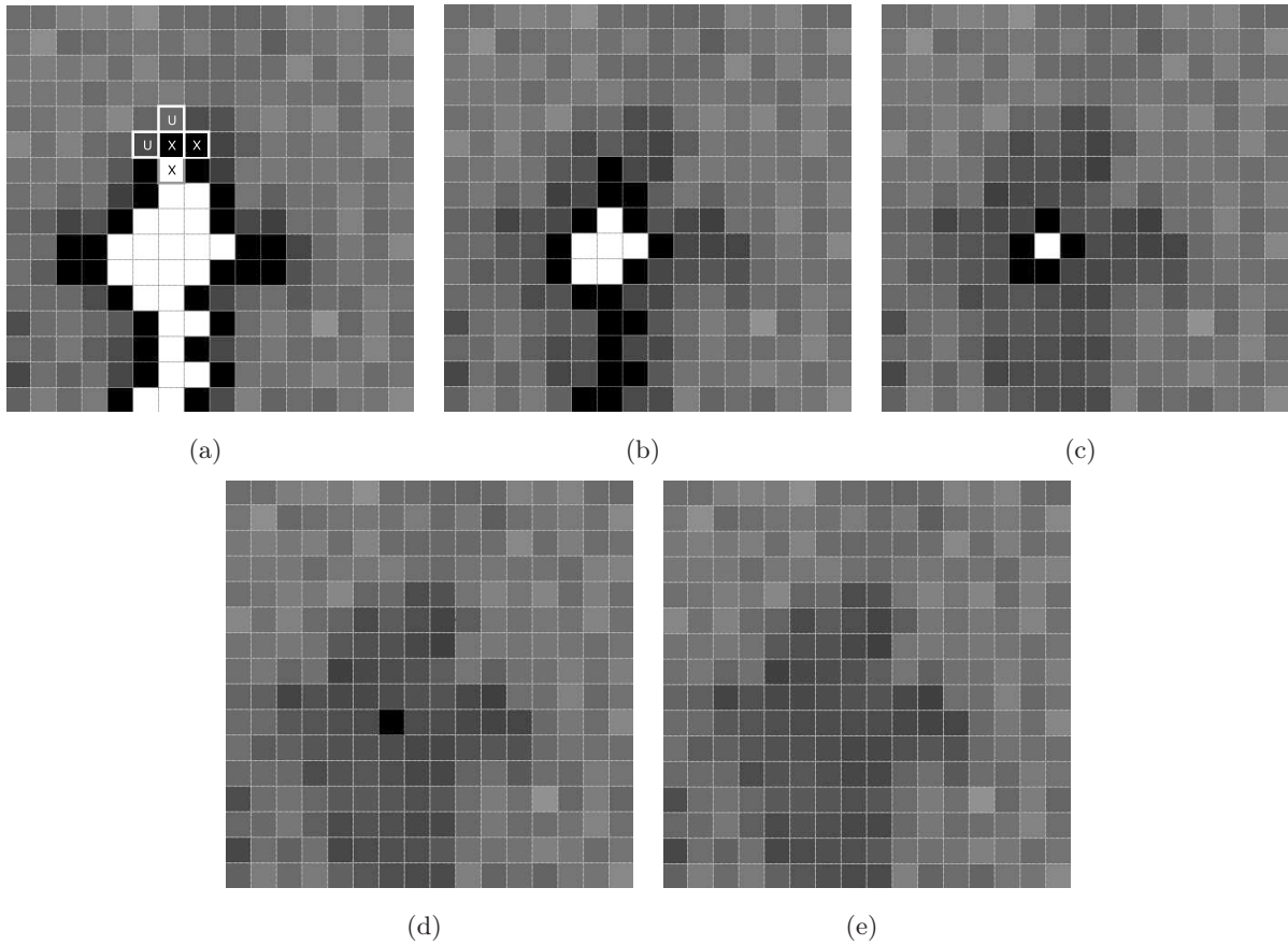
Figura 4.12: Exemplo de preenchimento iterativo no domínio espacial: em cada etapa, as cores preta e branca indicam os pixels irrelevantes que estão sendo processados na etapa atual e os que serão processados e etapas futuras, respectivamente.
