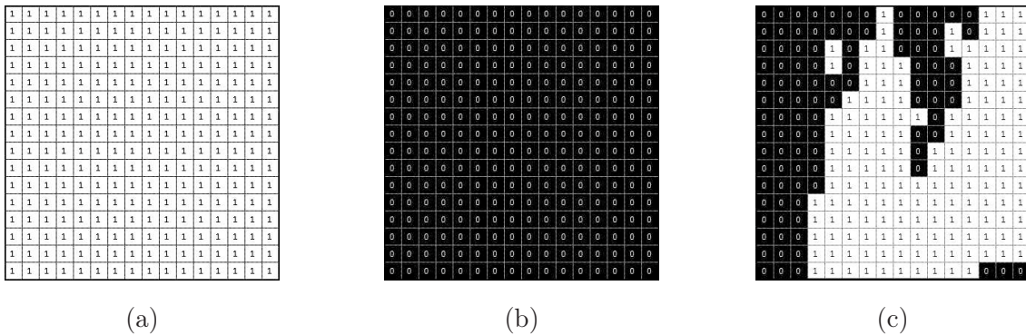
Figura 5.4: Exemplos das classes de macroblocos: (a) classe 0 (regiões pictóricas), (b) classe 1 (regiões de interior de texto) e (c) classe 2 (regiões de borda de texto).
