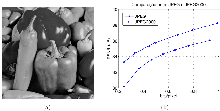
Figura 2.23: Comparação entre o JPEG e o JPEG2000: (a) imagem “peppers”; e (b) curvas PSNR para a imagem “peppers”.
