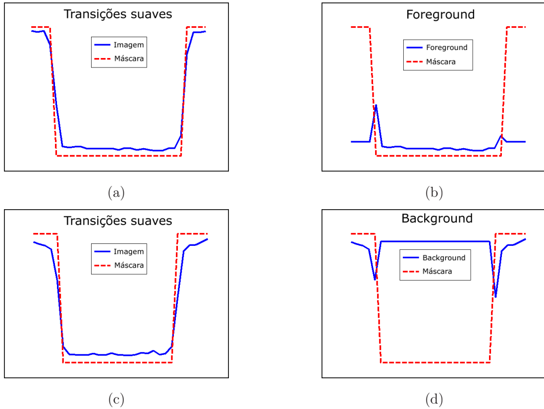
Figura 7.2: Exemplos em uma dimensão do efeito da segmentação em transições suaves. Em (a) e (c) duas transições e suas respectivas máscaras, indicadas em linhas pontilhadas, podem ser observadas. No planos (b) FG e (d) BG, as respectivas regiões irrelevantes são substituídas por valores constantes, enquanto parte das transições não, causando os picos indesejáveis.
