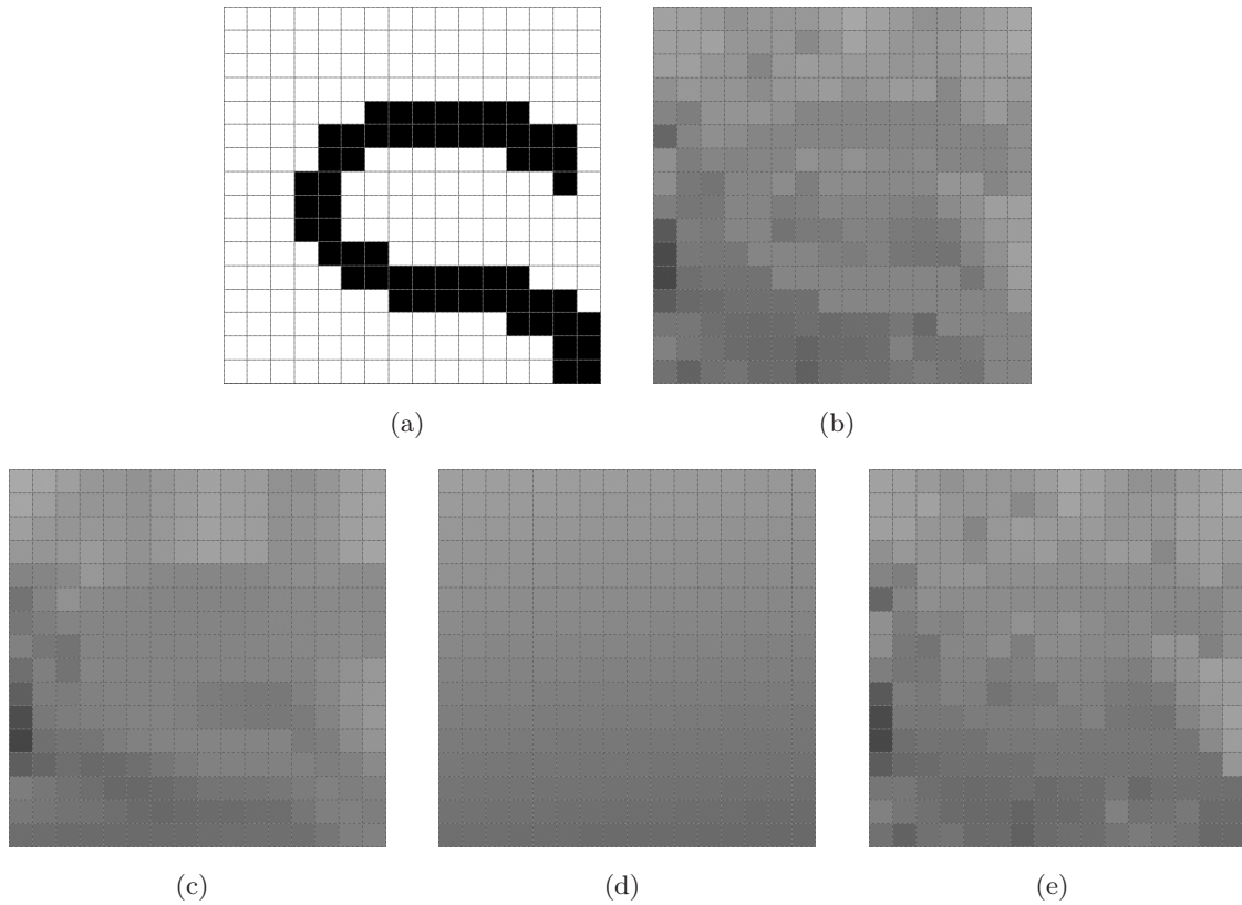
Figura 6.1: Data-filling baseado nas previsões I16 do AVC-I: (a) máscara binária; (b) BG_0 ; (c) BG'_0 ( QP = 30 ); (d) BG_{pred} ; e (e) BG_{df} .
