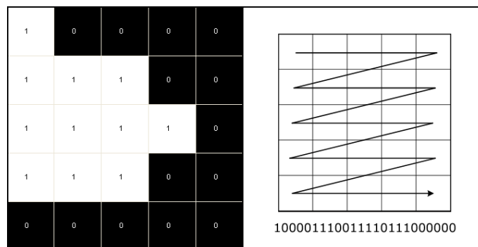
Figura 2.10: Imagem binária representada como um fluxo de dígitos binários unidimensional, organizado a partir da varredura raster .
