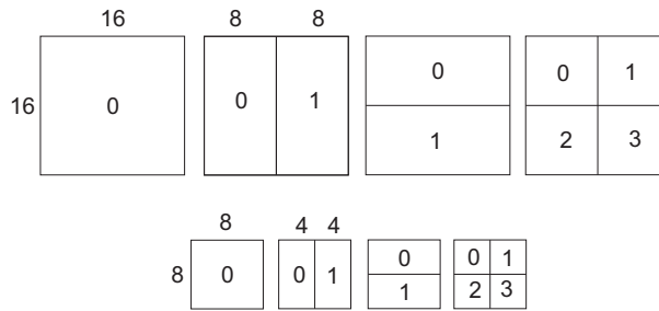
Figura 3.6: Partição com tamanho de bloco variável. Os números ao redor dos blocos representam suas dimensões em pixels .
