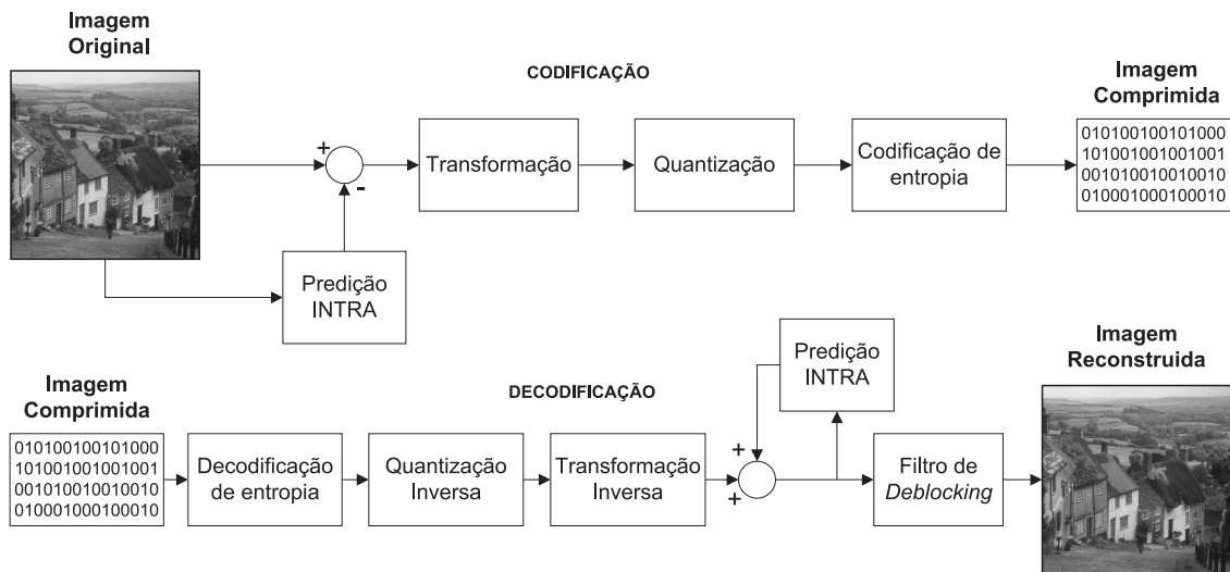
Figura 3.16: Diagrama de blocos do AVC-I: codificação e decodificação.
