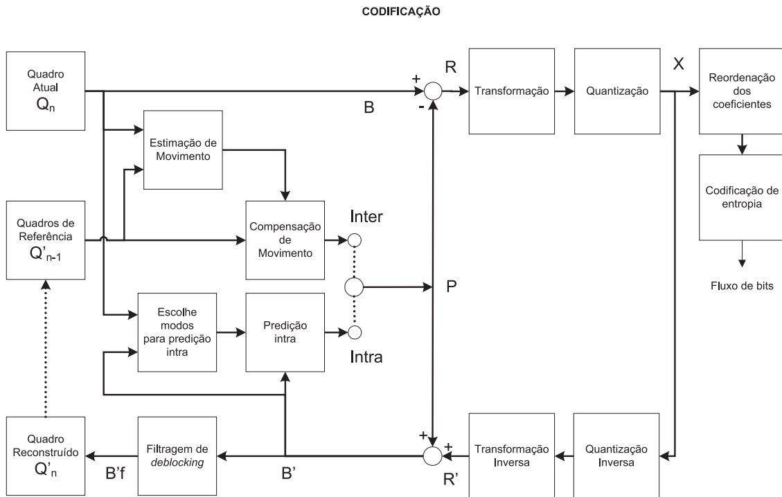
Figura 3.7: Codificação H.264/AVC.
