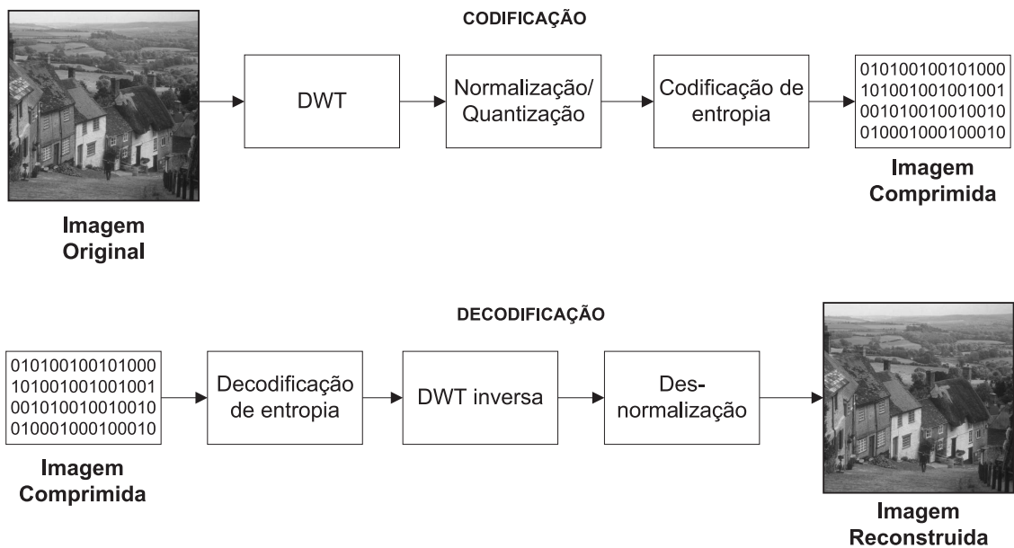
Figura 2.18: Diagrama de blocos do JPEG2000: codificação e decodificação.
