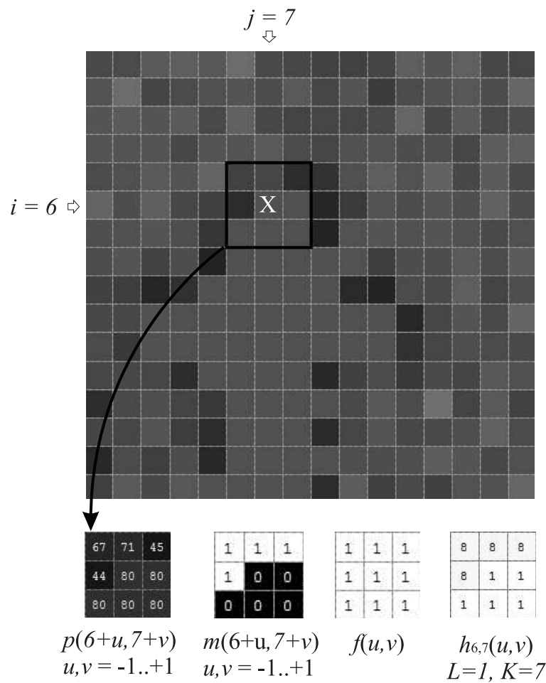
Figura 4.15: Exemplo de preenchimento utilizando filtragem segmentada. A amostra X = p_f(6, 7) é determinada a partir da filtragem segmentada que utiliza o filtro variante ao deslocamento h_{6,7}(u, v) . No exemplo, p_f(6, 7) = (8 \cdot (67 + 71 + 45 + 44) + 5 \cdot 80) / 37 = 60 . Para o melhor entendimento do exemplo, sugere-se a análise atenta das Equações 4.22 e 4.23.
