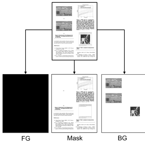
Figura 4.2: Ilustração do modelo de imageamento MRC. O documento original é representado utilizando-se três camadas: Foreground (FG), Background (BG) e máscara ( Mask ).
