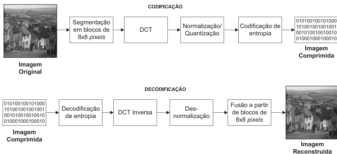
Figura 2.15: Diagrama de blocos do JPEG: codificação e decodificação.
