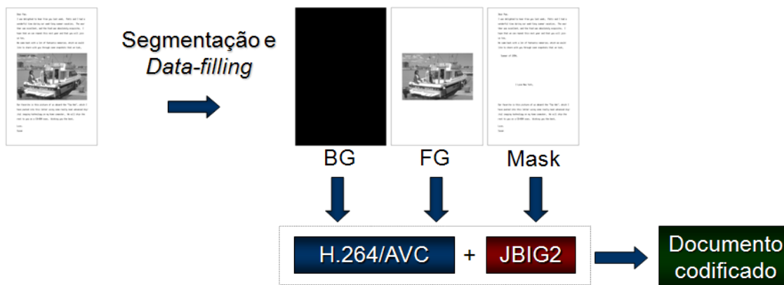
Figura 6.2: Codificador MRC proposto: propõe-se um codificador que utiliza o H.264/AVC na compressão dos planos FG e BG, e o JBIG2 na compressão da máscara binária.
