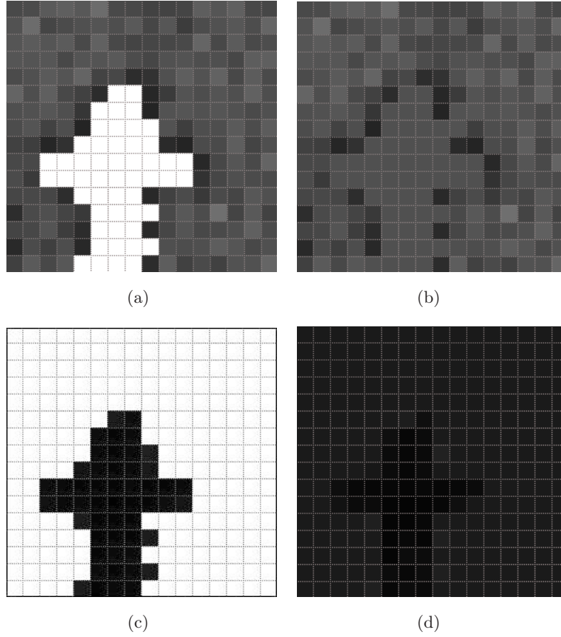
Figura 4.11: Exemplo de preenchimento por valor constante igual à média: (a) e (c) BG e FG; (b) e (d) BG_{df} e FG_{df} , versões processadas de BG e FG, respectivamente.
