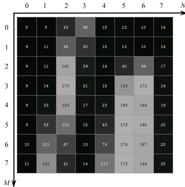
Figura 2.9: Exemplo de imagem com M = 8 linhas, N = 8 colunas e K = 256 níveis de cinza. Cada quadrado representa um pixel . O número no interior dos pixels indica o nível de cinza a que pertencem.
