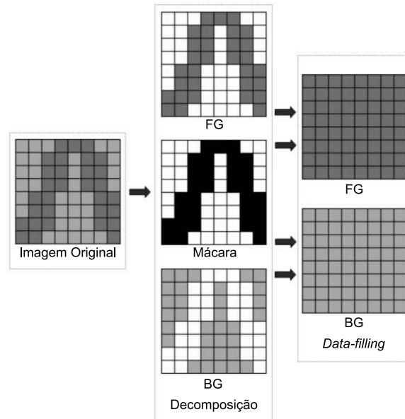
Figura 4.10: Diagrama que ilustra a decomposição MRC e o procedimento de data-filling .
