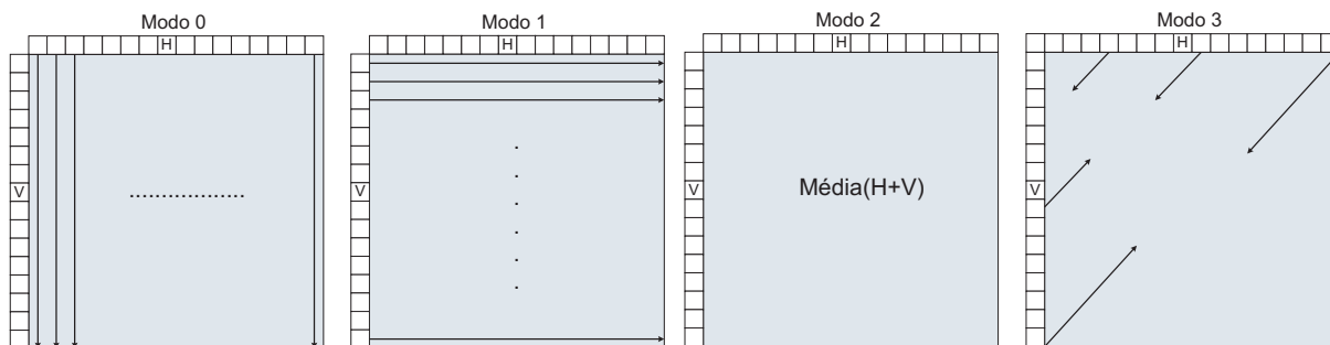
Figura 3.13: Predição intra para blocos de luminância com tamanho 16 \times 16 pixels .
