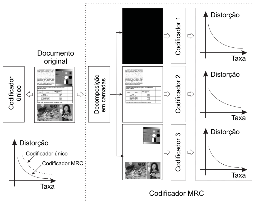
Figura 4.5: Cada plano do modelo MRC pode ser processado e comprimido por meio de algoritmos específicos, resultando em um comportamento global de taxa e distorção mais eficiente do que a abordagem baseada em um codificador único.
