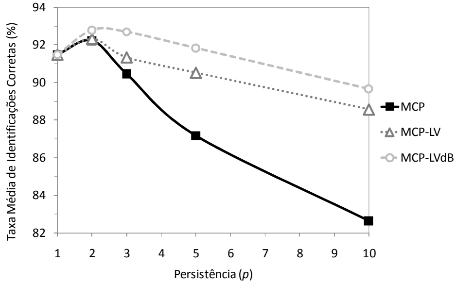
Figura 4.18: Taxa média de identificações corretas de sistemas de RAL multicondicionais MCP, MCP-LV e MCP-LV dB , em função do valor de persistência, p .
