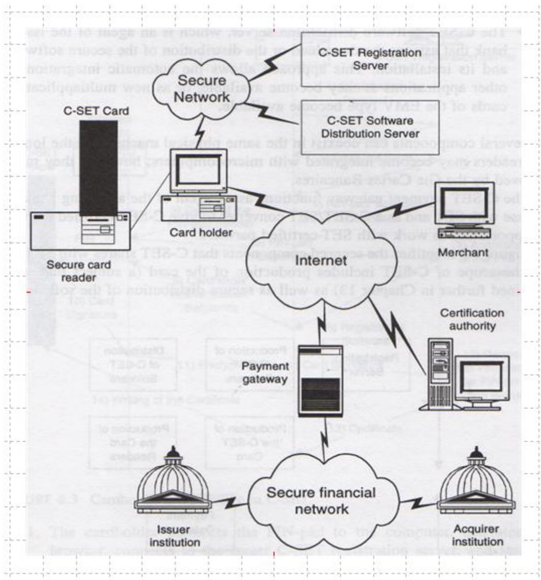
Gráfico 4-13 – Arquitetura geral do cSET
