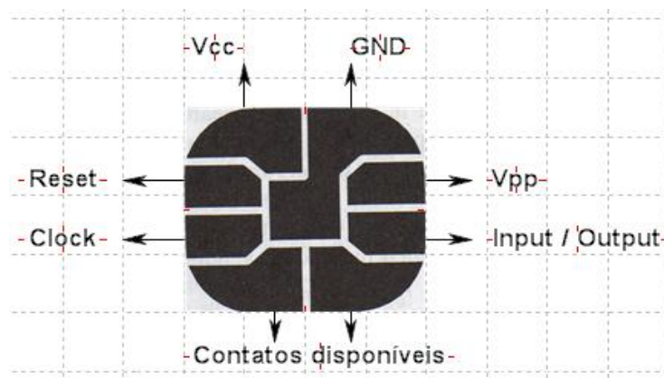
Gráfico 3-6 – Representação dos oito contatos de um circuito integrado de cartões inteligentes.
