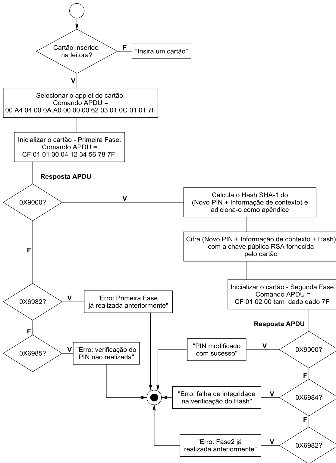
Gráfico 6-14 – Inicialização do cartão inteligente
