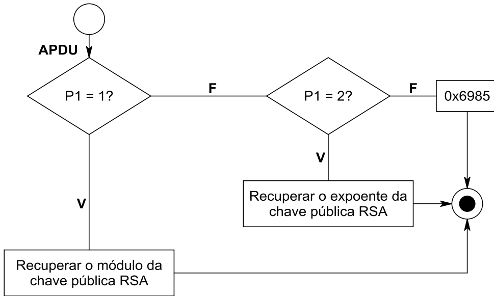
Gráfico 6-8 – Recuperar Chave Pública para Cifrar
