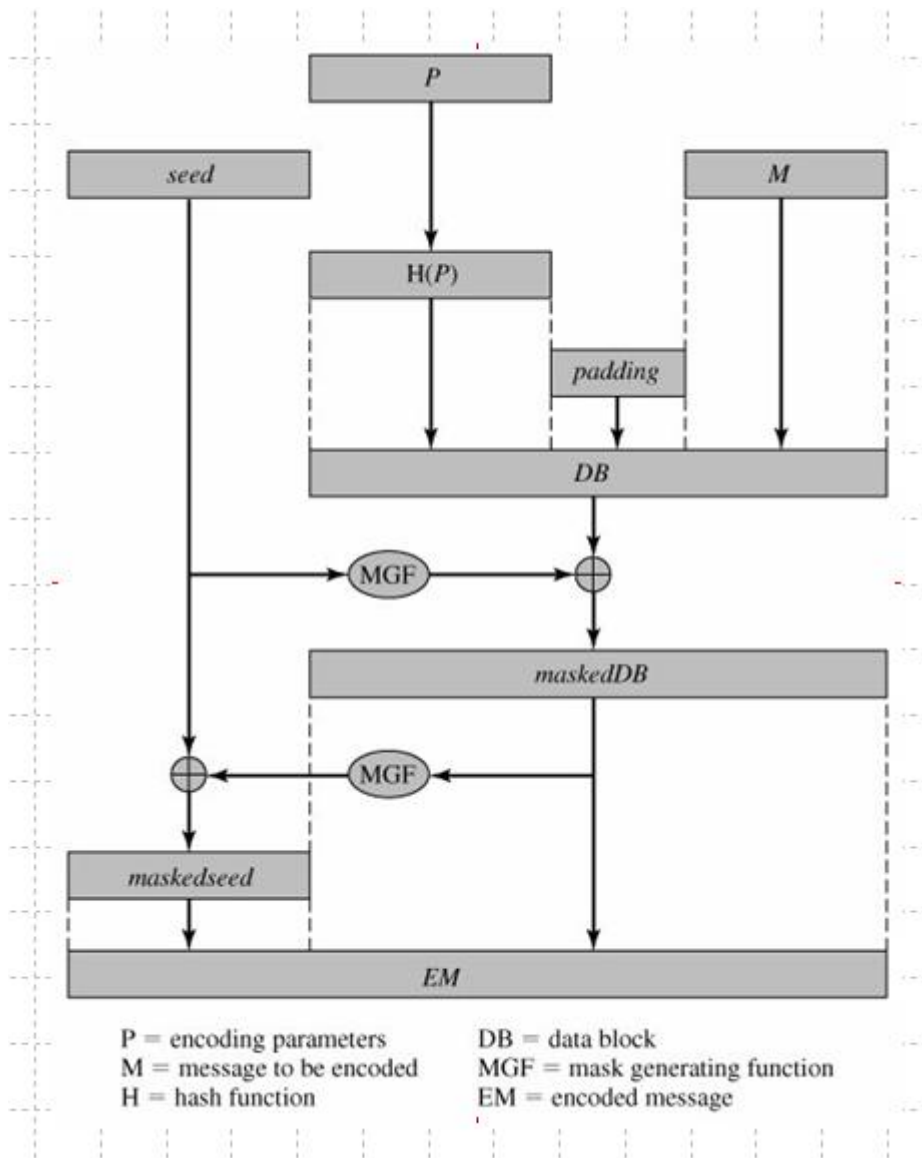
Gráfico 2-3 – Optimal Asymmetric Encryption Padding (OAEP) .
