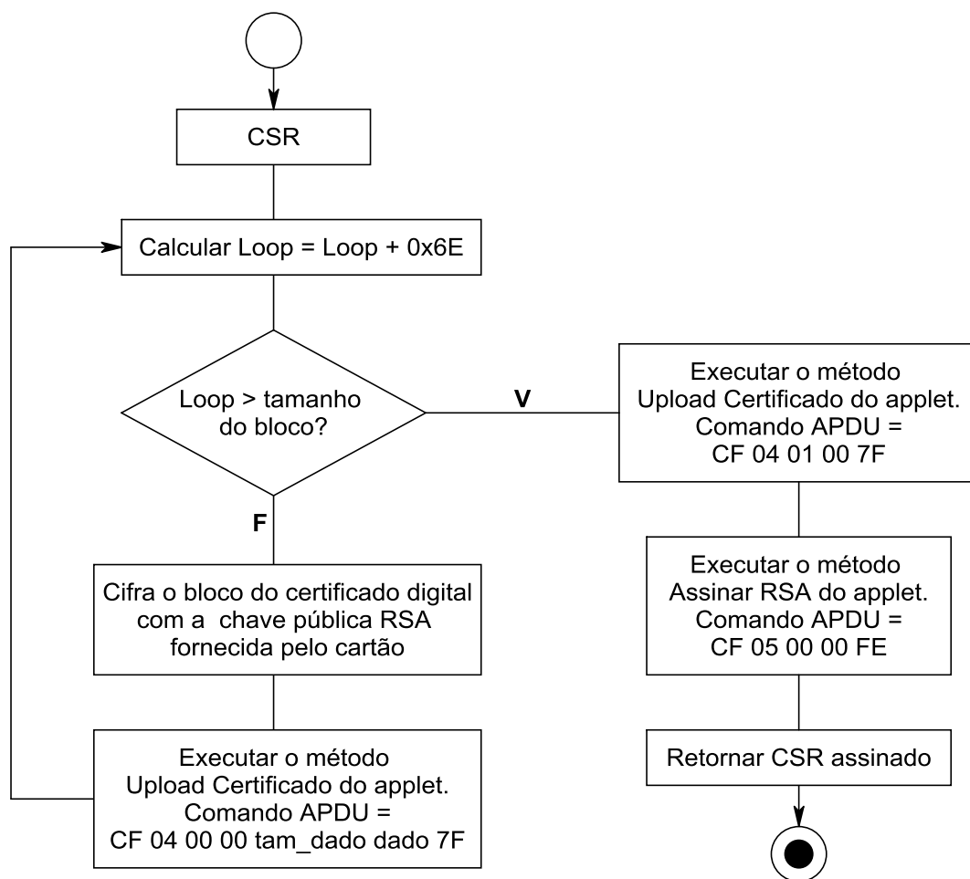
Gráfico 6-19 – Assinatura no Cartão
