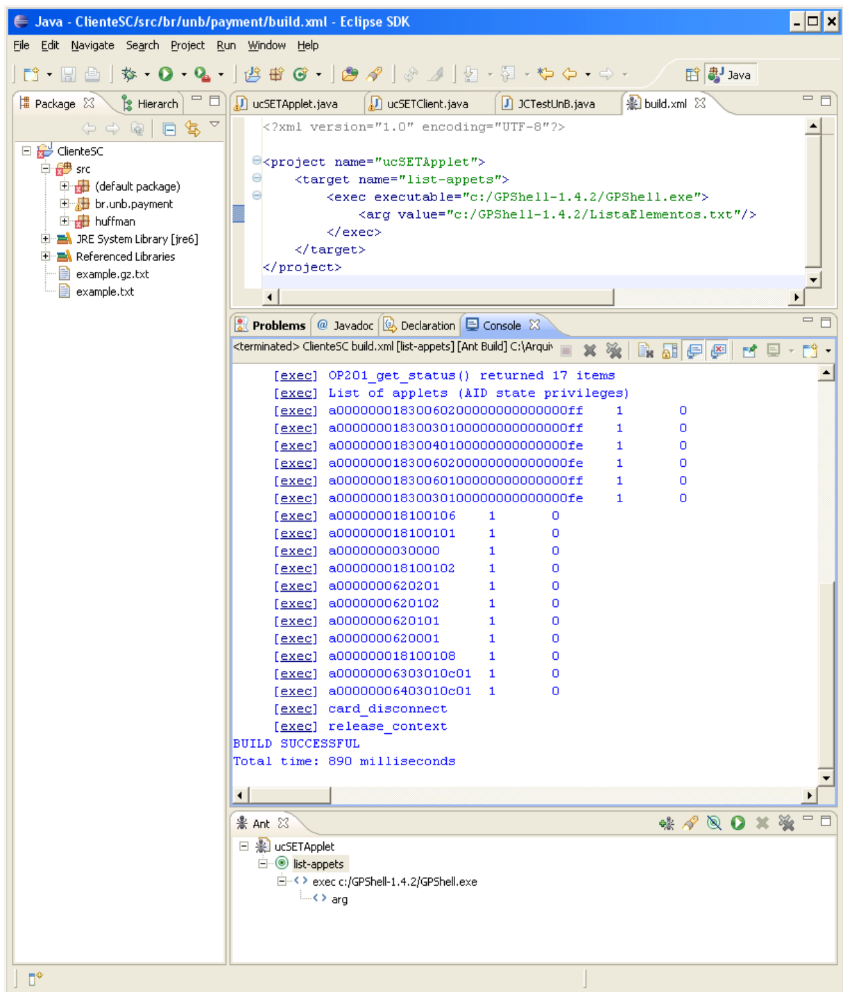
Gráfico A-1 – Saída na console do Eclipse para o script Ant de listagem
