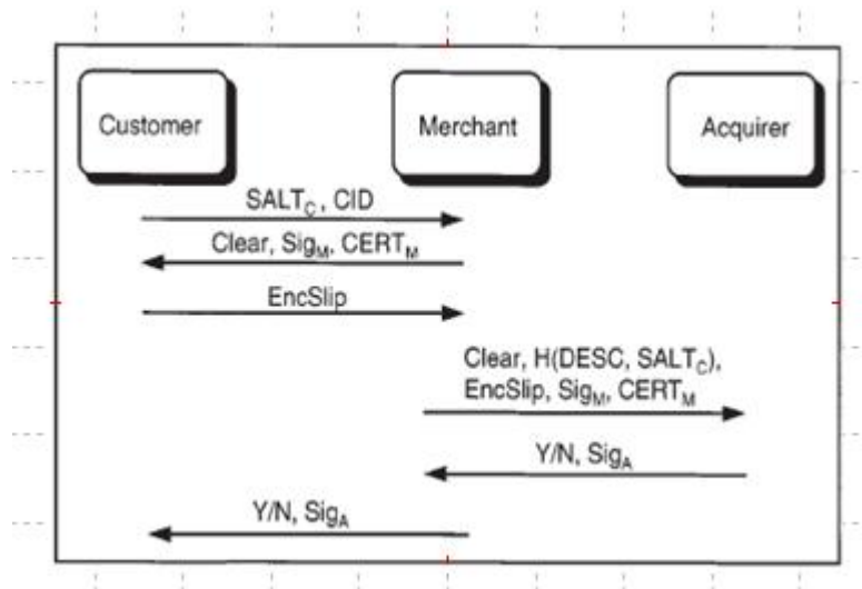
Gráfico 4-11 – Fluxo de mensagens no 2KP
