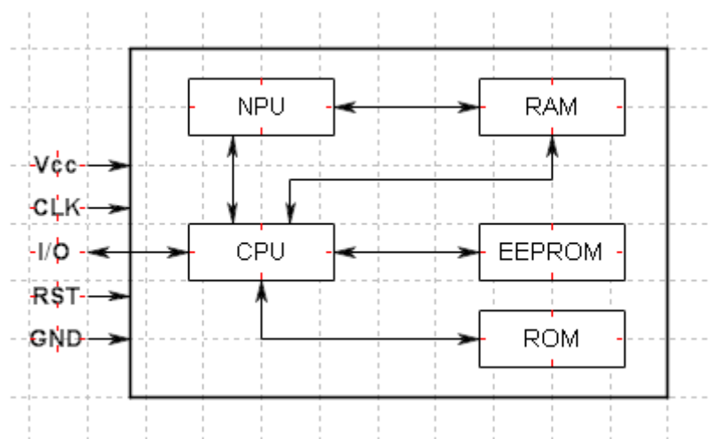
Gráfico 3-8 – Esquemático básico de um microcontrolador de um cartão inteligente.
