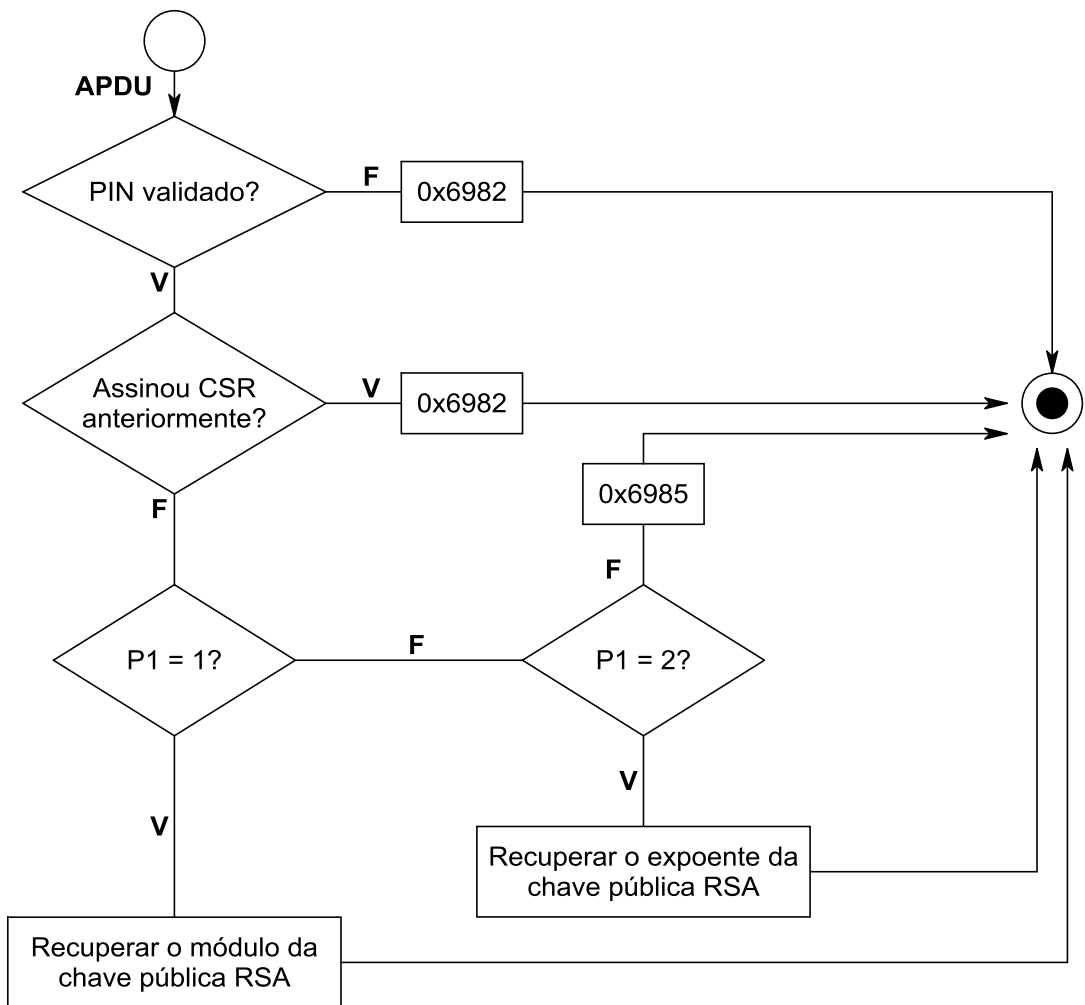
Gráfico 6-9 – Recuperar Chave Pública para Assinar
