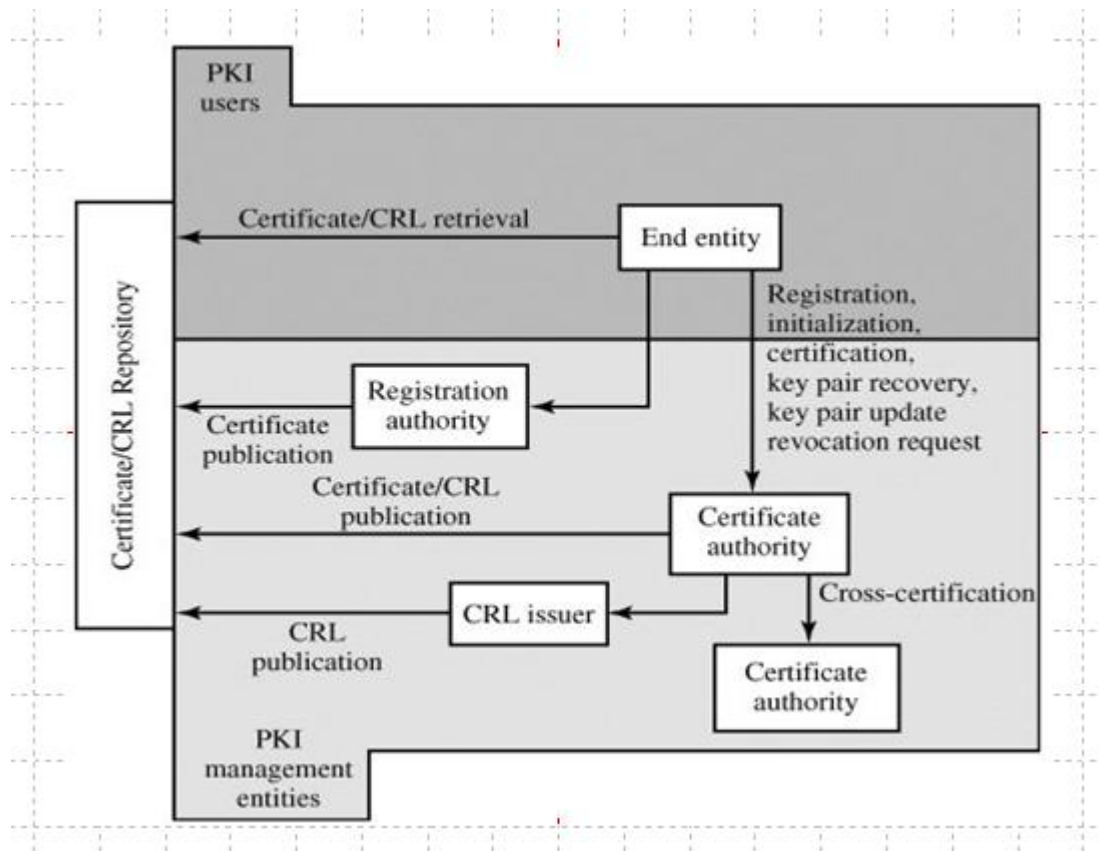
Gráfico 2-7 – Arquitetura PKIX.
