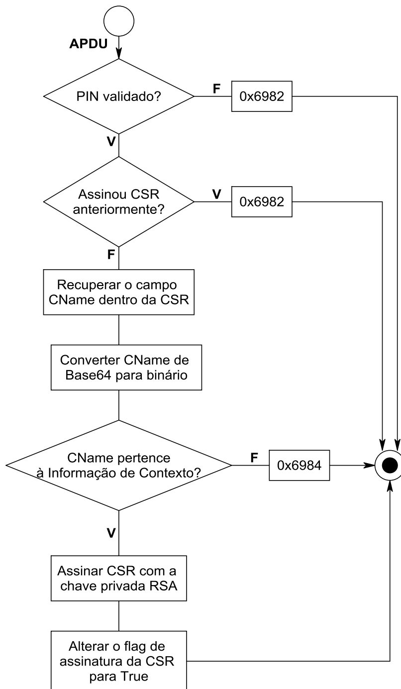
Gráfico 6-11 – Assinar RSA
