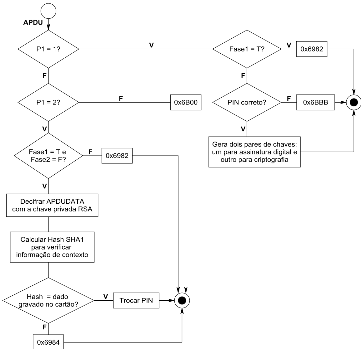
Gráfico 6-6 – Inicializar Cartão
