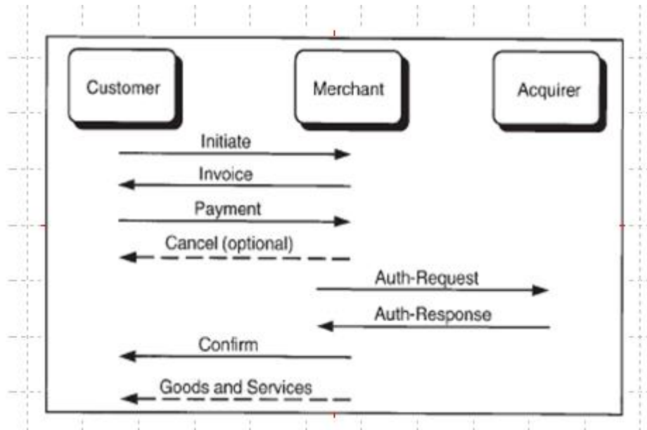
Gráfico 4-9 – Fluxo de mensagens no iKP
