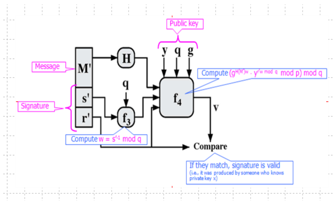
Gráfico 2-5 – Verificação da assinatura DSS.
