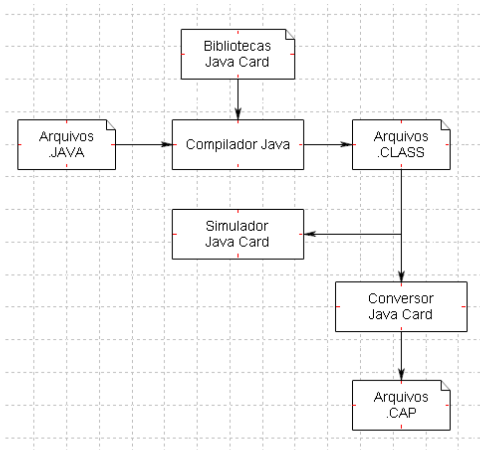
Gráfico 3-12 – Criação de um applet Java Card.
