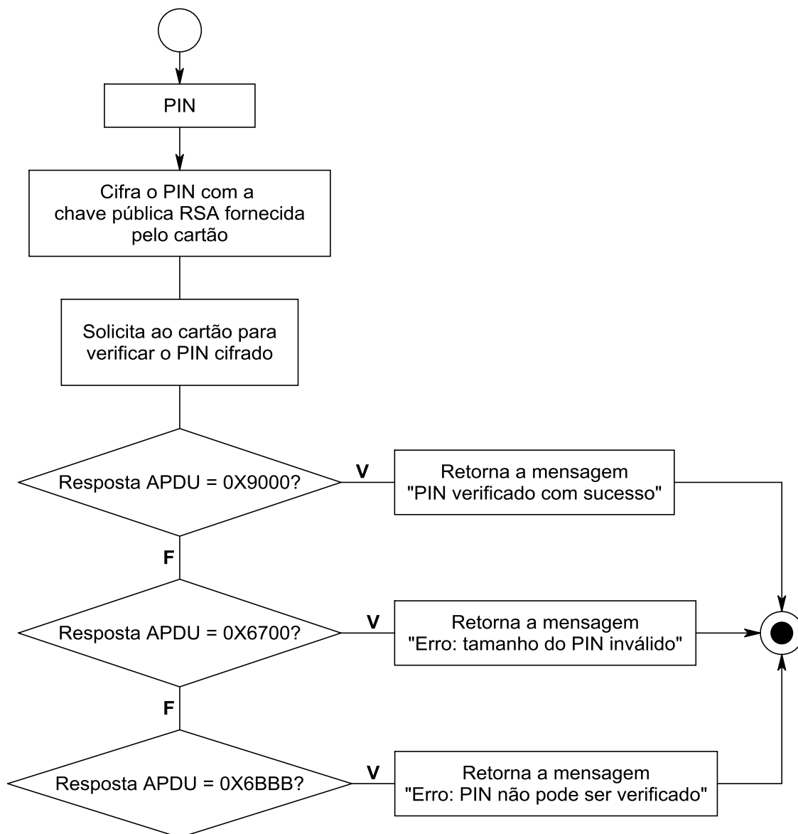
Gráfico 6-15 – Verificação do PIN
