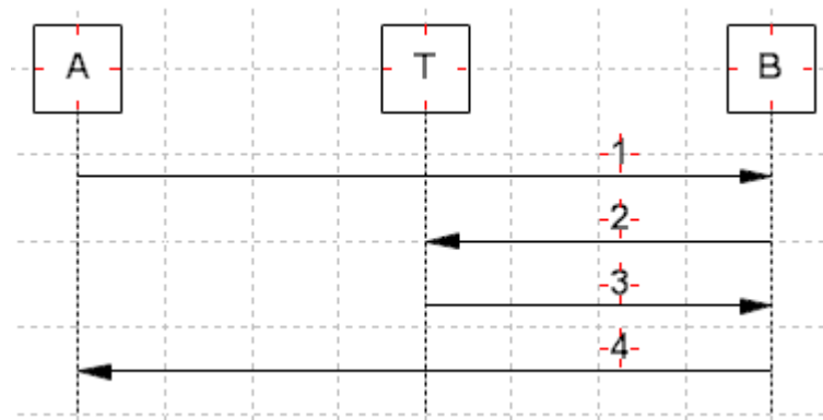
Gráfico 4-4 – Exemplo para o caso de cifrar apenas quando necessário.
