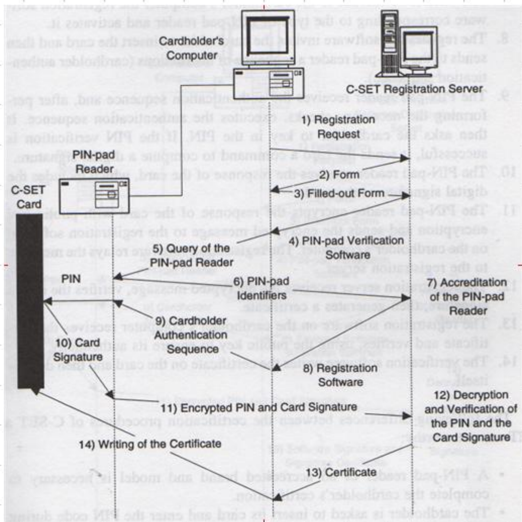
Gráfico 4-14 – Procedimento de Registro no cSET
