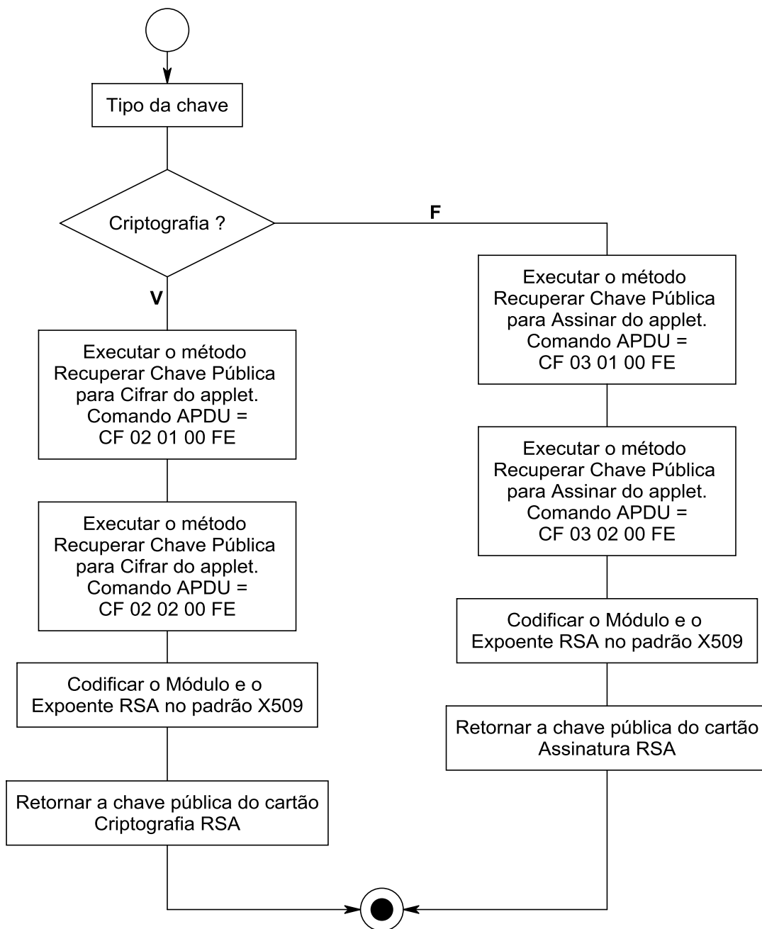
Gráfico 6-18 – Recuperação de Chaves Públicas
