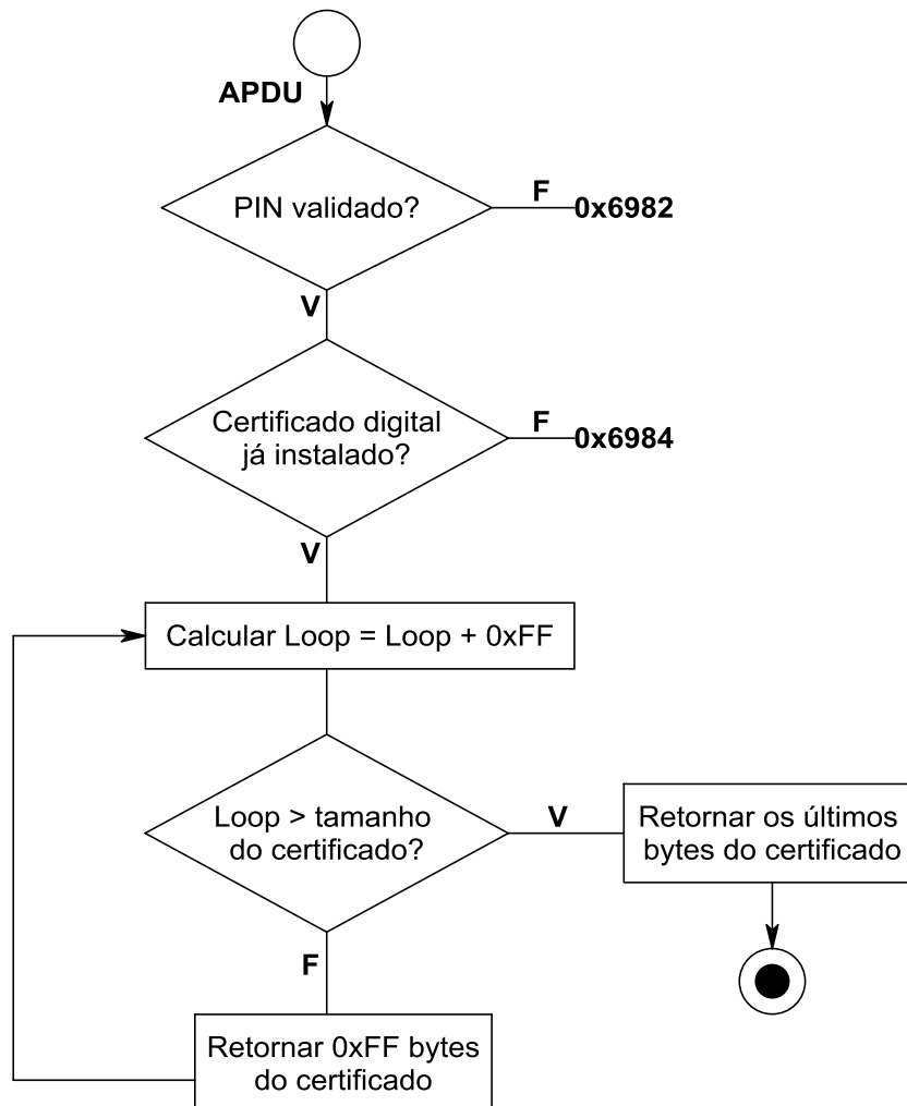
Gráfico 6-13 – Recuperar Certificado Digital
