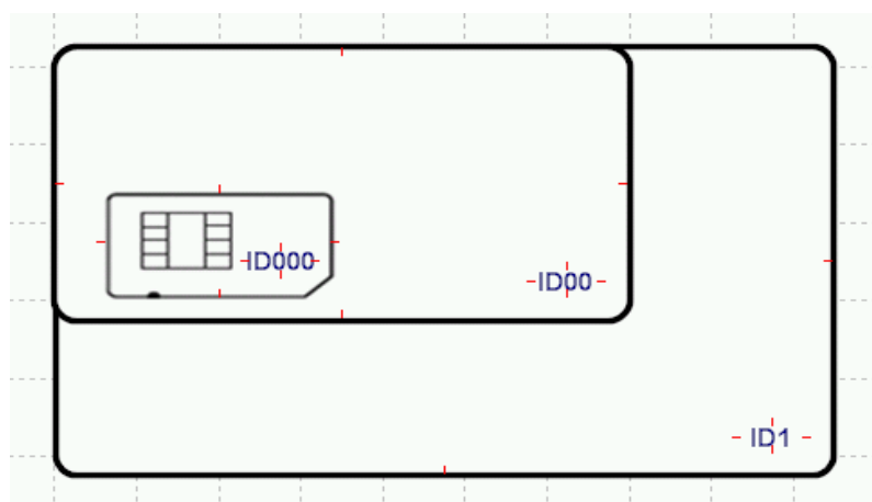
Gráfico 3-7 – Dimensões de um smart card.
