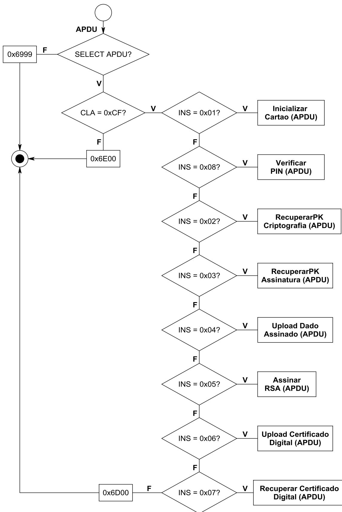
Gráfico 6-5 – Processamento do comando APDU pela JCRE de um applet
