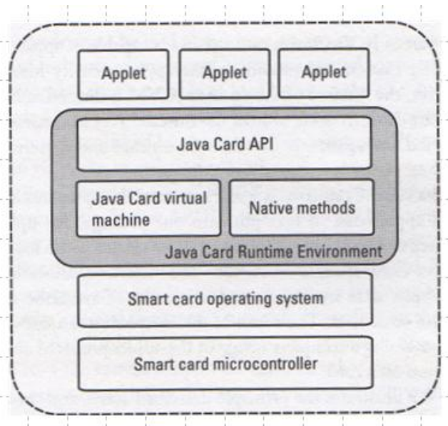
Gráfico 3-11 – Arquitetura Java Card.
