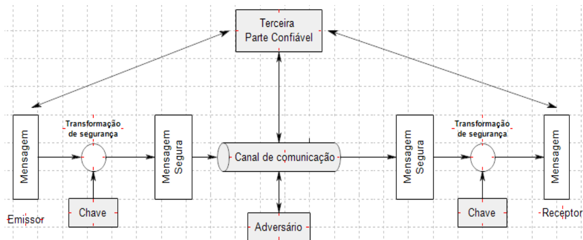
Gráfico 2-6– Representação de um modelo de segurança de comunicação.
