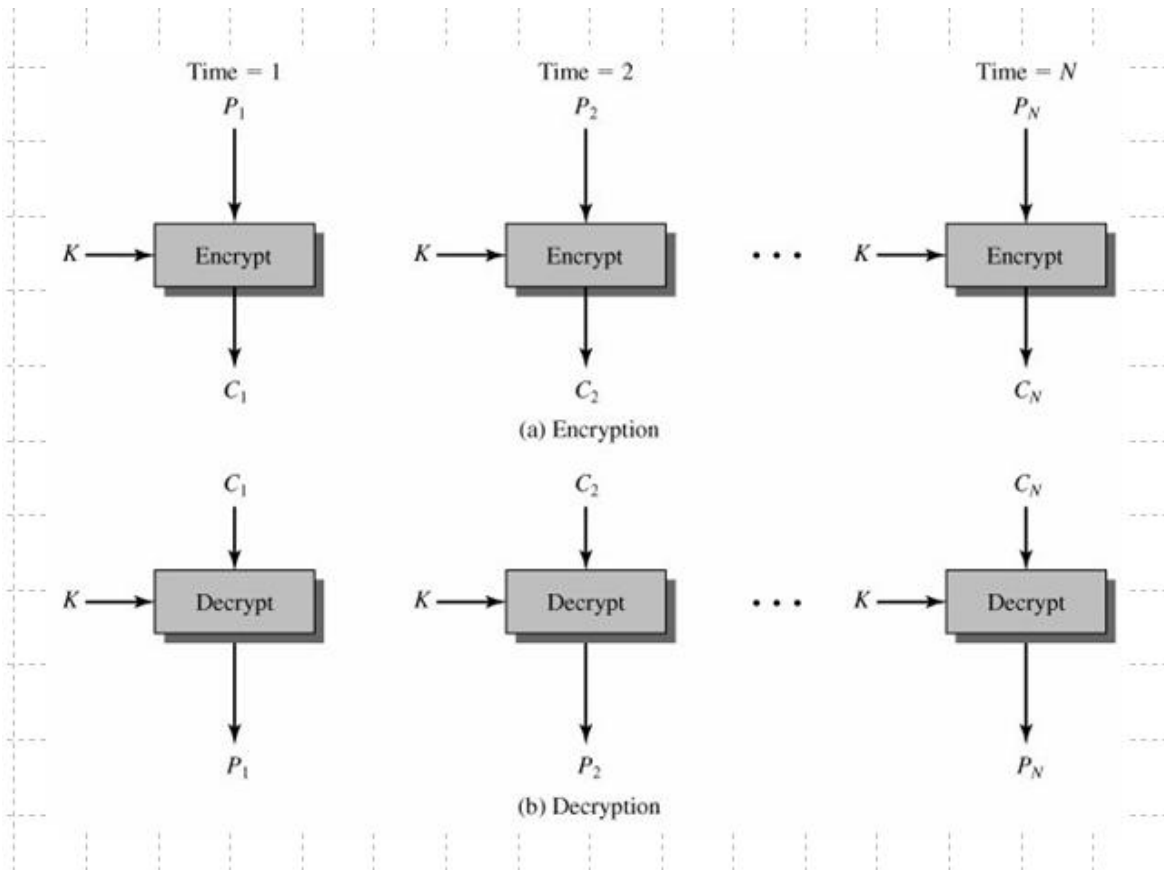
Gráfico 2-2 – Modo ECB.
