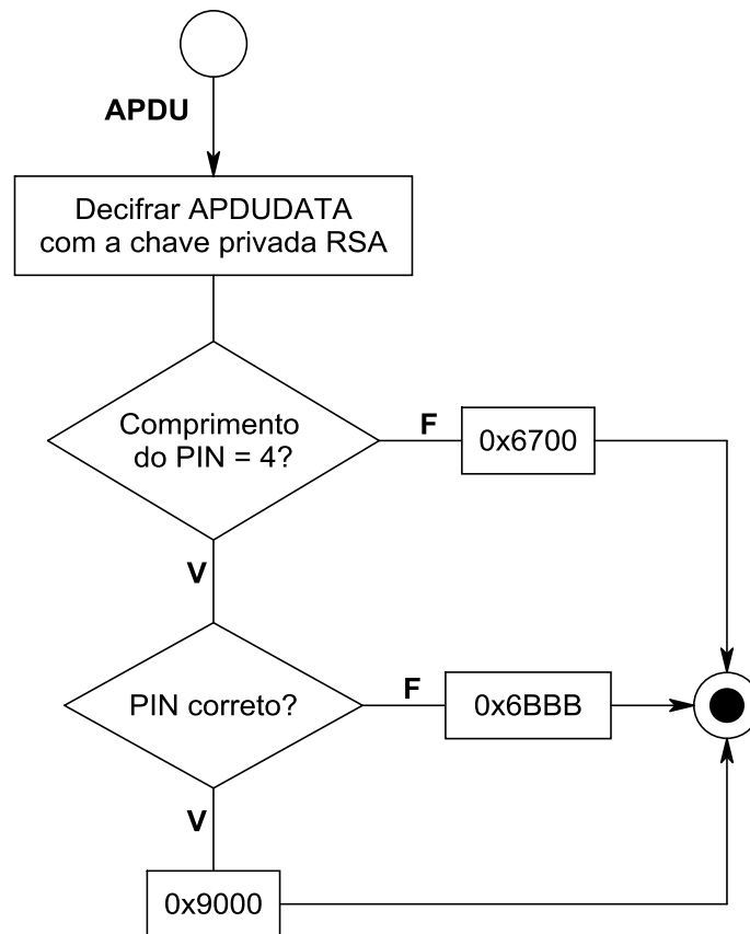
Gráfico 6-7 – Verificar PIN
