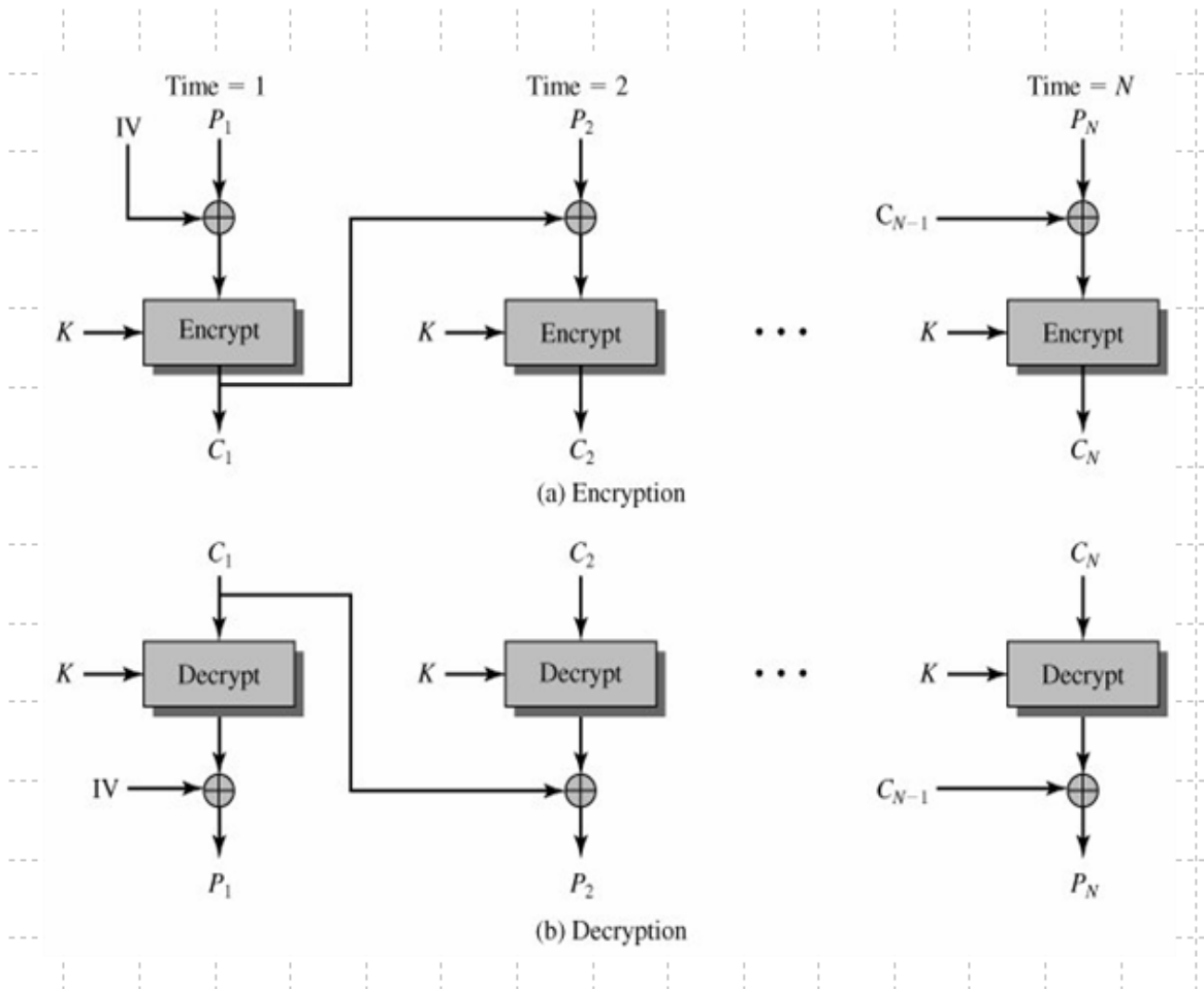
Gráfico 2-3 – Modo CBC
