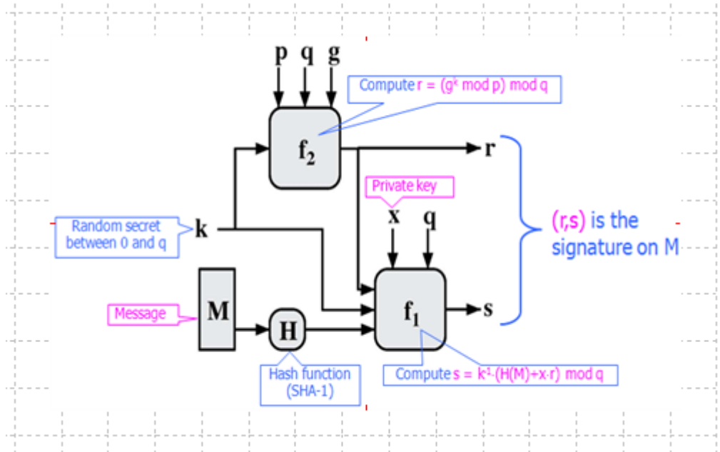
Gráfico 2-4 – Assinatura DSS.
