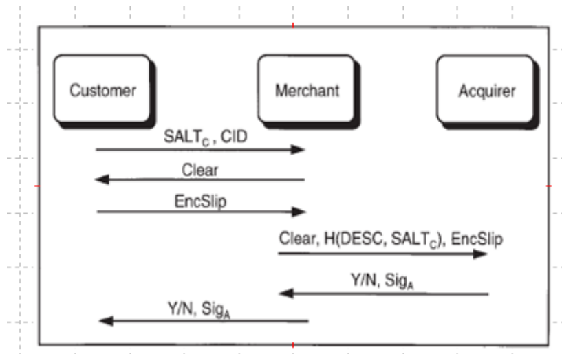
Gráfico 4-10 – Fluxo de mensagens no 1KP
