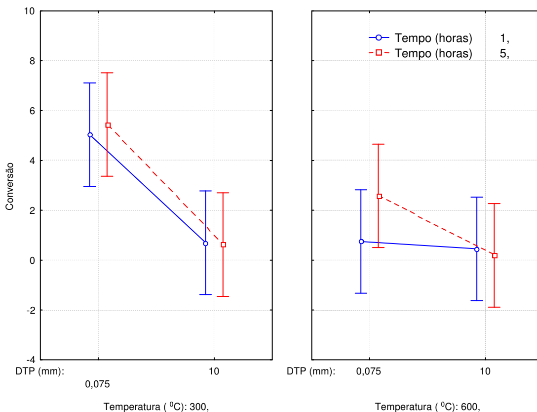
Figura 50 - Comparativo entre variáveis temperatura, tempo e tamanho de partículas.
