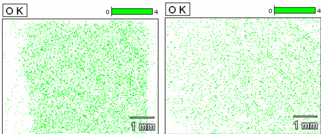
Figura 36 - EDS – tratada termicamente – Oxigênio, esquerda; EDS – In Natura – 18x – Oxigênio, direita.
