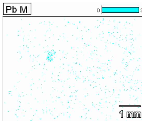
Figura 32 - EDS – Chumbo.
