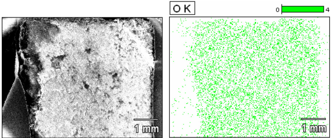
Figura 30 - MEV amostra 1 – 18x, esquerda; EDS amostra 1 – Oxigênio, direita.
