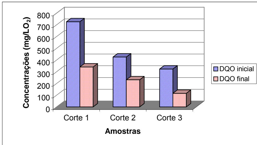
Figura 5.18– Capacidade de atenuação do solo da área de corte para DQO.
