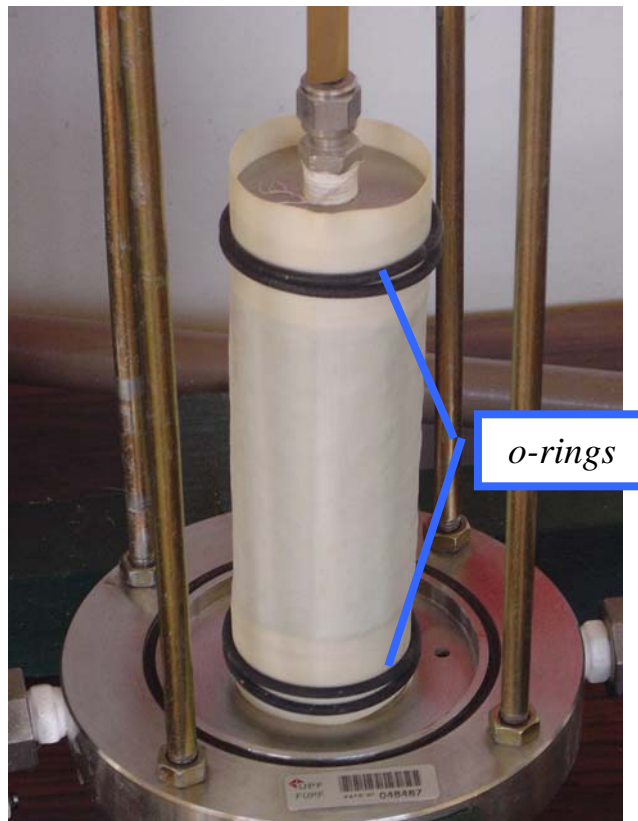
Figura 4.13 – Cilindro do solo com corpo de prova revestido com membrana de látex.
