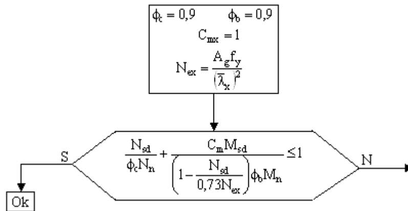
Figura 24– Fluxograma de resistência à flexocompressão
