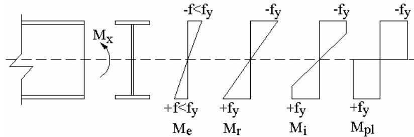
Figura 5 – Distribuição de tensões normais na flexão
