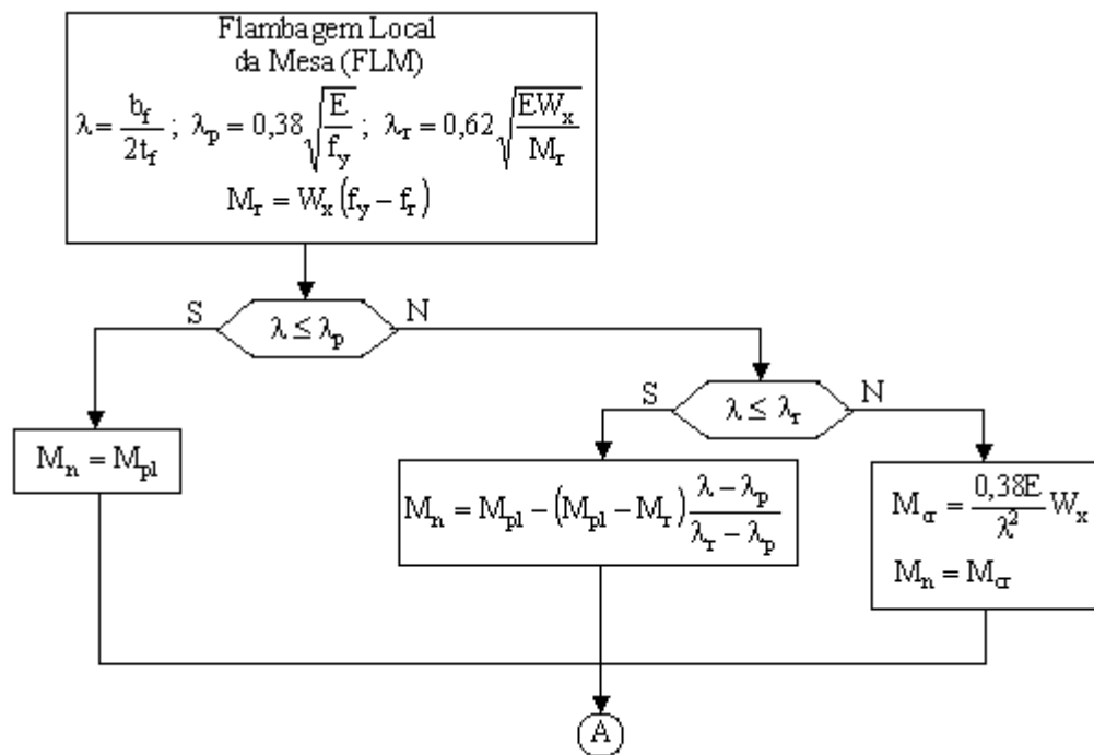
Figura 19– Fluxograma de resistência do momento fletor FLM
