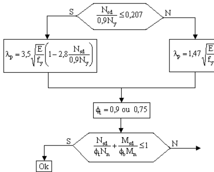
Figura 23– Fluxograma de resistência à flexotração
