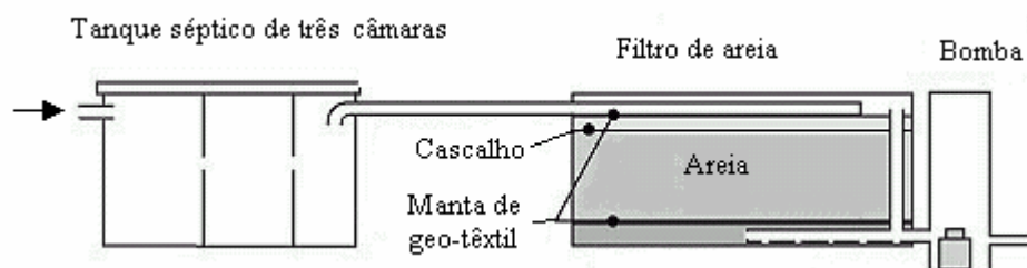
Figura 17: Esquema do tratamento da água cinza.
