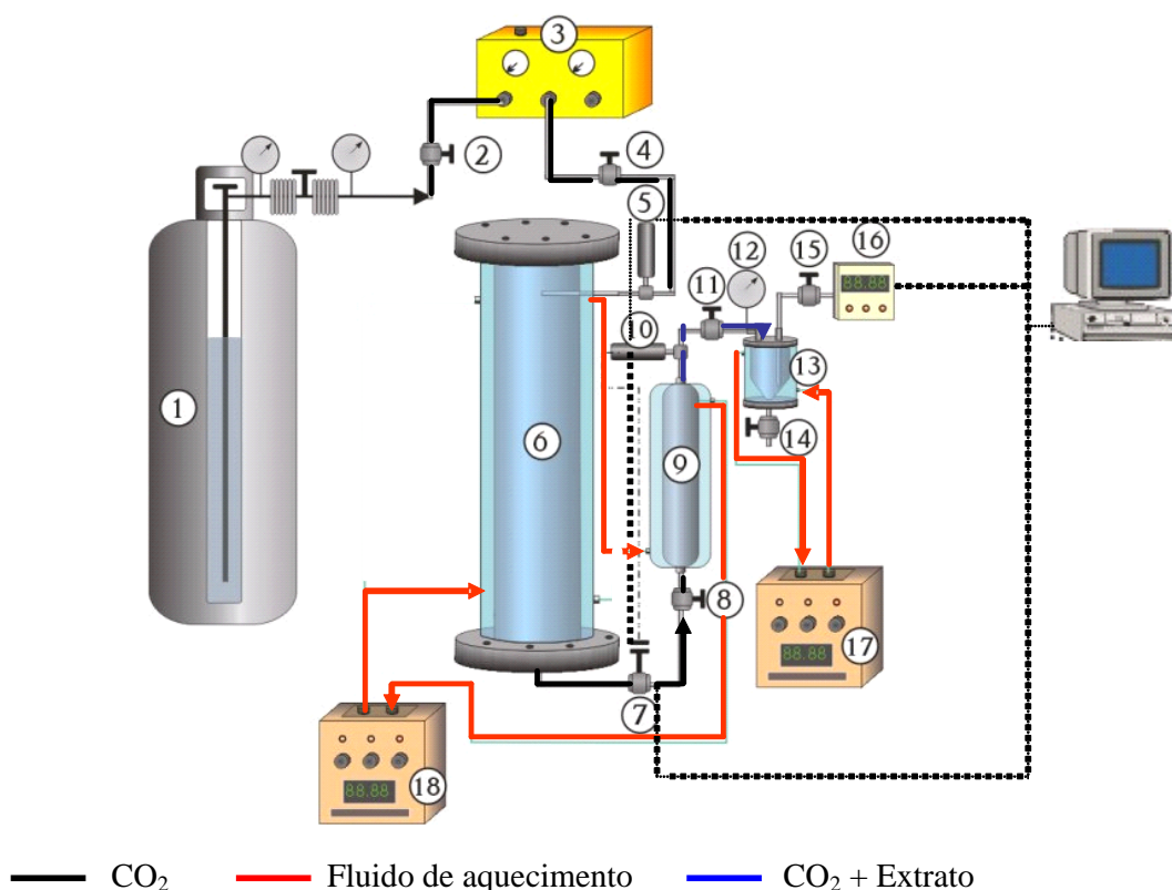
Figura 4.3. Equipamento de extração a alta pressão.
