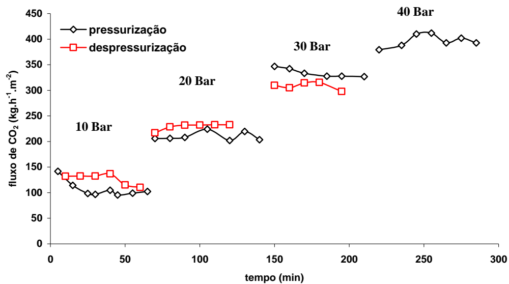
Figura 5.14. Comportamento do fluxo permeado de CO 2 SC puro em função do diferencial de pressão aplicado ao longo do tempo quando da pressurização e despressurização da membrana NF.
