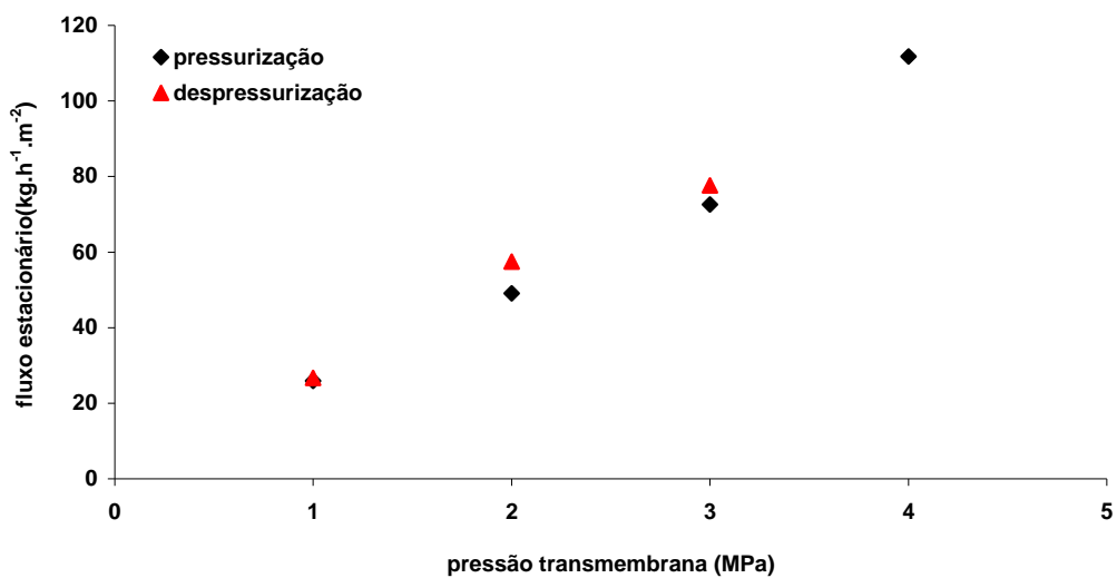
Figura 5.20. Comportamento do fluxo permeado estacionário de CO 2 SC puro em função do diferencial de pressão aplicado durante a pressurização e despressurização da membrana NF-90
