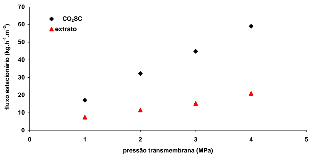
Figura 5.31. Comportamento do fluxo permeado estacionário de CO 2 SC e de extrato de cacau em função do diferencial de pressão aplicado à membrana NF.
