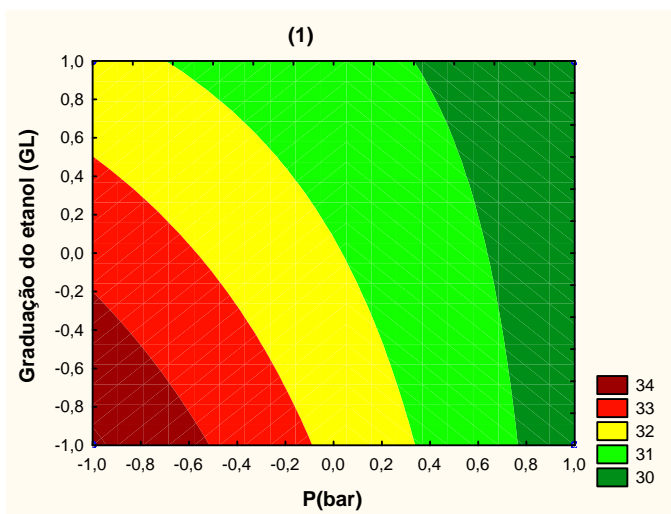
Figura 5.9. Curva de nível para a variável resposta rendimento para os fatores pressão/graduação de etanol.
