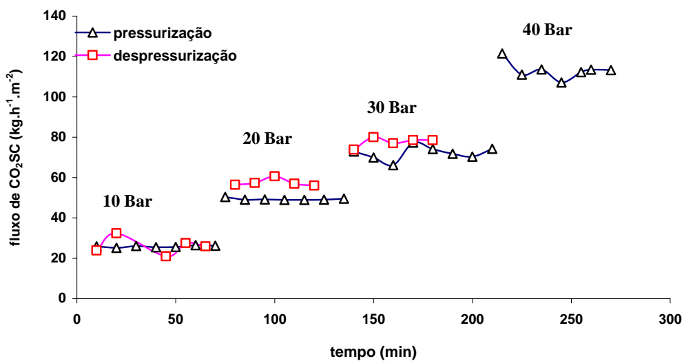
Figura 5.15. Comportamento do fluxo permeado de CO 2 SC puro em função do diferencial de pressão aplicado ao longo do tempo quando da pressurização e despressurização da membrana NF-90
