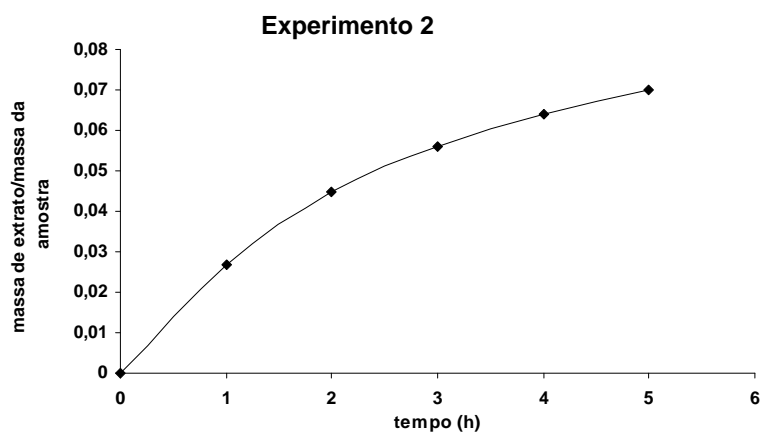
Figura 5.2. Curva de extração para obtenção do extrato de cacau utilizando CO 2 SC puro e pressão de 150 bar. (massa de cacau utilizada = 68,8g, amostra com gordura).
