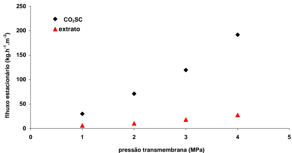
Figura 5.29. Comportamento do fluxo permeado estacionário de CO 2 SC e de extrato de cacau em função do diferencial de pressão aplicado à membrana DL.
