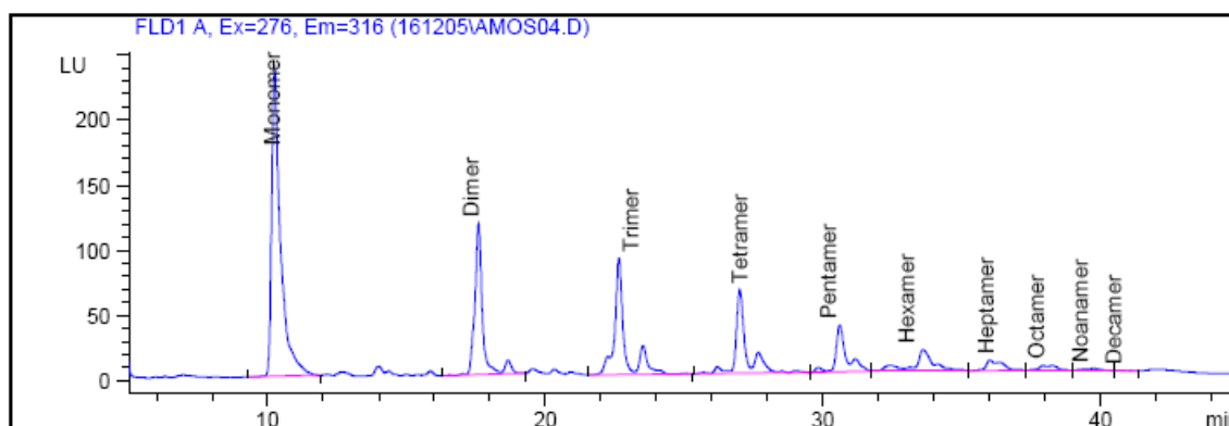
Figura 5.45. Perfil cromatográfico dos polifenóis encontrados no extrato de cacau retentado pela membrana BW-30.
