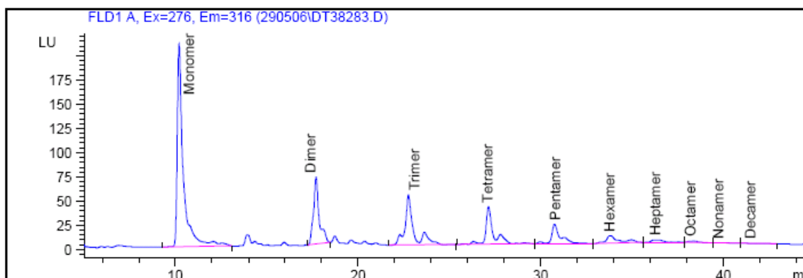
Figura 5.35. Perfil cromatográfico dos polifenóis encontrados no extrato de cacau retentado pela retentado membrana SG
