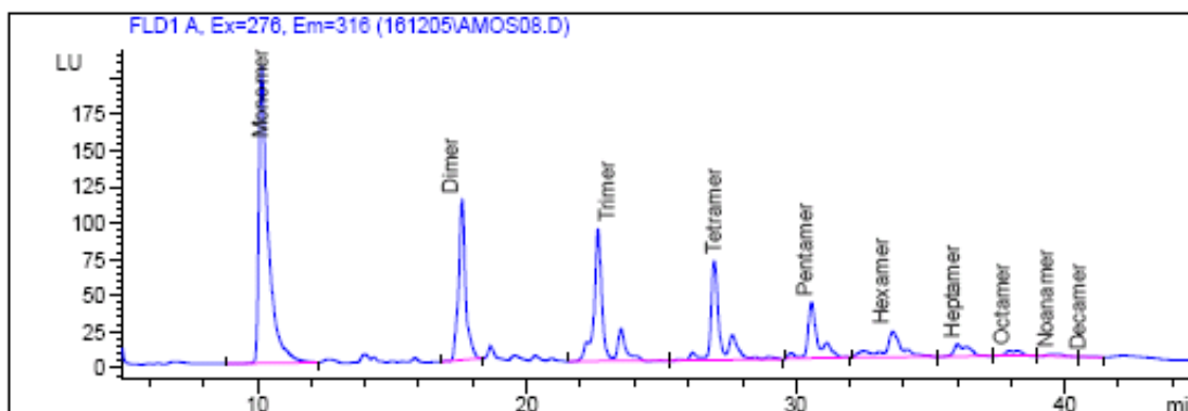
Figura 5.41. Perfil cromatográfico dos polifenóis encontrados no extrato de cacau retentado pela membrana NF
