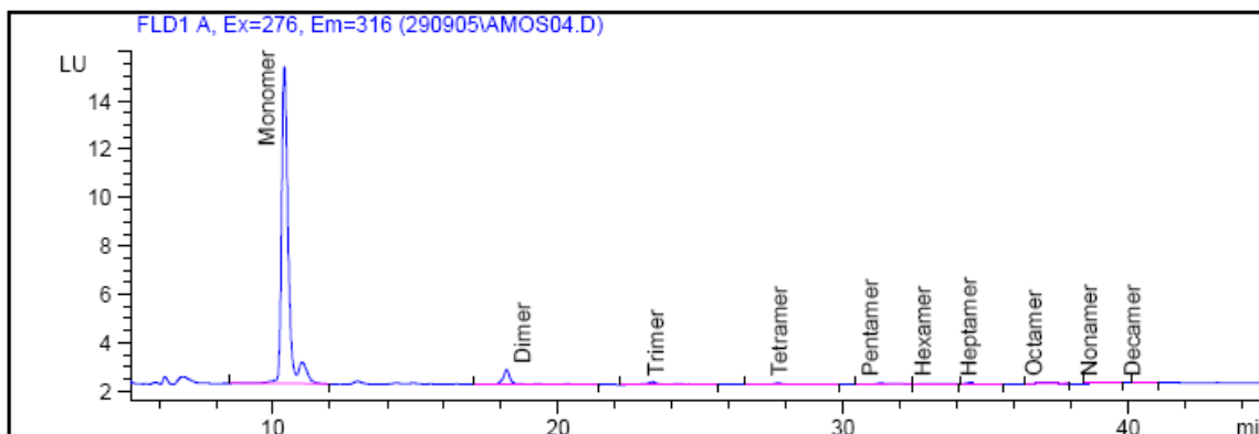
Figura 5.36 Perfil cromatográfico dos polifenóis encontrados no extrato de cacau permeado pela membrana DL
