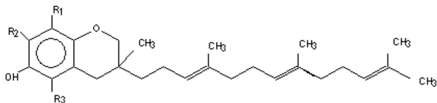
Figura 3.6. Estrutura básica dos tocotrienóis
