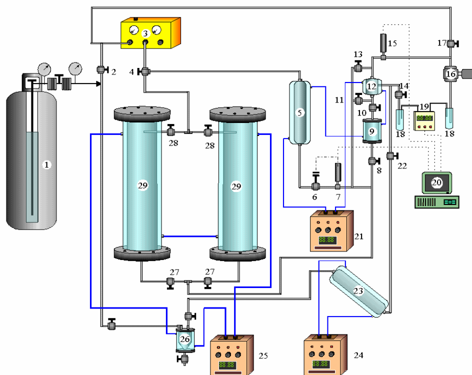
Figura 4.1. Equipamento de extração a alta pressão e separação com membranas.
