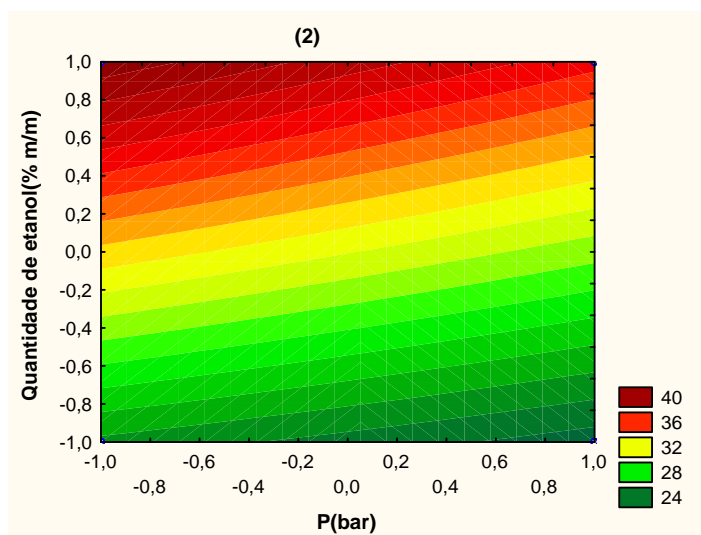
Figura 5.10. Curva de nível para a variável resposta rendimento para os fatores pressão/quantidade de etanol.
