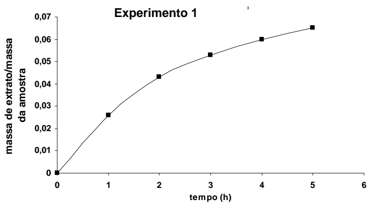
Figura 5.1. Curva de extração para obtenção do extrato de cacau utilizando CO 2 SC puro e pressão de 80 bar. (massa de cacau utilizada = 69,1g, amostra com gordura).
