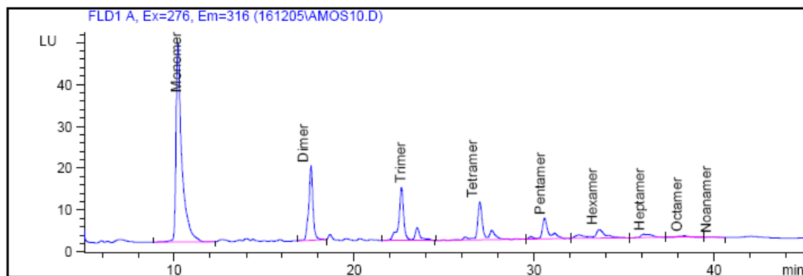
Figura 5.37. Perfil cromatográfico dos polifenóis encontrados no extrato de cacau retentado pela membrana DL
