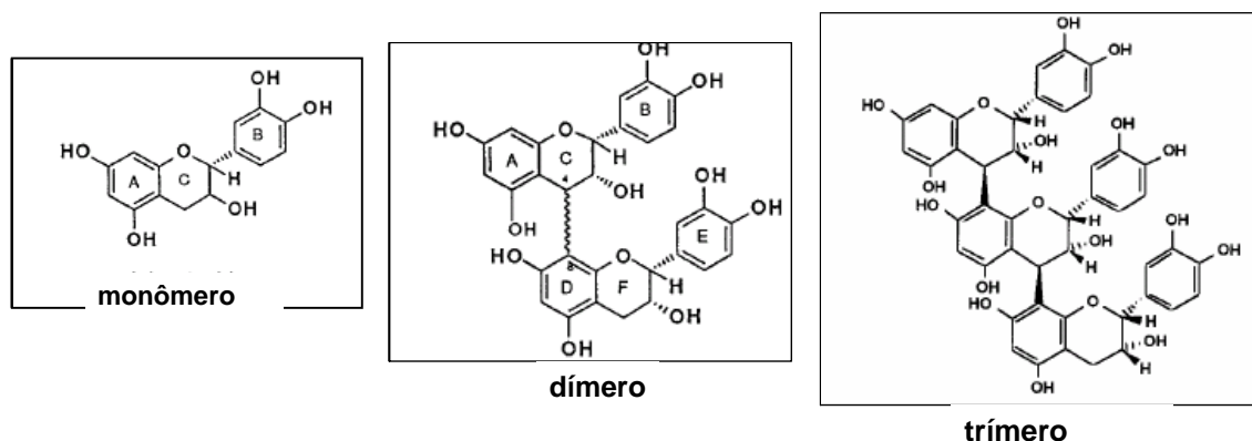
Figura 3.3. Estruturas de monômero, dímero e trímero de procianidinas.
