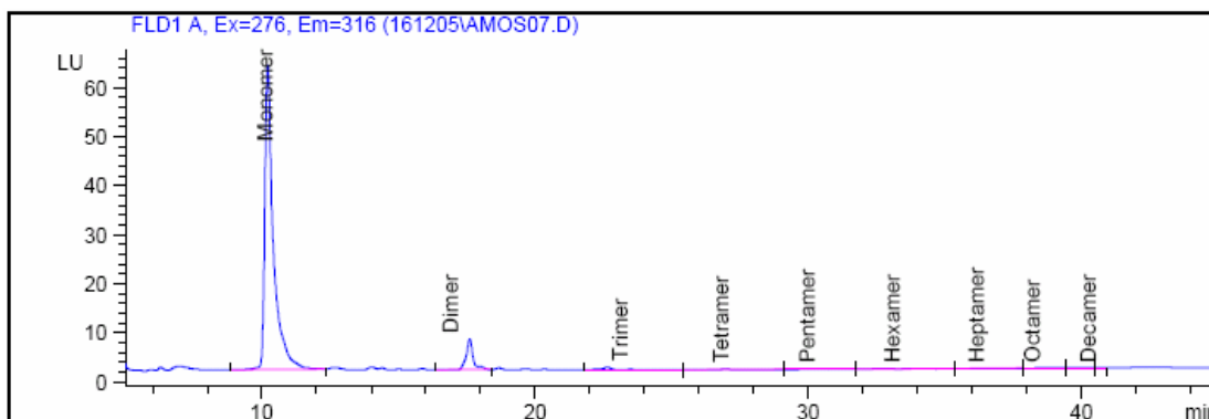
Figura 5.40. Perfil cromatográfico dos polifenóis encontrados no extrato de cacau permeado pela membrana NF.
