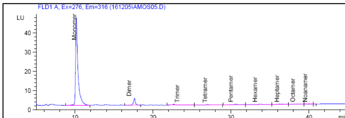
Figura 5.44. Perfil cromatográfico dos polifenóis encontrados no extrato de cacau permeado pela membrana BW-30.
