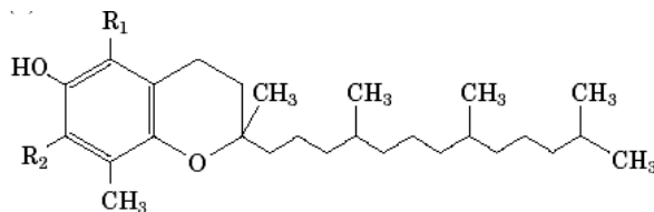
Figura 3.5. Estrutura básica dos tocoferóis
