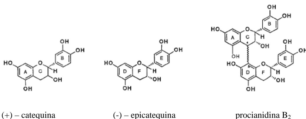
Figura 3.2. Exemplos de polifenóis encontrados em sementes de cacau
