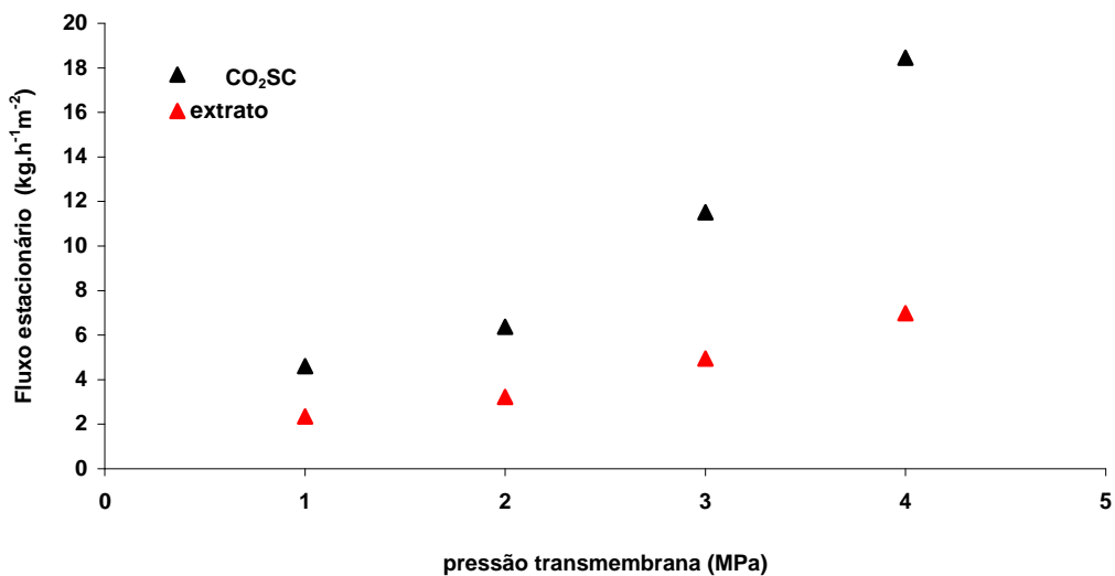
Figura 5.32. Comportamento do fluxo permeado estacionário de CO 2 SC e de extrato de cacau em função do diferencial de pressão aplicado à membrana NF-90.
