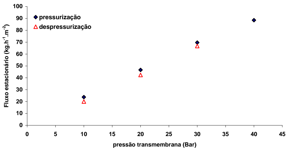
Figura 5.17. Comportamento do fluxo permeado estacionário de CO 2 SC puro em função do diferencial de pressão aplicado durante a pressurização e despressurização da membrana SG.
