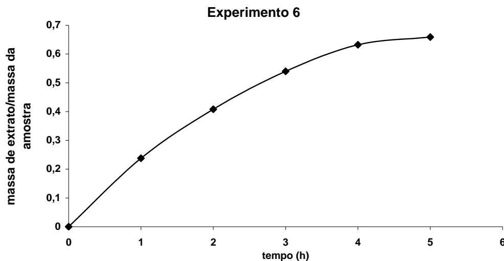
Figura 5.6. Curva de extração para obtenção do extrato de cacau utilizando CO 2 SC + 200% (V/m) de etanol 92,8GL pressão de 150 bar. (massa de cacau utilizada = 63,2g, amostra com gordura).
