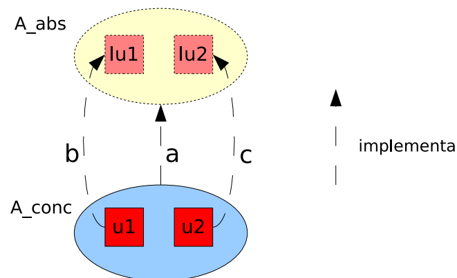
Figura 5.3: Relação entre componentes # e componente abstratos.
