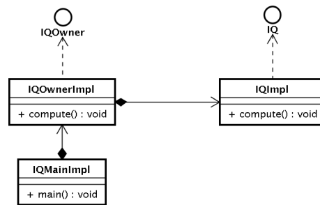
Figura 6.12: Diagrama de classes referentes a unidade q
