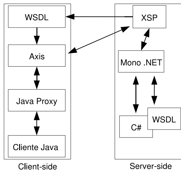
Figura 5.7: Cliente (Front-End) e servidor (Back-End) envolvidos através de Web Services
