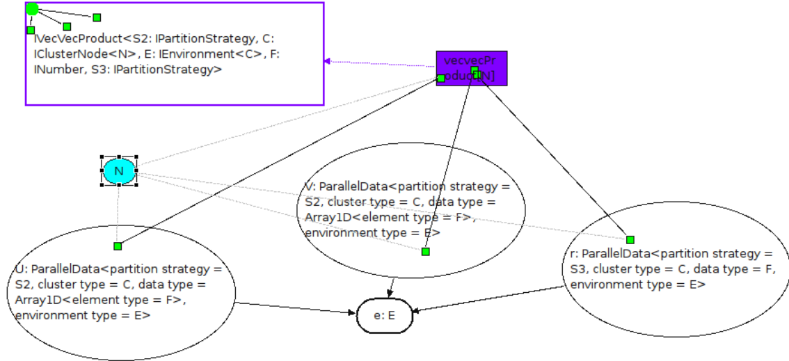
Figura 6.11: Componente para multiplicação paralela entre vetores
