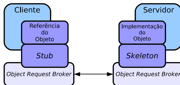
Figura 2.1: Modelo Cliente-Servidor em CORBA
