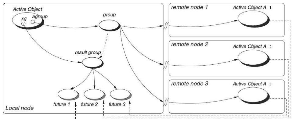
Figura 2.5: Comunicação em grupo. Fonte: [10]
