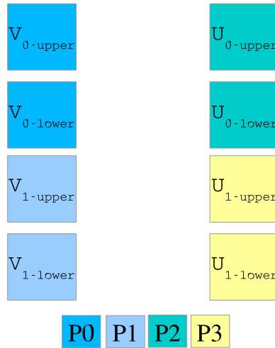
Figura 3.2: Particionamento dos vetores U e V nos respectivos processadores. A legenda indica a cor de cada processador
