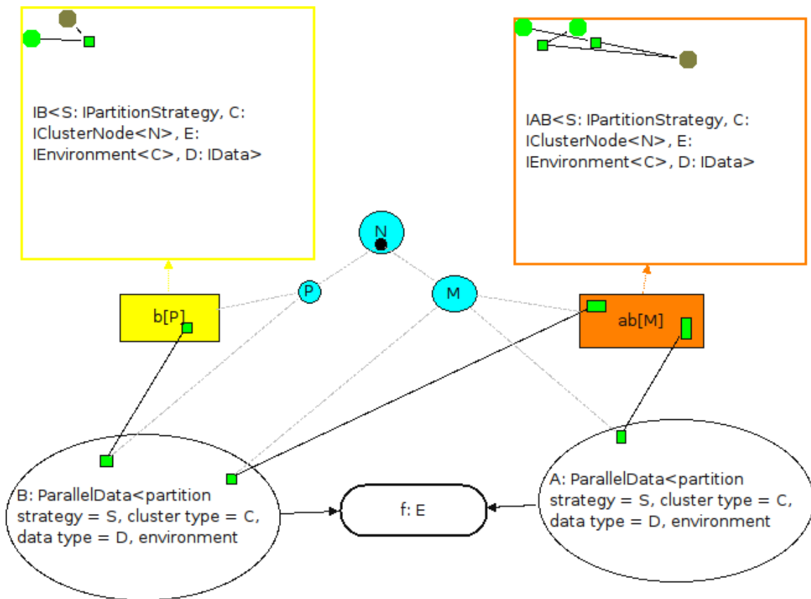
Figura 6.10: Componente para redistribuição de dados nós de uma arquitetura
