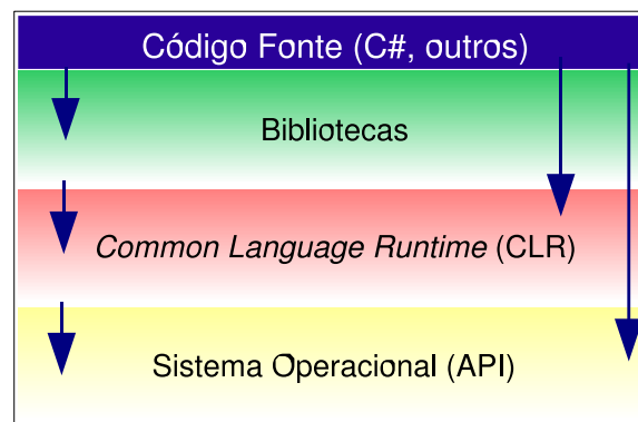
Figura 5.1: Arquitetura Mono simplificada
