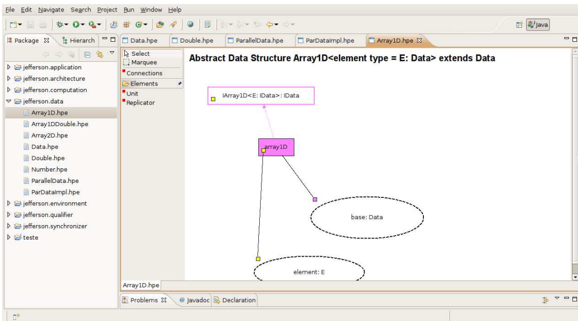
Figura 4.4: Plug-in HPE executando na plataforma Eclipse
