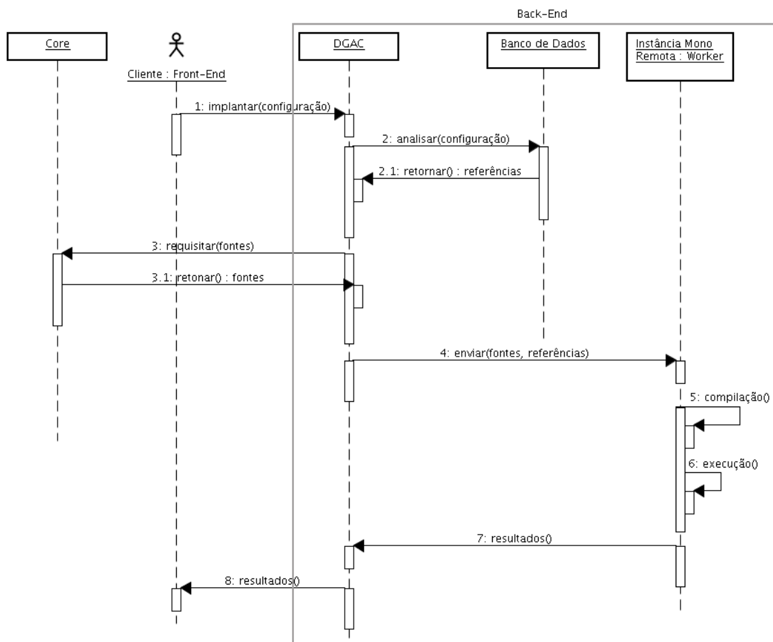
Figura 5.8: Cenário de implantação de um componente #
