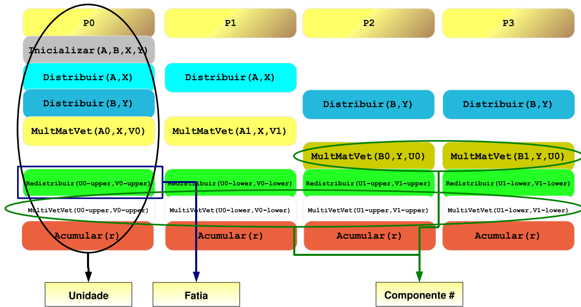
Figura 3.6: Usando ainda o exemplo da seção anterior, um componente # é formado pela união das unidades pertencentes a um interesse referente a um conjunto de processos em um programa paralelo
