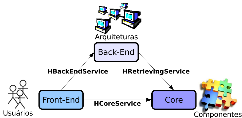
Figura 4.2: Arquitetura HPE
