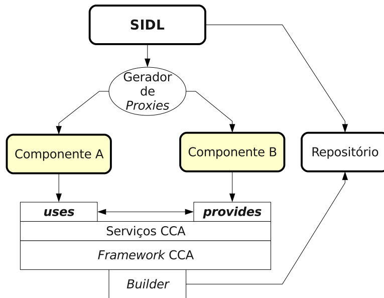
Figura 2.3: CCA
