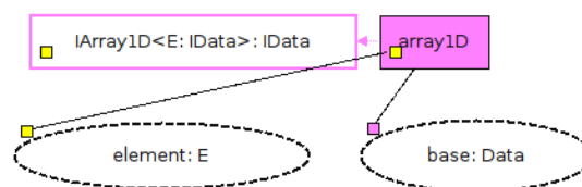
Figura 6.7: Componente Array1D
