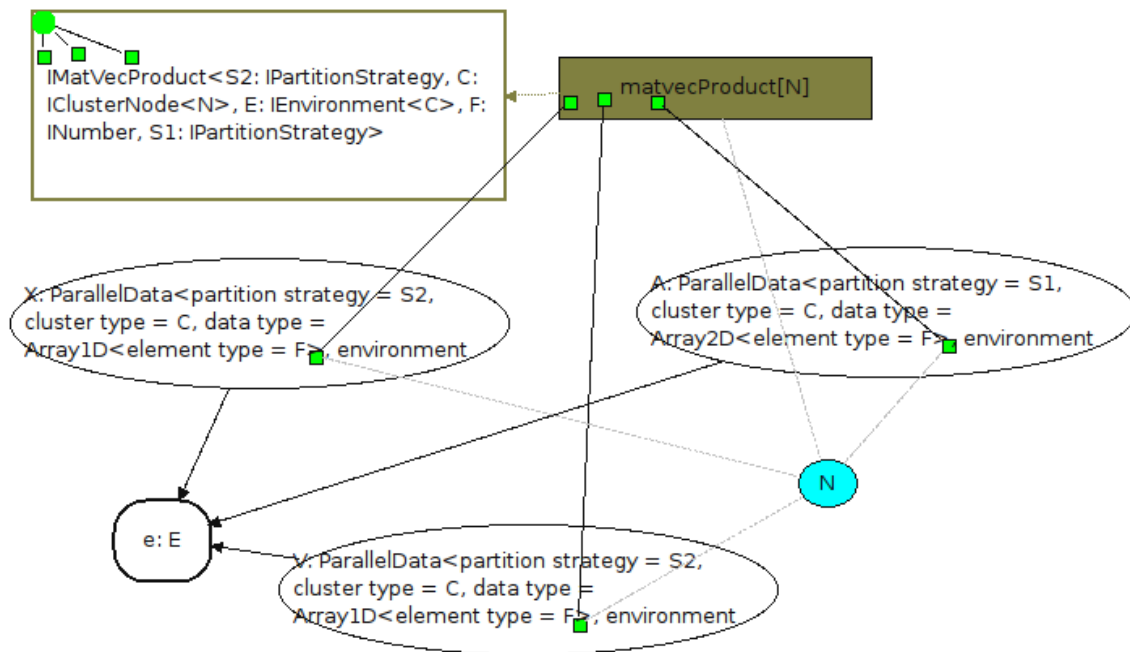
Figura 6.9: Componente para multiplicação paralela entre um Vetor e uma Matriz
