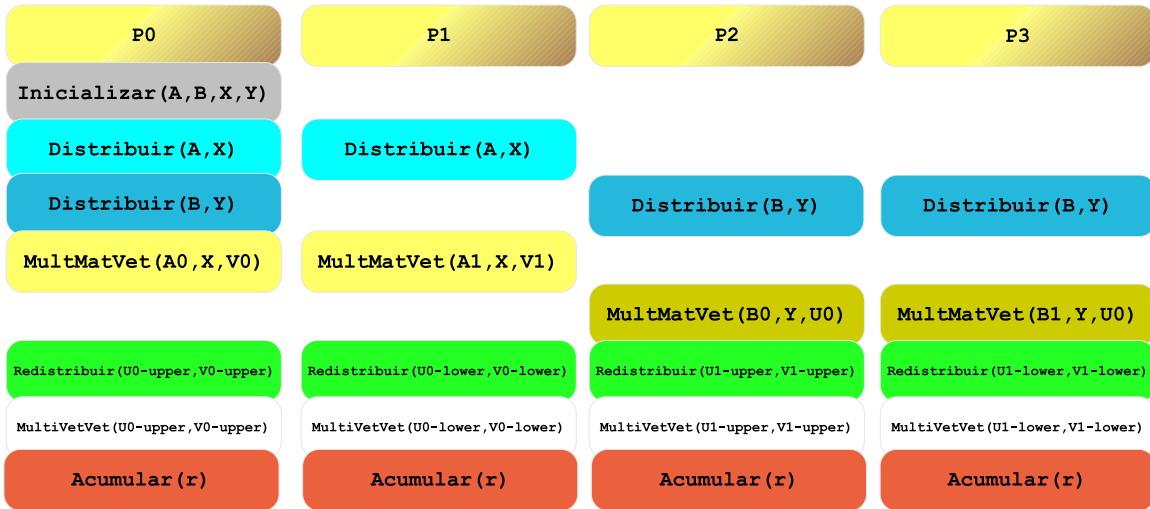
Figura 3.5: Interesses comuns e específicos discriminados por cor em cada processador
