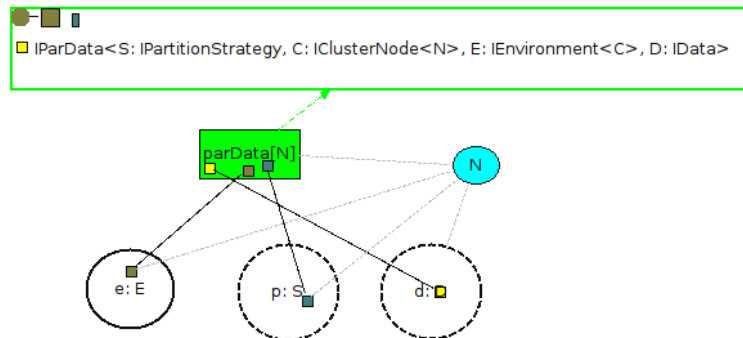
Figura 6.8: Componente Abstrato ParallelData
