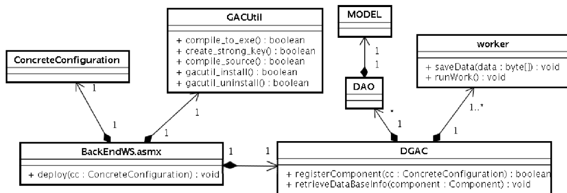
Figura 5.5: Diagrama de classes simplificado do relacionamento entre DGAC e o Web Service
