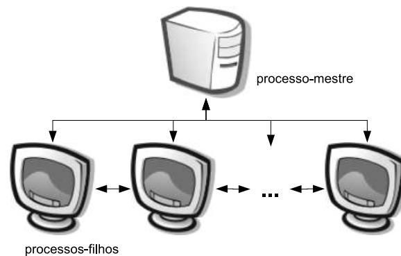
Figura 5.6: O processo-mestre comunica-se com os processos-filho através da implementação de RPC (Remote Procedure Call) em Mono . Cada um dos processos-filho troca dados entre si por meio do ambiente instalado na arquitetura do Back-End .
