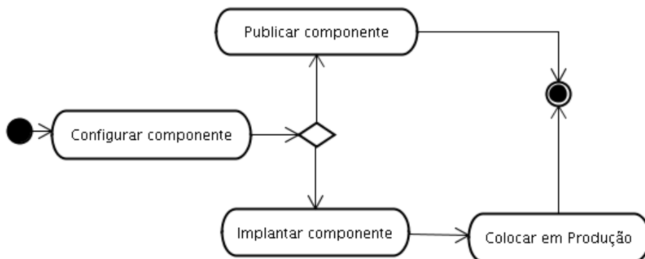
Figura 4.1: Ciclo de Vida em sistemas de programação baseados no Framework HPE
