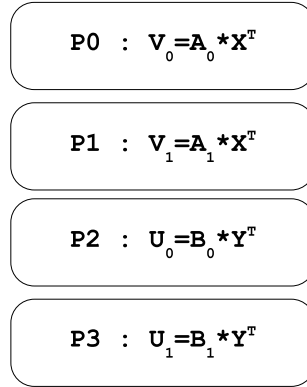
Figura 3.1: Separação da computação nos processos envolvidos
