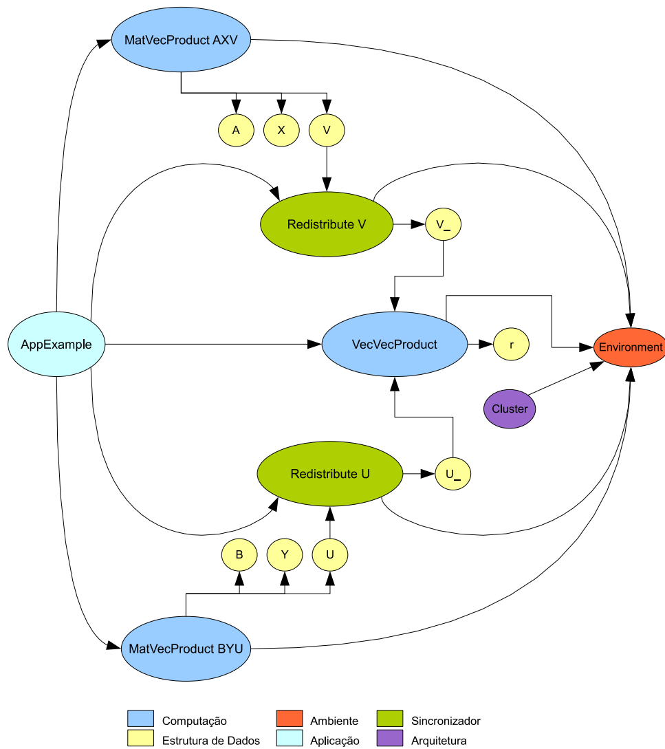
Figura 6.1: Aplicação exemplo abstrata ( AppExample ), apresentando seus componentes internos. As cores discriminam a Espécie de Componente.
