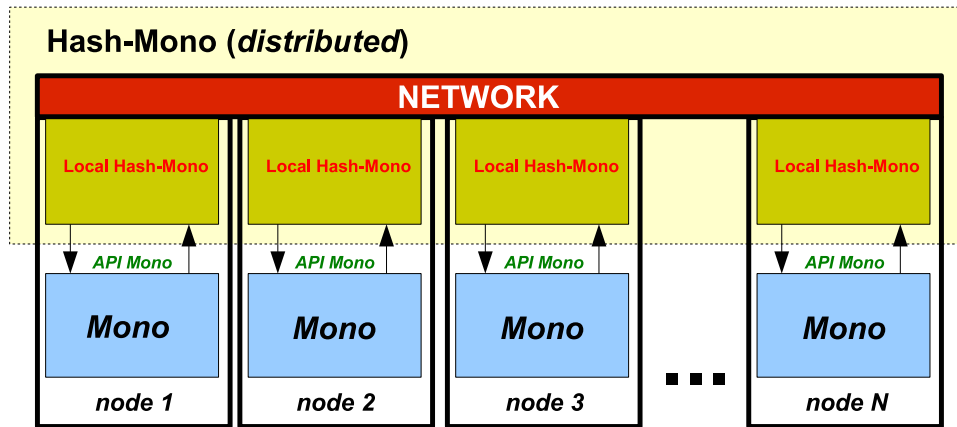
Figura 4.5: Mono embutido na arquitetura Hash
