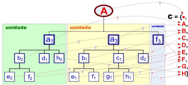
Figura 3.10: Novas unidades formadas a partir da sobreposição de fatias dos componentes internos à A
