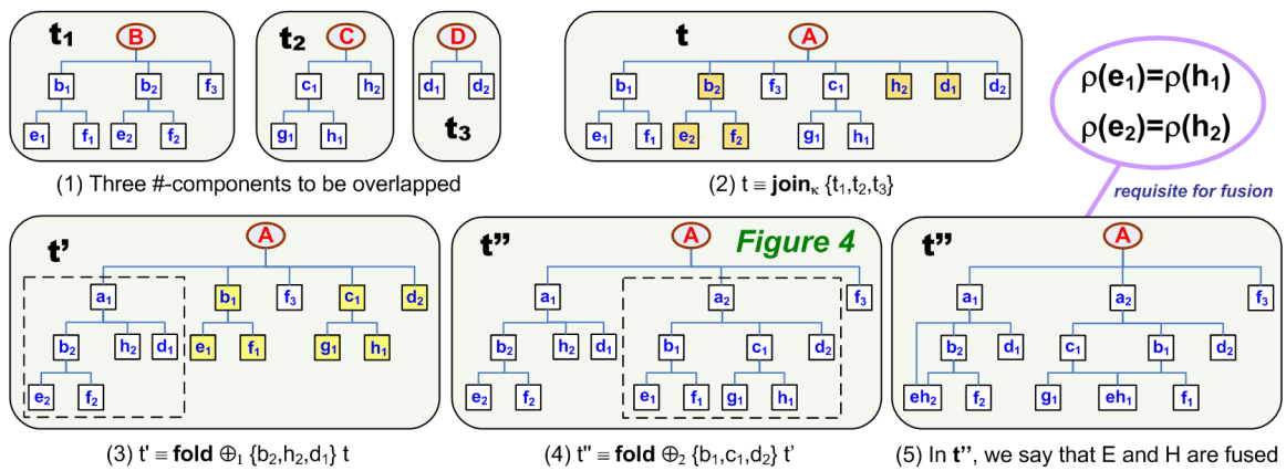
Figura 3.11: Operações fundamentais de sobreposição sobre componentes internos à A
