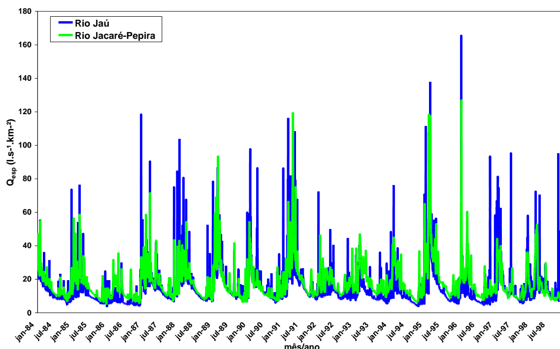
Figura 24: Vazões específicas ( l \cdot s^{-1} \cdot km^{-2} de bacia) Rios Jaú e Jacaré-Pepira de 1984 a 1998.
