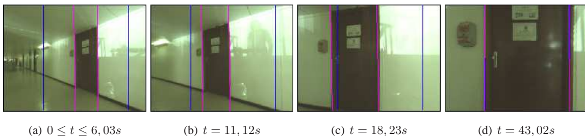
Figura 4.17: Seqüência de imagens da câmara esquerda durante o experimento de estimação e controle PBVS simultâneos partindo da posição 2 descrita na Figura D..2. As linhas em magenta são as projeções da estimativa e as linhas azuis são a projeção da referência de controle.
