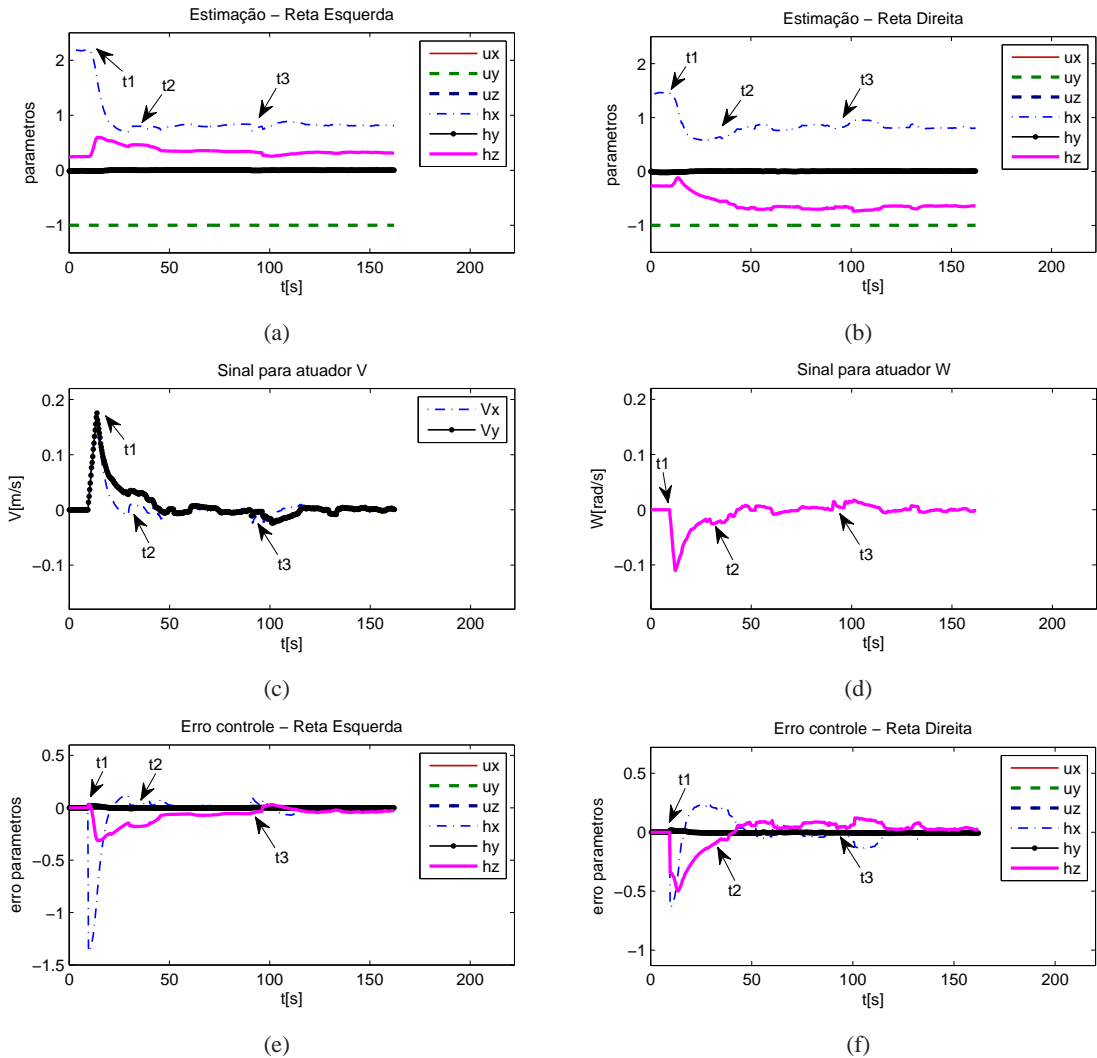
Figura 4.20: Resultados do experimento de estimação e controle PBVS simultâneos partindo da posição 3 descrita na Figura D..2. (a) e (b) Estimação dos parâmetros da reta esquerda e direita, respectivamente. (c) Velocidades de translação enviadas ao atuador. (d) Velocidade de rotação enviada ao atuador. (e) e (f) Erro de controle referente aos parâmetros 3D da reta esquerda e direita, respectivamente. t_1 = 9,61 corresponde ao instante de início da ação de controle. t_2 = 33,12 corresponde ao instante em que o tracking perdeu a reta direita. t_3 = 91,03 corresponde ao instante em que a reta direita volta a ser rastreada.
