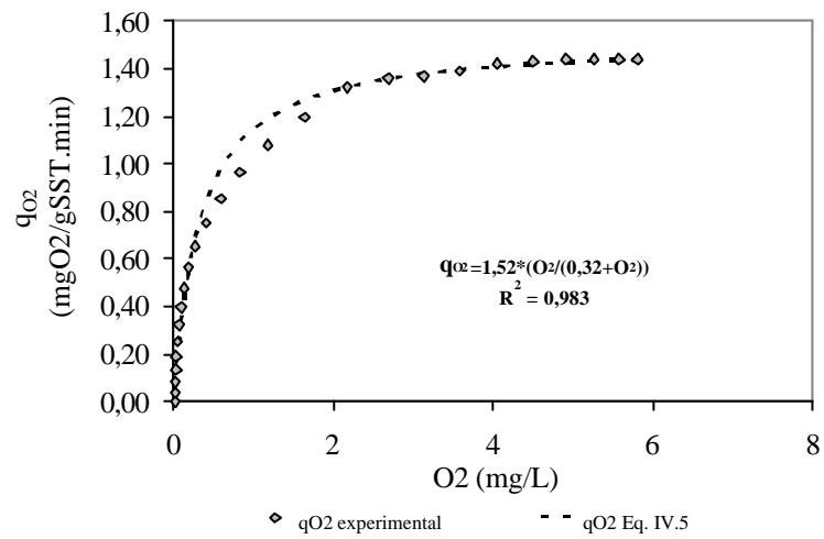
Figura 2.4.: Ajuste da Eq. IV.5 aos pontos experimentais de velocidade específica de consumo de oxigênio – Condição IV.
