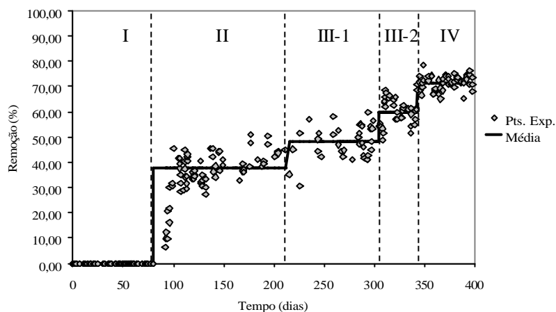
Figura V. 11: Remoção de nitrogênio durante a operação do reator SBR
