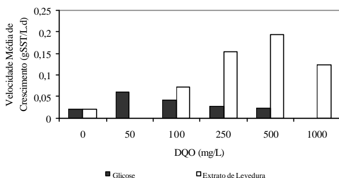
Figura V. 4: Influência da concentração de DQO na velocidade média de crescimento de T. denitrificans (media nas primeiras 24 horas)
