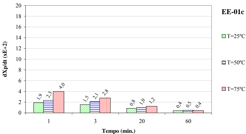
Figura 5.23 – Efeito da temperatura da solução sobre a cinética da velocidade de conversão do calcário EE-01c, para os tempos de 1, 3, 20 e 60 minutos.
