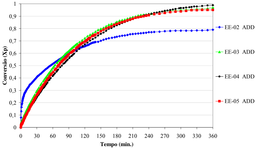
Figura 5.13 – Efeito da composição química dos calcários EE-02 até EE-05 sobre a cinética de conversão, para T = 50^{\circ}\text{C} , \text{pH} = 5,0 , 0,1\text{M CaCl}_2 , Q_{\text{CO}_2} = 315\text{cm}^3/\text{min} borbulhado.
