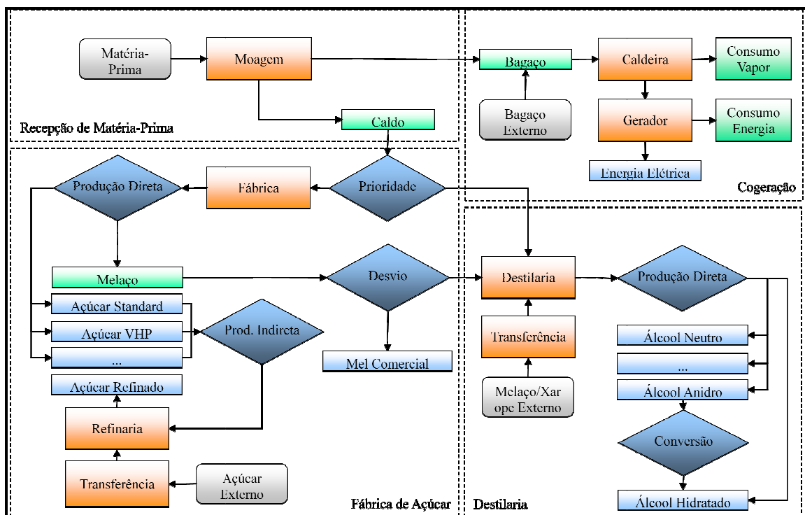
Figura 14. Fluxograma do processo de produção de açúcar, álcool e energia elétrica
