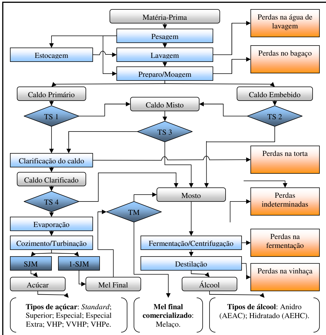
Figura 15. Fluxograma do processo de produção de açúcar, álcool e melaço
