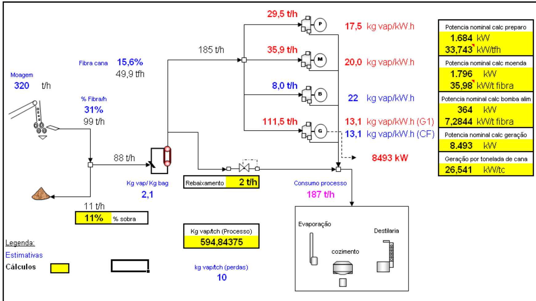
Figura 40. Exemplo de cálculo do balanço de vapor e energia da USC
