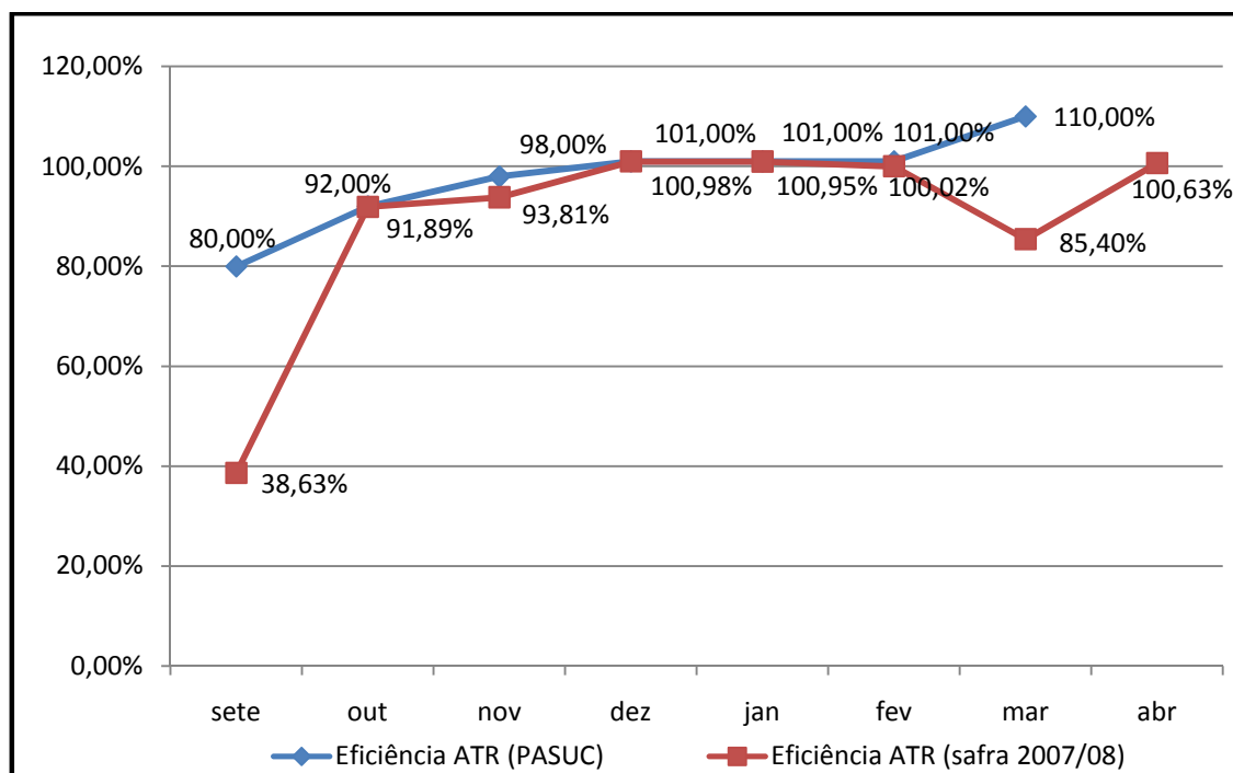
Figura 23. Comparativo da eficiência global em ATR utilizada no modelo PASUC e valores reais ( E_{atr}^{USC^t} )
