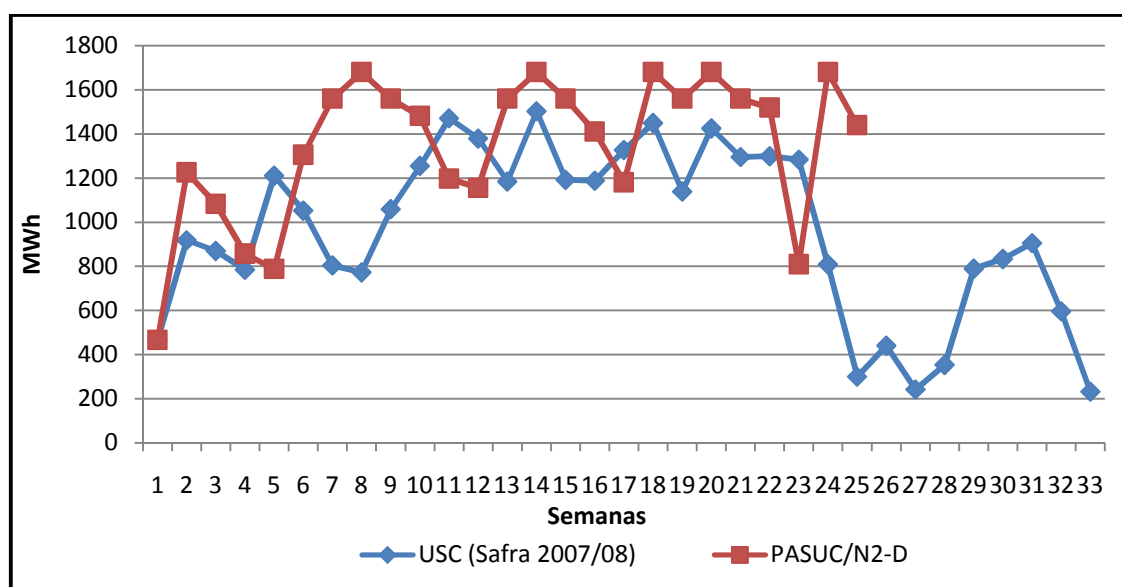
Figura 19. Geração de energia planejada pelo modelo PASUC/N2 e a dados da safra 2007/2008
