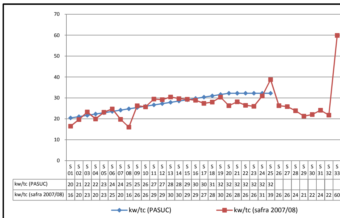
Figura 18. Comparativo de geração de energia por tonelada de cana – PASUC/N2
