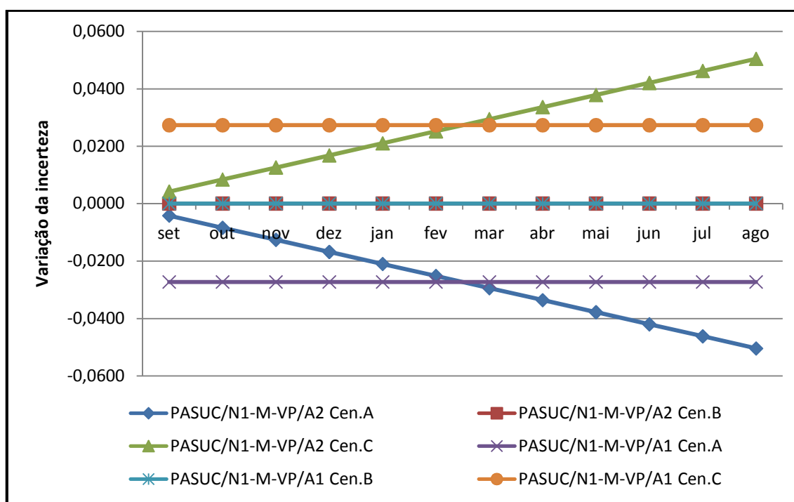
Figura 27. Percentual de incerteza em cada abordagem/cenário do modelo PASUC/N1-M-VP
