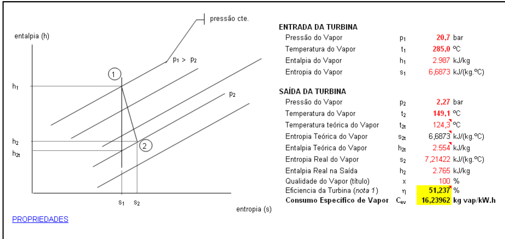
Figura 41. Exemplo de cálculo de rendimento e consumo de vapor de uma turbina
