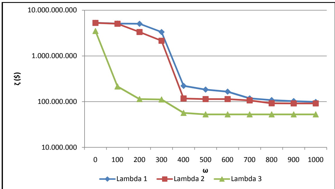
Figura 29. Impacto dos parâmetros de robustez e variabilidade entre cenários na margem de contribuição provável do modelo PASUC/N1-M-VP/A2
