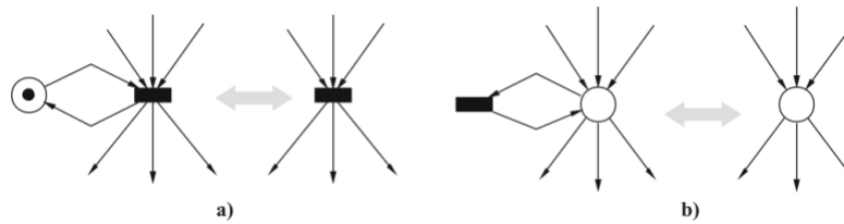
Eliminação de lugares auto-iterativos (a) e Eliminação de transições auto-iterativas (b).
