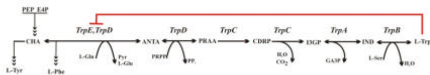
Figura 7. Inibição retroativa da enzima antranilato sintase, TrpE, pelo produto final da via, o triptofano.
