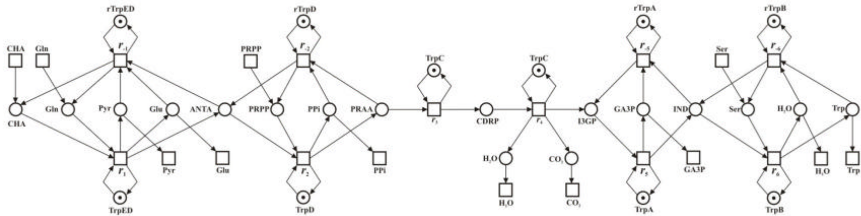
Figura 66. Modelo ilimitado da via de biossíntese do triptofano em termos de redes de Petri. A concentração das enzimas é considerada constante. Entradas e saídas obedecem a um fluxo infinito. Principais abreviações: ANTA, antranilato; CDRP, 1-( o -carboxifenilamino)-1-deoxiribulose 5-fosfato; CHA, corismato; GA3P, gliceraldeído 3-fosfato; I3GP, indol 3-glicerol-fosfato; IND, indol; Gln, glutamina; Glu, glutamato; Trp, triptofano; PPA, pafenato; PPI, fenilpiruvato; PRAA, fosforibosil antranilato; PRPP, 5-fosforibosil- a -pirofosfato; Pyr, piruvato; TrpA, TrpB, TrpC, TrpD e TrpE, conjunto de enzimas expressas pelo operon trpEDCBA .
