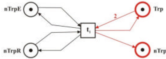
Figura 64. Regulação do triptofano no nível basal médio.
