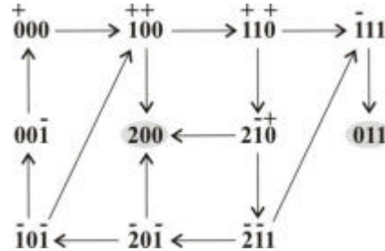
Figura 37. Grafo de transição assíncrona para o grafo de regulação da Figura 35.
