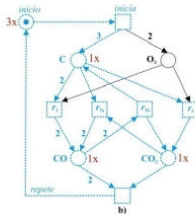
Figura 31. Circuito correspondente a invariante de lugar \mathbf{y}_1 = \{3inicio, C, CO, CO_2\} .
