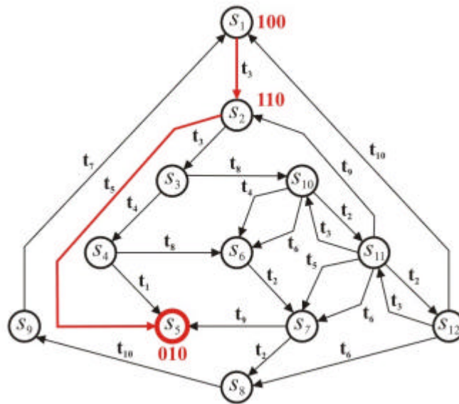
Figura 65. Grafo de alcançabilidade para o triptofano basal no nível médio.
