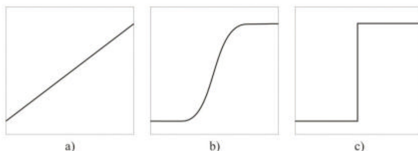
Figura 32. Idealização linear (a); Comportamento sigmoidal relacionando a concentração do regulador e seu efeito (b); Idealização lógica, a qual é infinitamente não linear.
