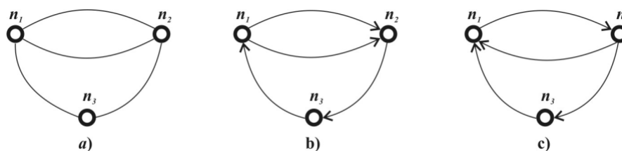
Figura 9. Multiplicidade : Multiplicidade entre os nodos n_1 e n_2 caracterizando um multigrafo não orientado (a); Multiplicidade entre os nodos n_1 e n_2 em um multigrafo orientado (b); Não caracteriza um multigrafo, pois as arestas paralelas entre os nodos n_1 e n_2 possuem orientação diferentes (c).
