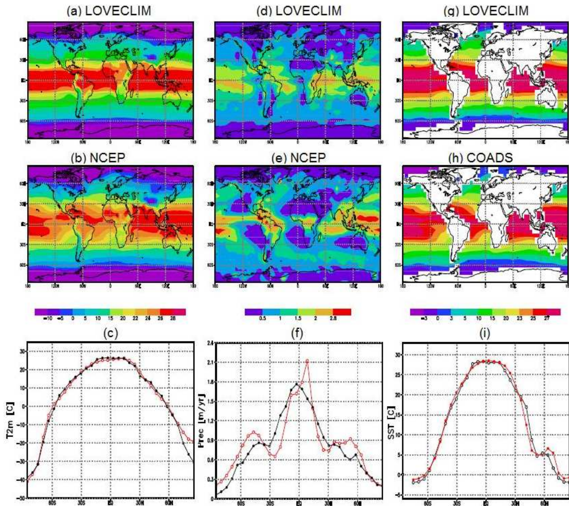
Figura 4: Temperatura média anual do ar a 2m (°C). a) simulada pelo LOVECLIM, b) reanálise do NCEP e c) linha preta: média zonal do LOVECLIM, linha vermelha: média zonal pela reanálise do NCEP, d), e) e f) o mesmo que a, b, c, mas para a precipitação e g), h), i) para a TSM.
