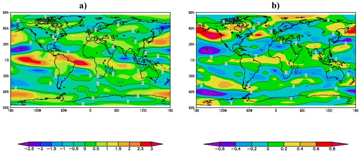
Figura 13: a) Anomalia nos Ventos com experimento acoplado, entre um cenário com 700ppm de CO 2 e CTR. b) Anomalia nos Ventos com experimento desacoplado, entre um cenário com 700ppm de CO 2 e CTR
