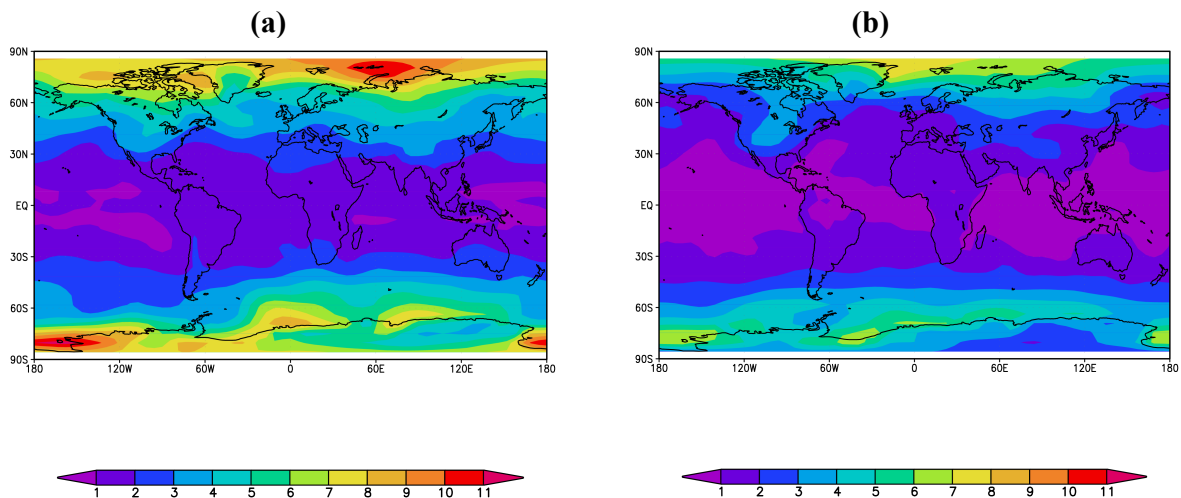
Figura 9: (a) Anomalia da temperatura a 2m no experimento acoplado, entre simulação com 700ppm de CO 2 e CTR. (b) Anomalia da temperatura a 2m no experimento desacoplado, entre simulação com 700ppm de CO 2 e CTR
