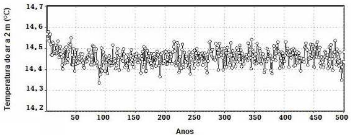
Figura 3: Média Global do ar a 2m na simulação de controle (°C).
